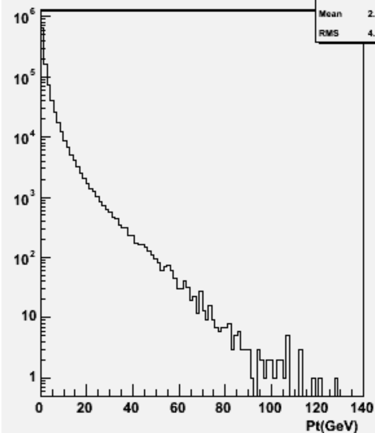
Particle Pt : w102441 cce3e3bb_o
