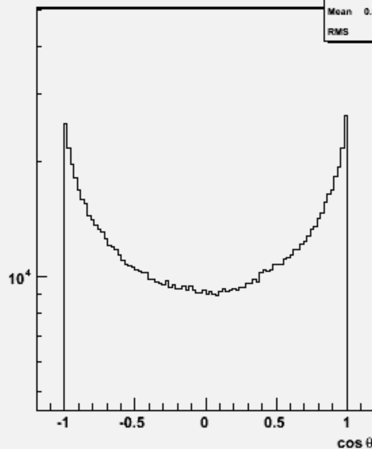
Particle cos \theta : w102441 cce3e3bb_o
