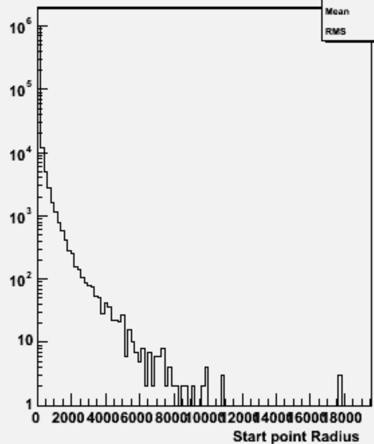
Start point R : w102441 cce3e3bb_o
