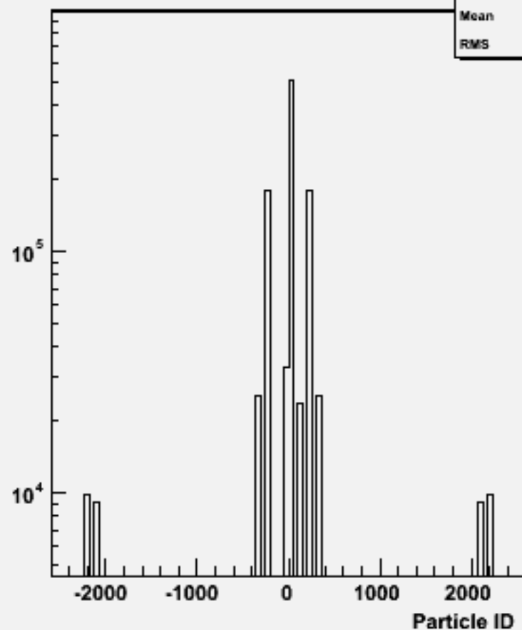
Particle ID : w102441 cce3e3bb_o
