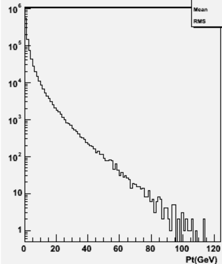
Particle Pt : w102436 cce3e3dd_o
