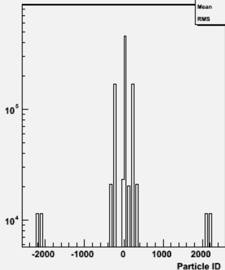
Particle ID : w102436 cce3e3dd_o
