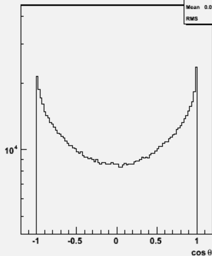
Particle cos \theta : w102436 cce3e3dd_o
