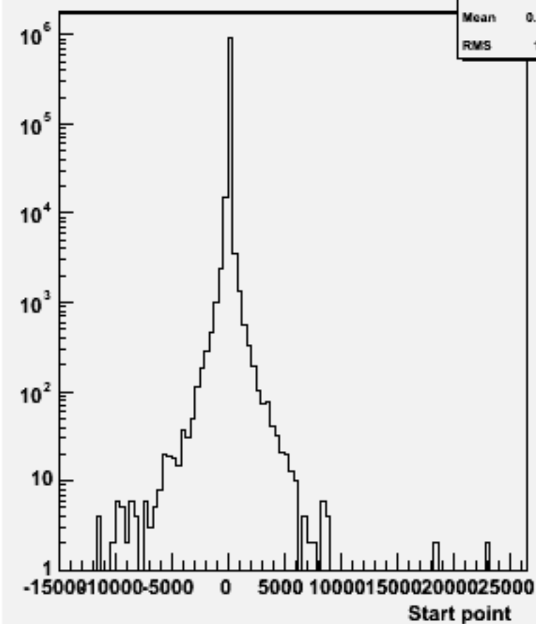
Start point Z : w102436 cce3e3dd_o
