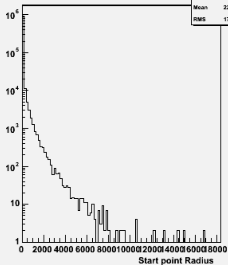
Start point R : w102436 cce3e3dd_o
