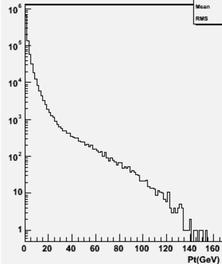
Particle Pt : w102429 cce2e2bb_o
