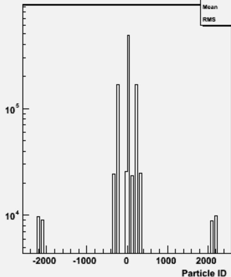
Particle ID : w102429 cce2e2bb_o
