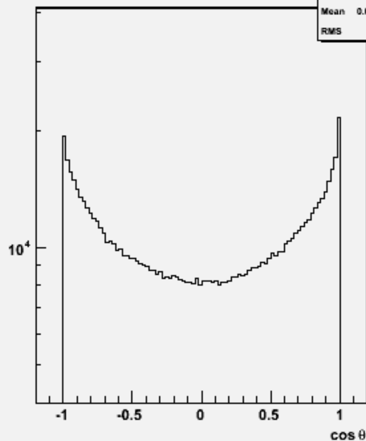
Particle cos \theta : w102424 cce2e2dd_o
