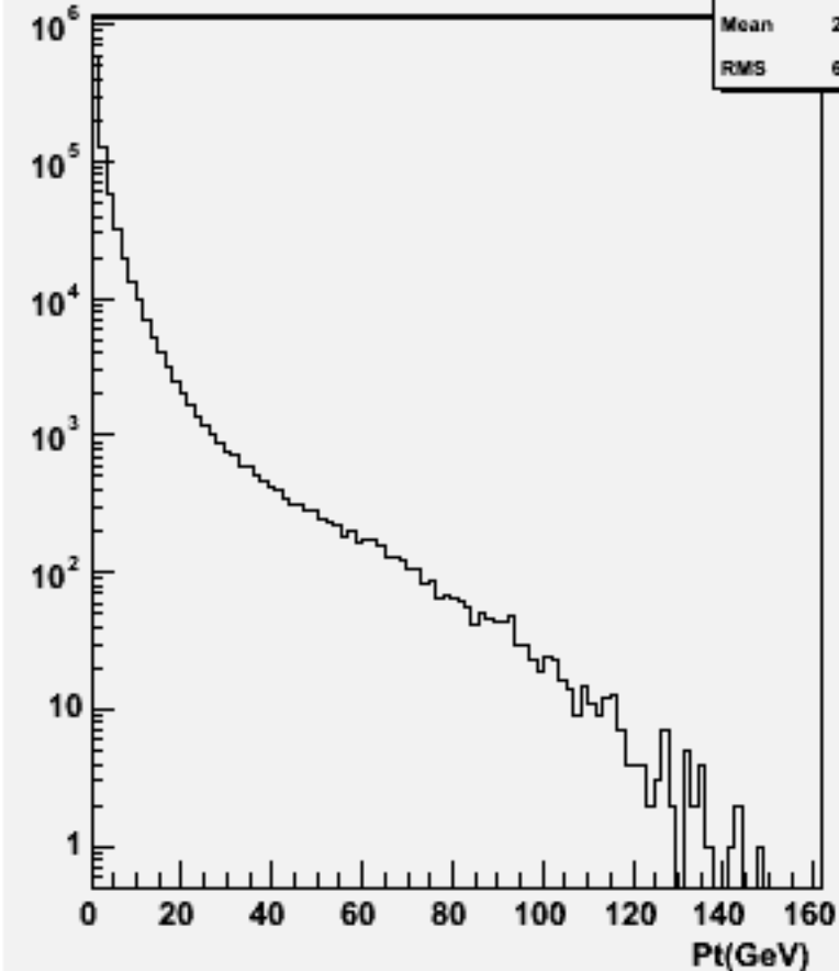
Particle Pt : w102424 cce2e2dd_o
