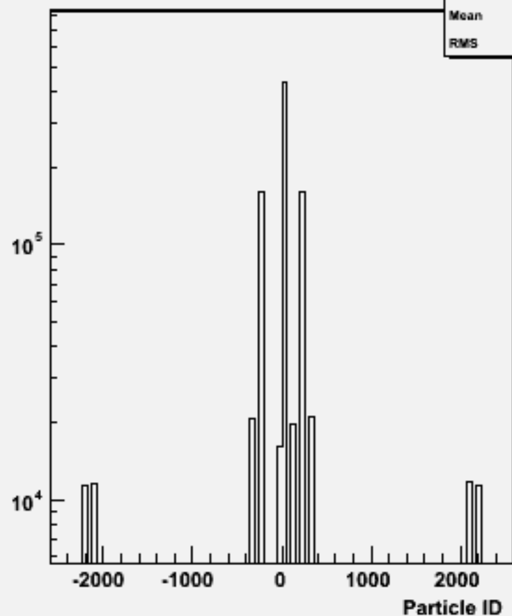
Particle ID : w102424 cce2e2dd_o
