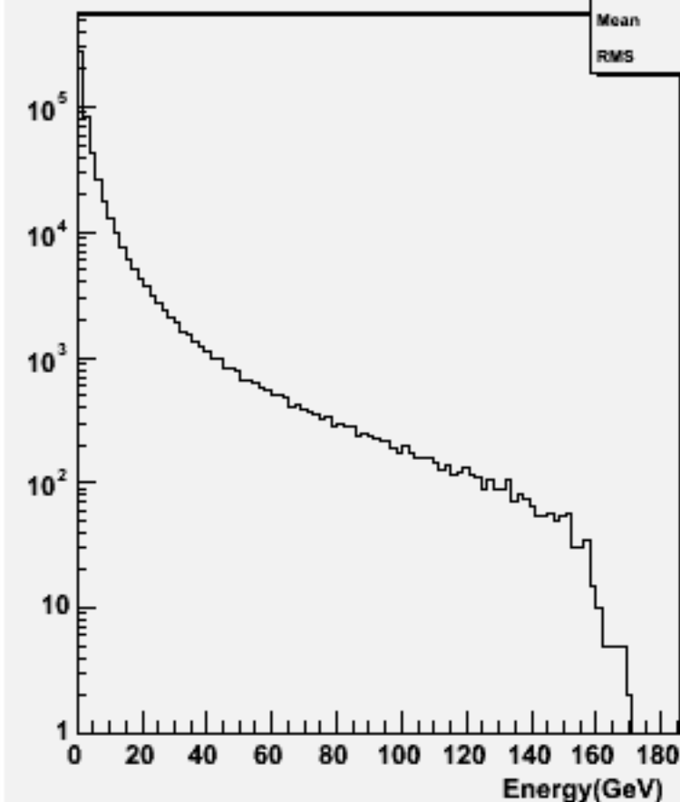
Start point R : w102421 cce2e2e3e3_o
