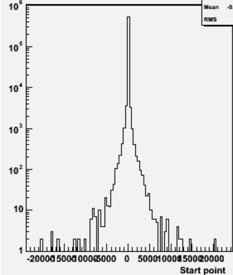
Start point Z : w102421 cce2e2e3e3_o
