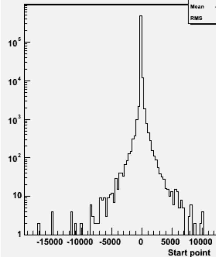
Start point Z : w102416 cce2e2e2e2_o
