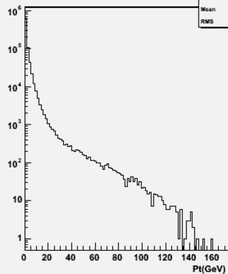
Particle Pt : w102414 cce1e1bb_o
