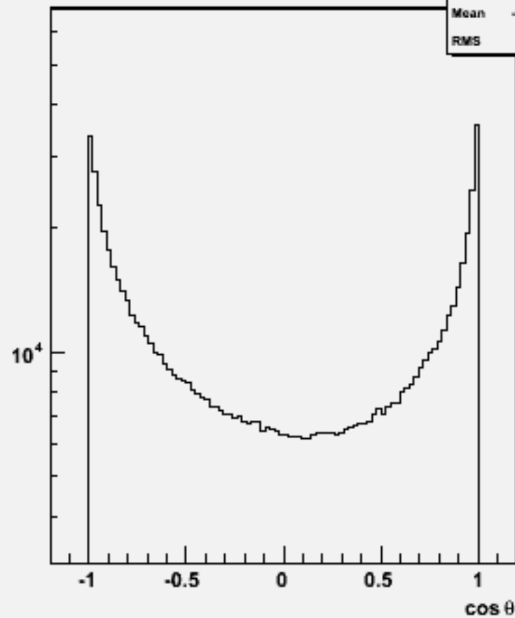
Particle cos \theta : w102414 cce1e1bb_o
