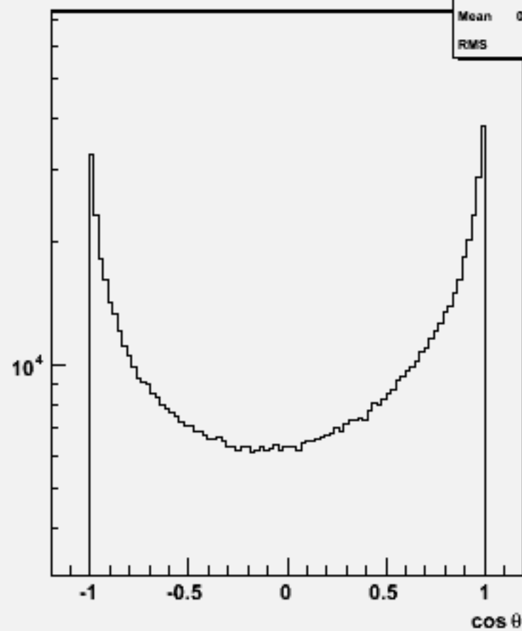
Particle cosθ : w102411 cce1e1bb_o
