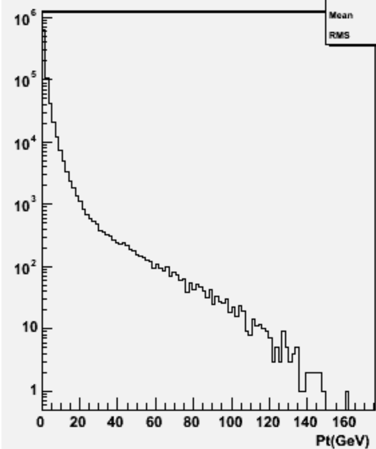
Particle Pt : w102411 cce1e1bb_o
