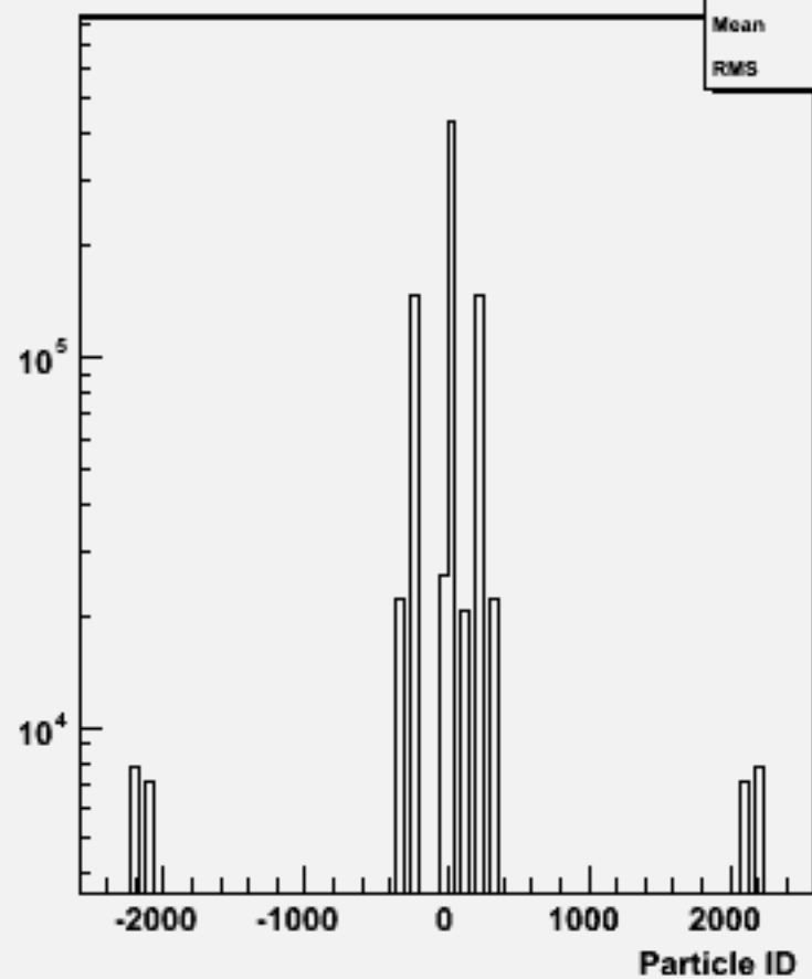
Particle ID : w102411 cce1e1bb_o
