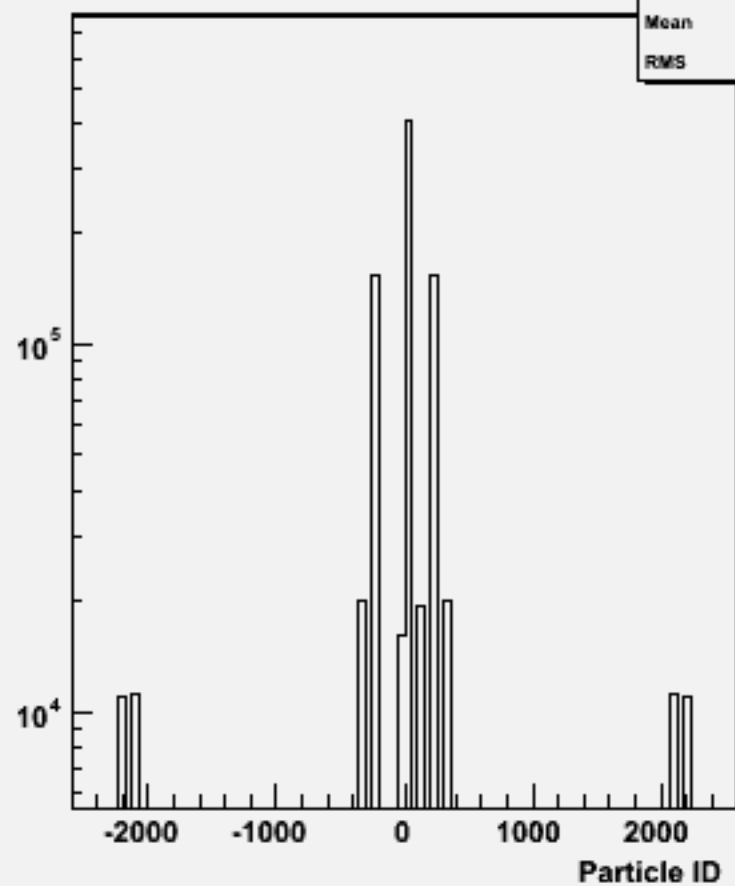
Particle ID : w102409 cce1e1dd_o
