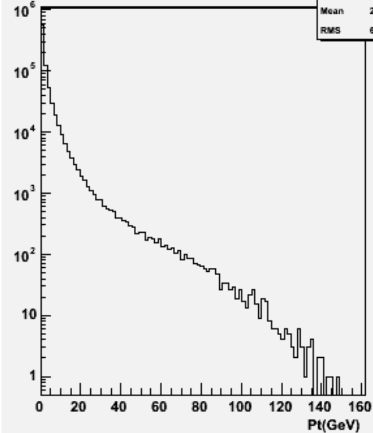
Particle Pt : w102409 cce1e1dd_o
