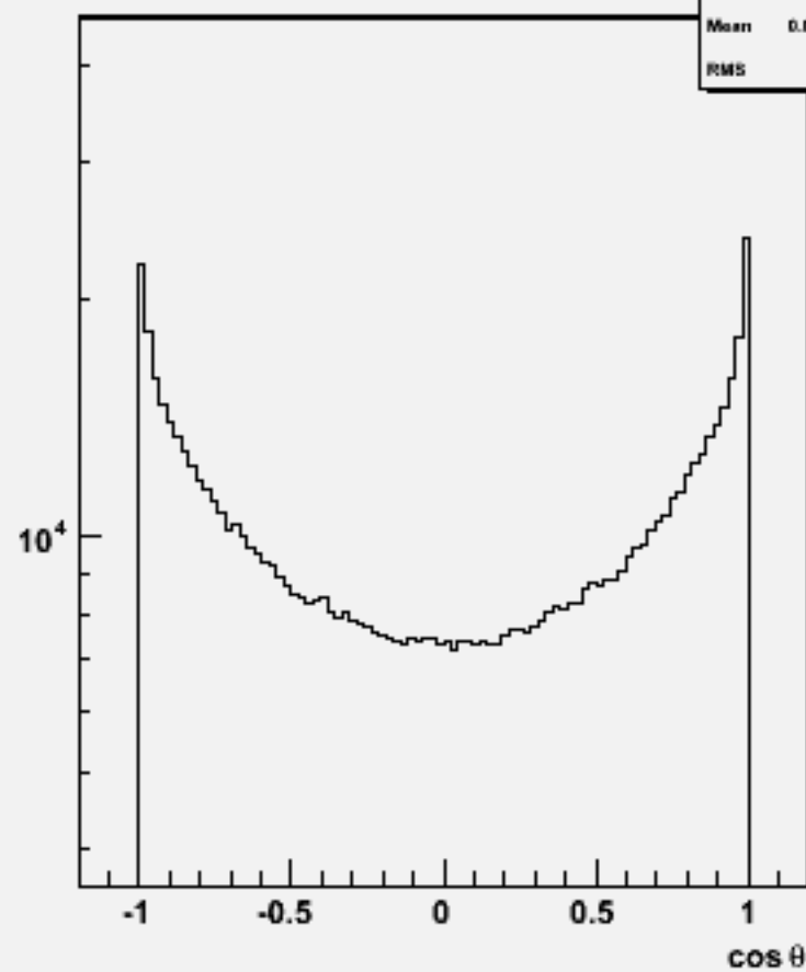
Particle cos \theta : w102409 cce1e1dd_o
