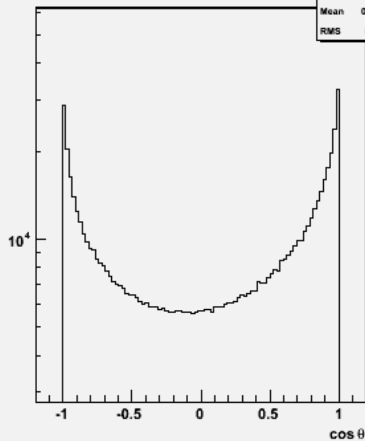
Particle cos \theta : w102407 cce1e1dd_o
