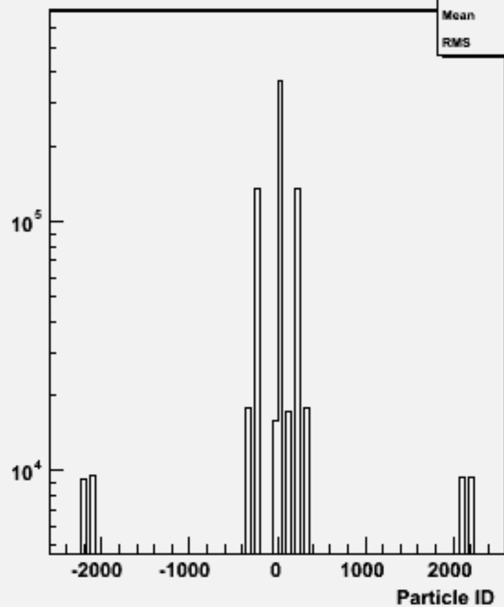
Particle ID : w102407 cce1e1dd_o
