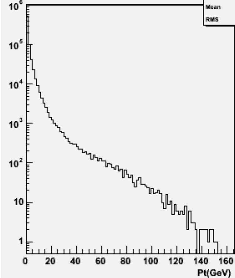
Particle Pt : w102407 cce1e1dd_o
