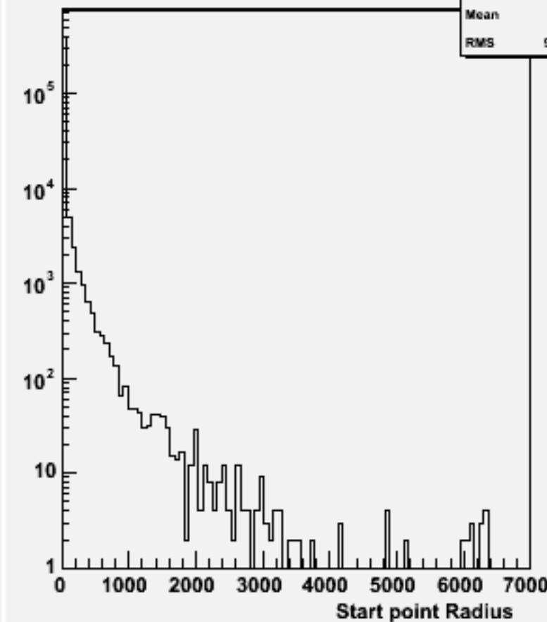
Start point R : w102406 cce1e1e3e3_o
