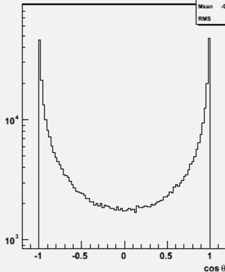
Particle cosθ : w102406 cce1e1e3e3_o
