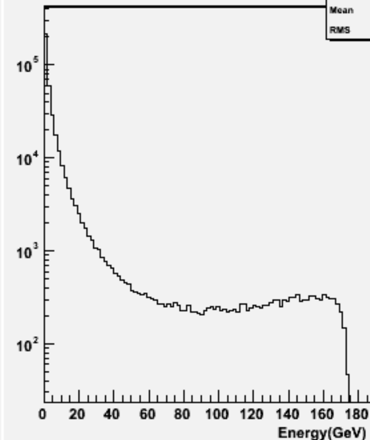
Start point R : w102406 cce1e1e3e3_o
