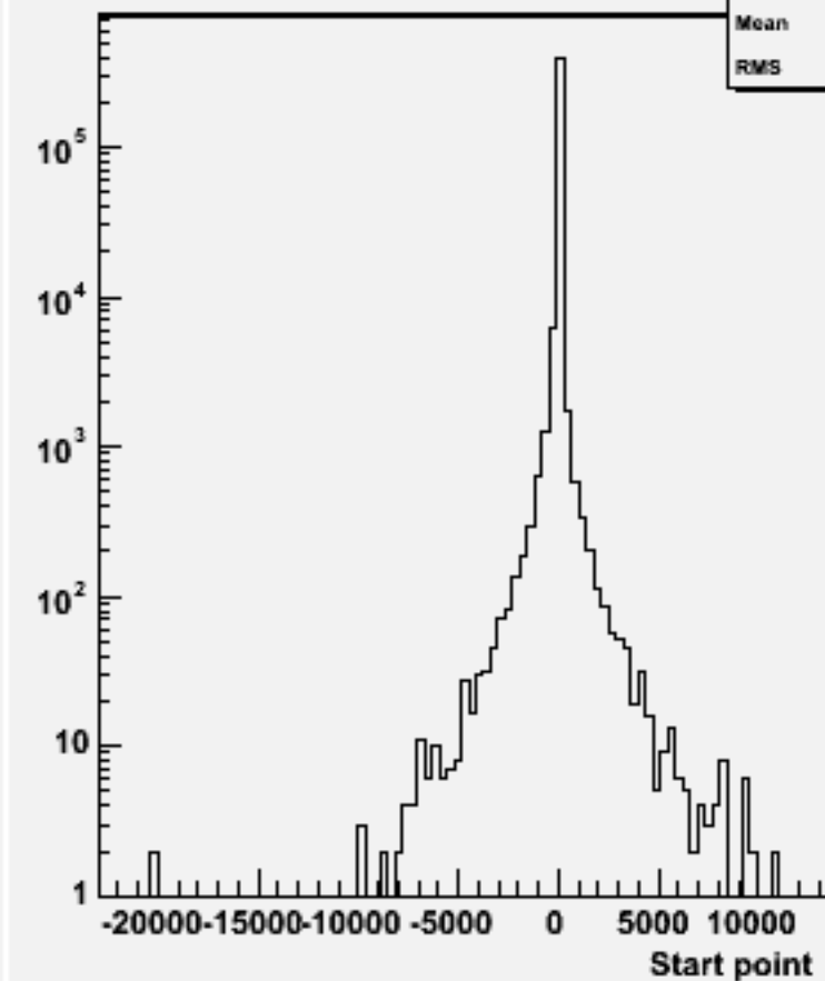
Start point Z : w102406 cce1e1e3e3_o
