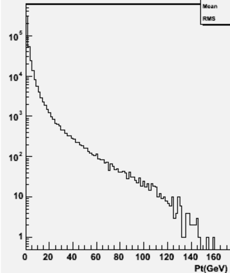
Start point Z : w102405 cce1e1e3e3_o
