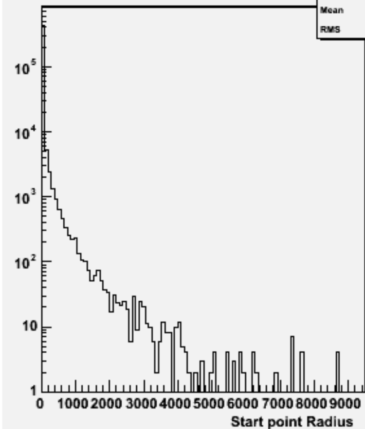
Start point R : w102405 cce1e1e3e3_o
