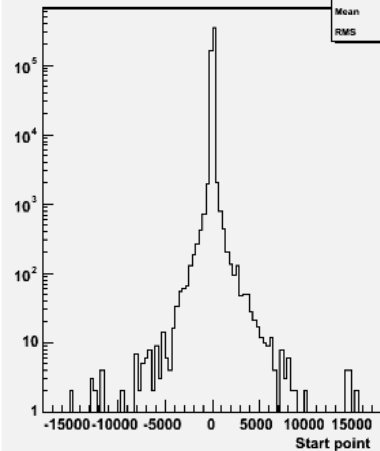
Start point Z : w102404 cce1e1e3e3_o
