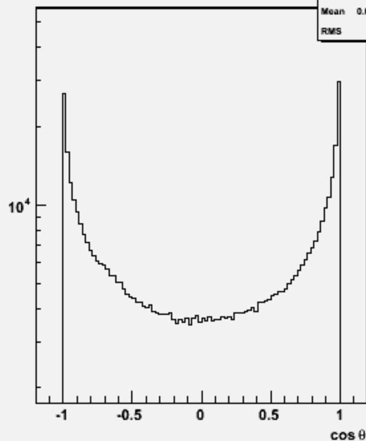
Particle cosθ : w102404 cce1e1e3e3_o
