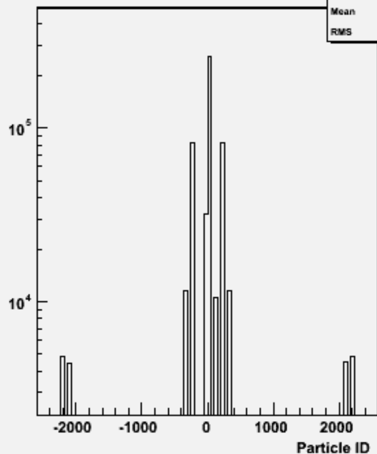
Particle ID : w102404 cce1e1e3e3_o
