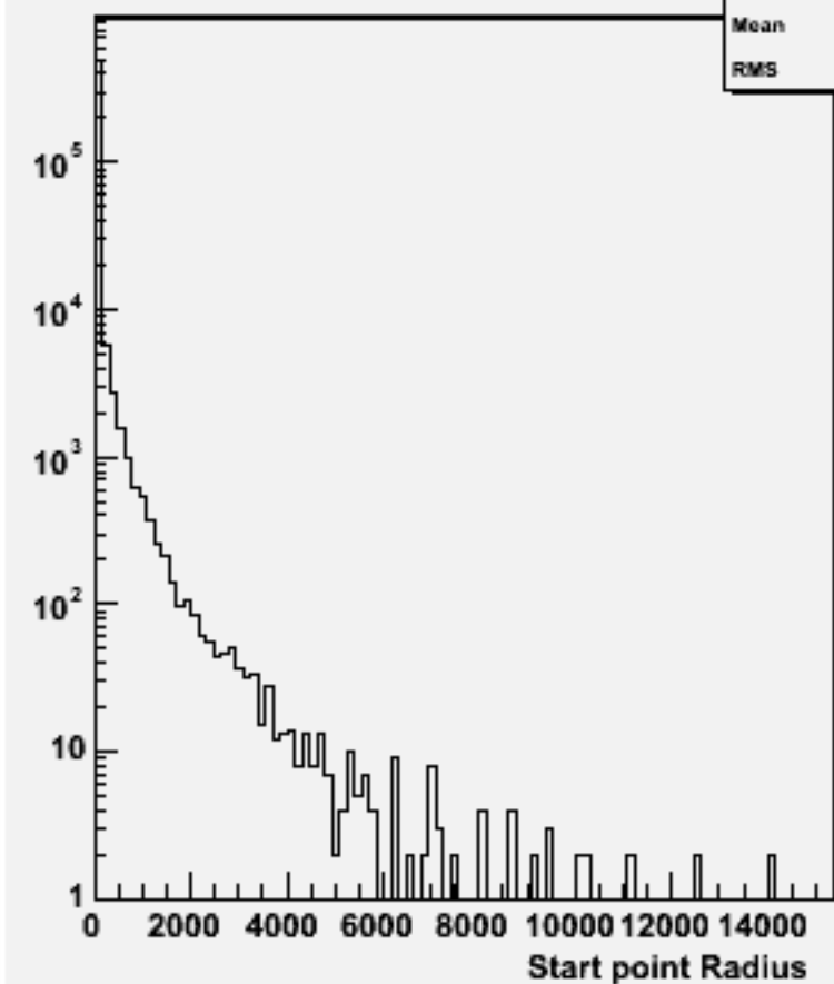
Start point R : w102404 cce1e1e3e3_o
