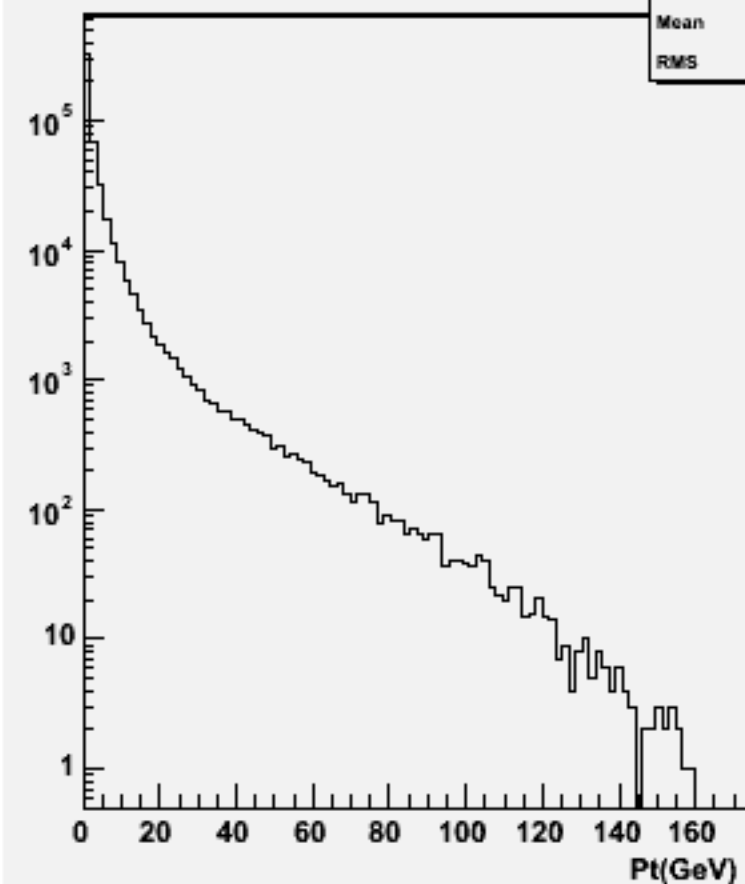
Particle Pt : w102404 cce1e1e3e3_o
