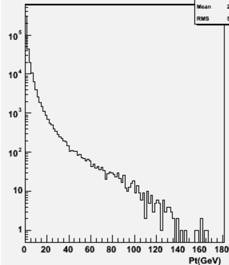
Particle Pt : w102403 cce1e1e3e3_o
