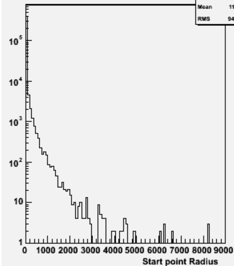
Start point R : w102403 cce1e1e3e3_o
