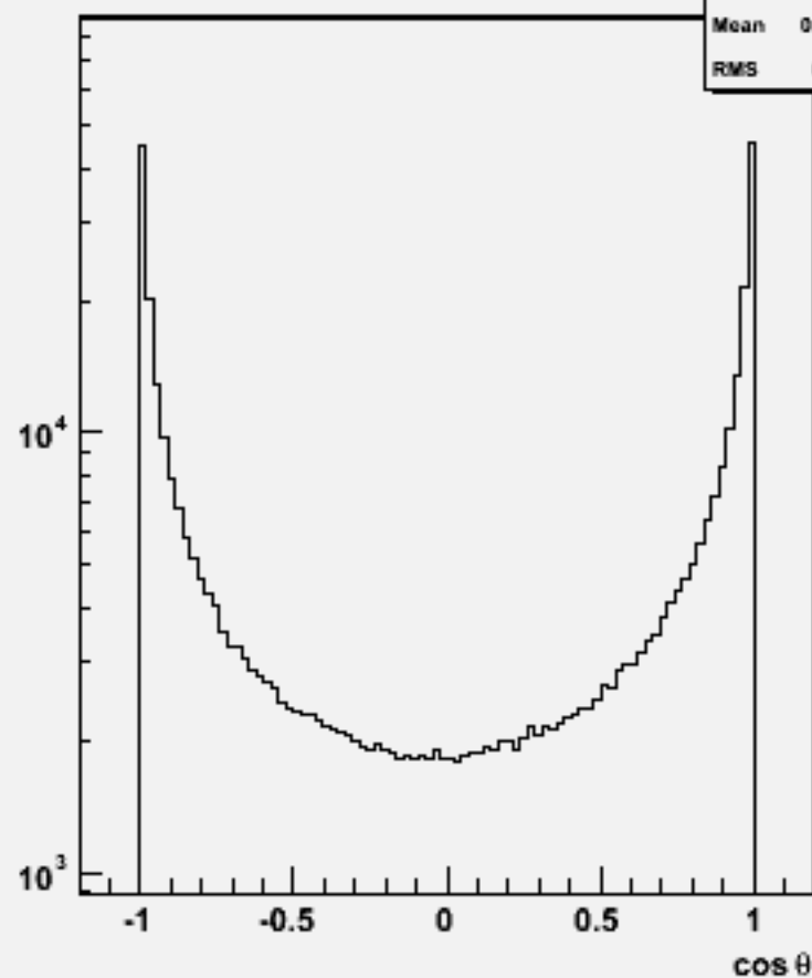
Particle cos \theta : w102403 cce1e1e3e3_o
