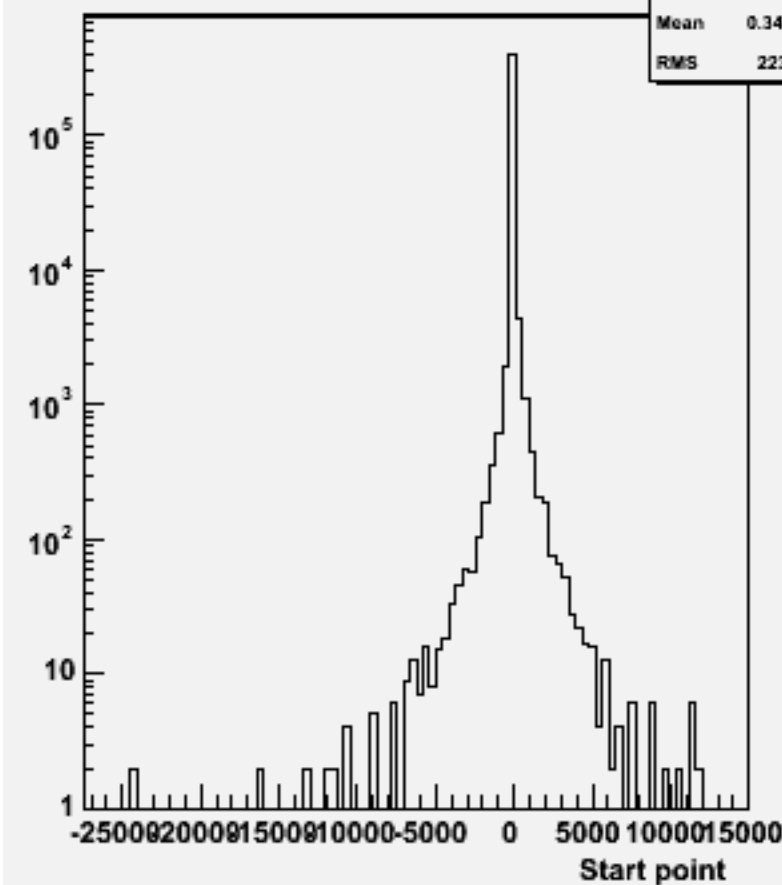
Start point Z : w102403 cce1e1e3e3_o
