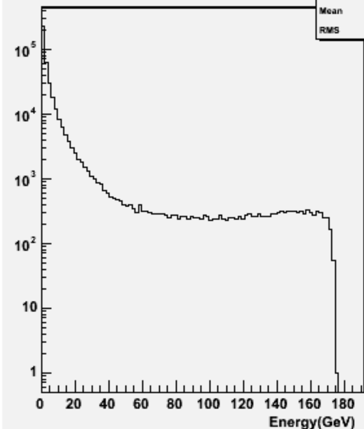
Particle Energy : w102403 cce1e1e3e3_o
