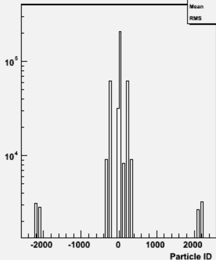
Particle ID : w102403 cce1e1e3e3_o
