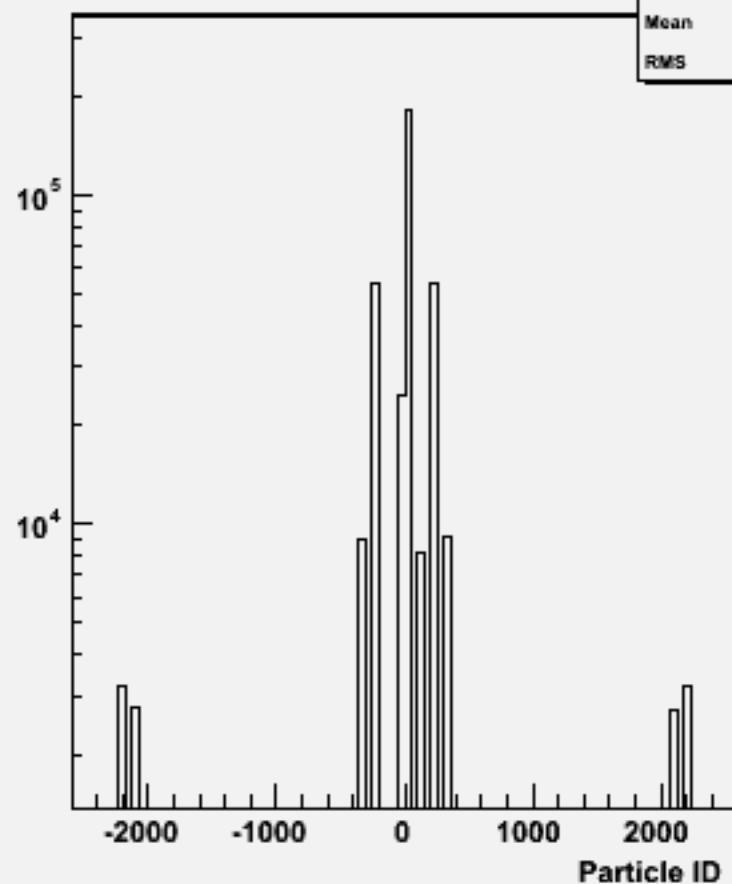
Particle ID : w102402 cce1e1e2e2_o
