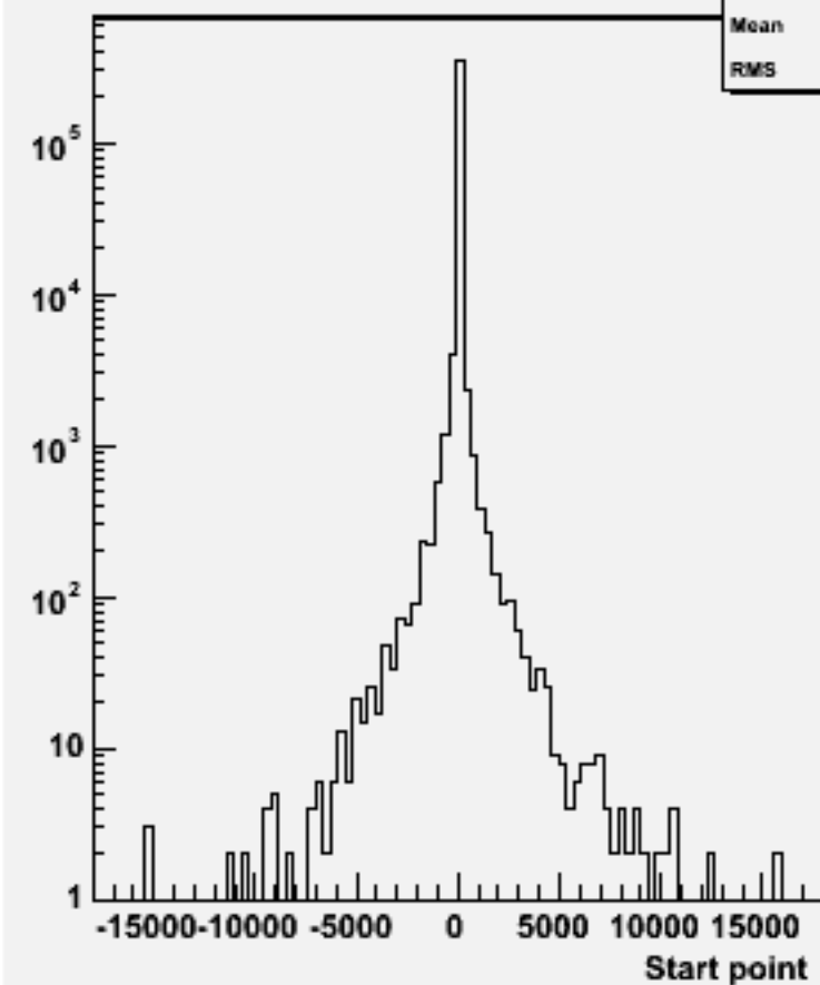
Start point Z : w102402 cce1e1e2e2_o
