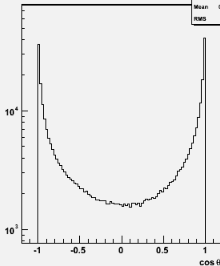
Particle cosθ : w102402 cce1e1e2e2_o
