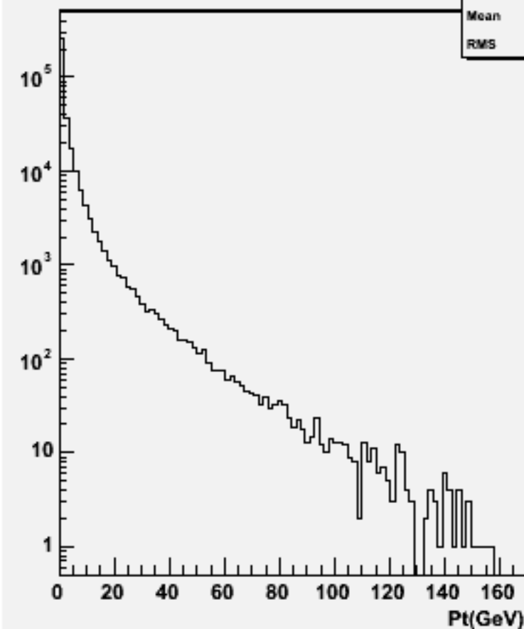
Particle Pt : w102402 cce1e1e2e2_o
