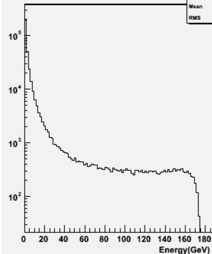
Particle Energy : w102402 cce1e1e2e2_o
