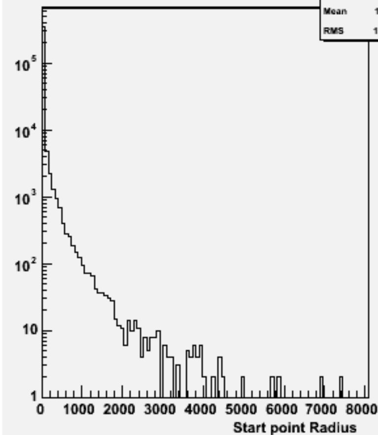
Start point R : w102402 cce1e1e2e2_o
