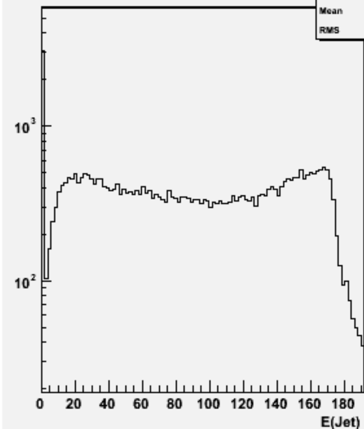
Jet energies(All jets)w102401 cce1e1e2e2_o
