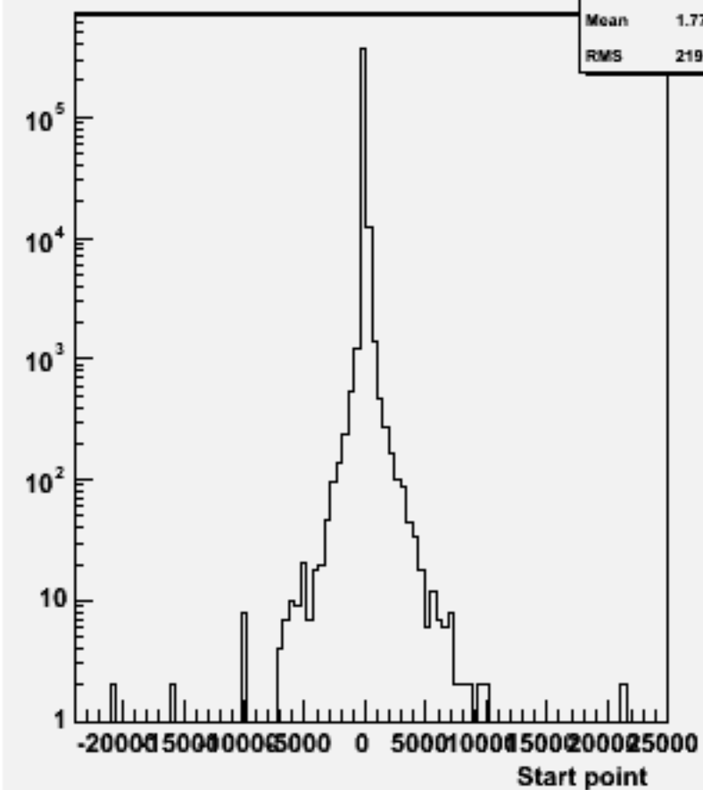
Start point Z : w102401 cce1e1e2e2_o
