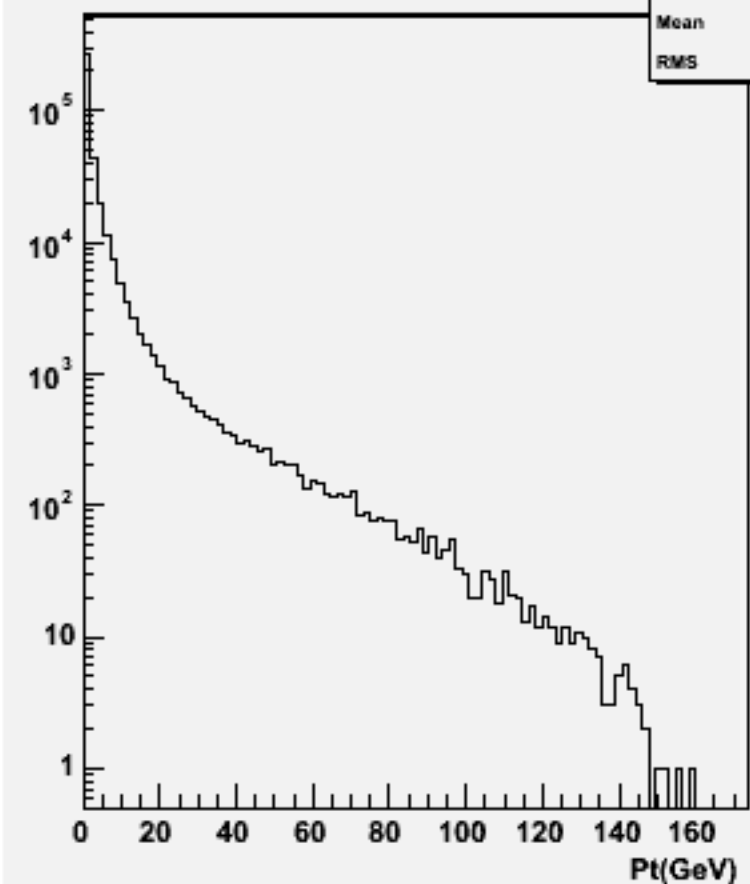
Particle Pt : w102401 cce1e1e2e2_o
