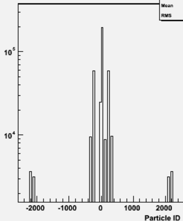
Particle ID : w102401 cce1e1e2e2_o
