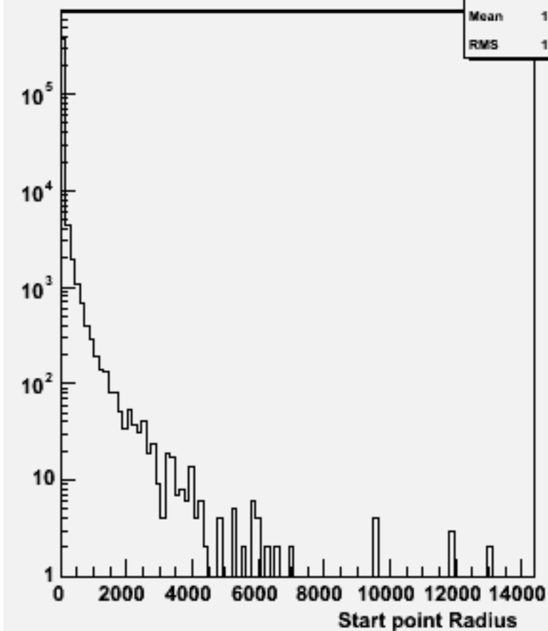
Start point R : w102401 cce1e1e2e2_o
