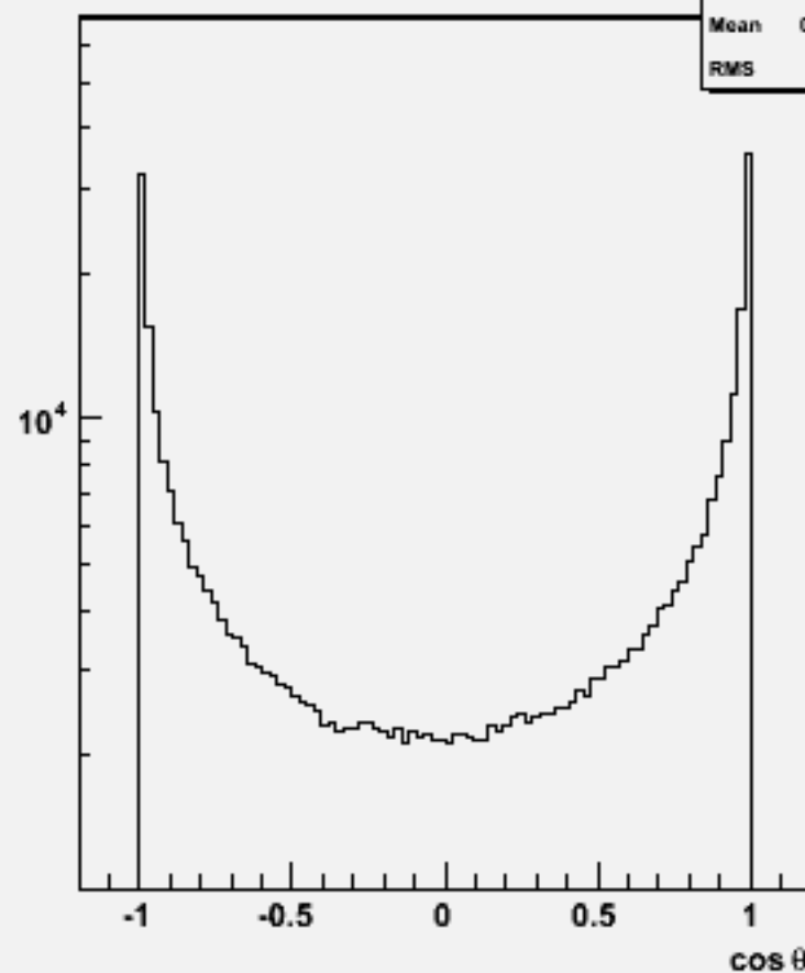
Particle cosθ : w102401 cce1e1e2e2_o
