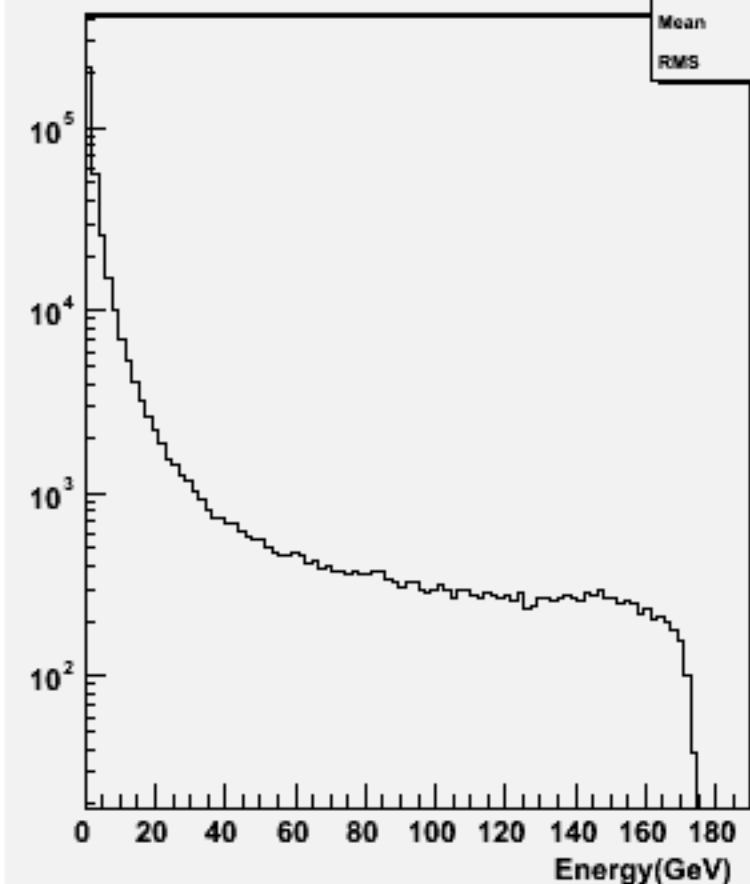
Particle Energy : w102401 cce1e1e2e2_o
