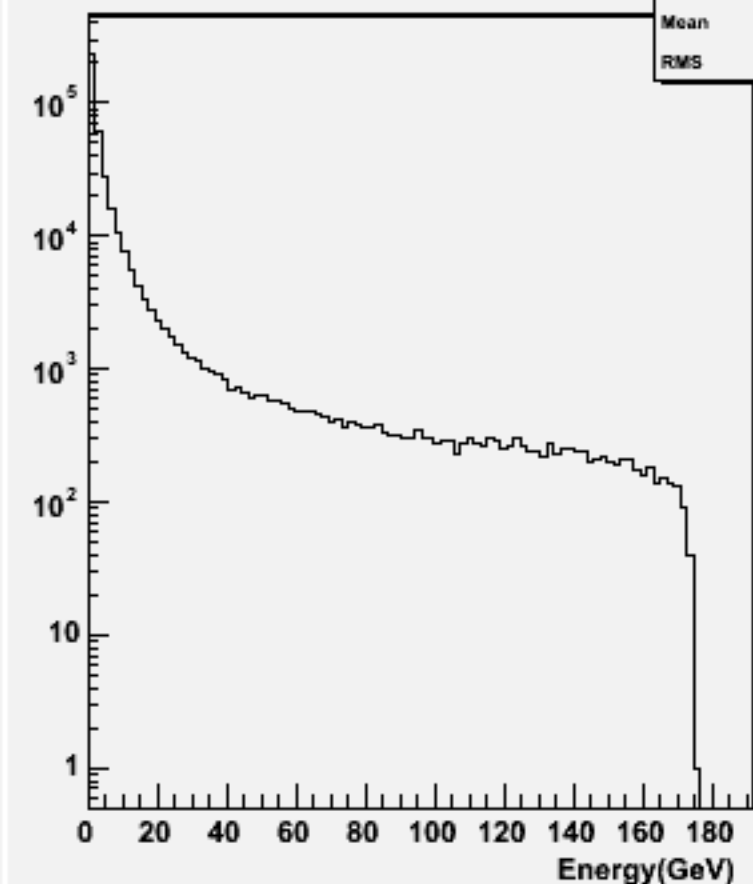
Start point R : w102400 cce1e1e2e2_o
