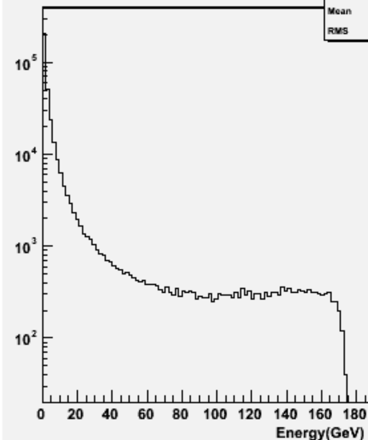
Start point R : w102399 cce1e1e2e2_o
