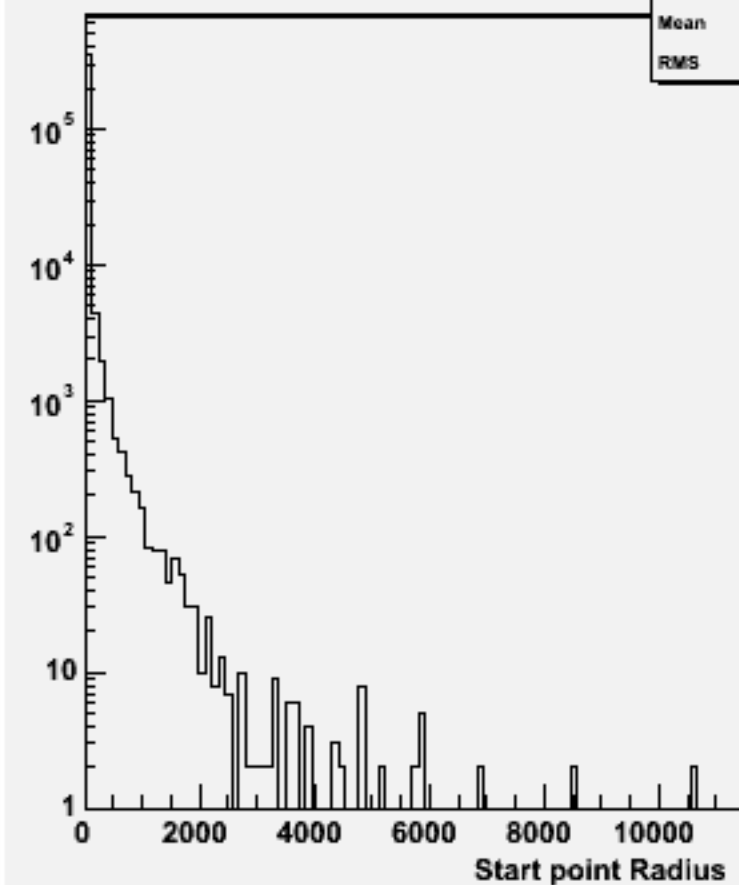
Start point R : w102399 cce1e1e2e2_o
