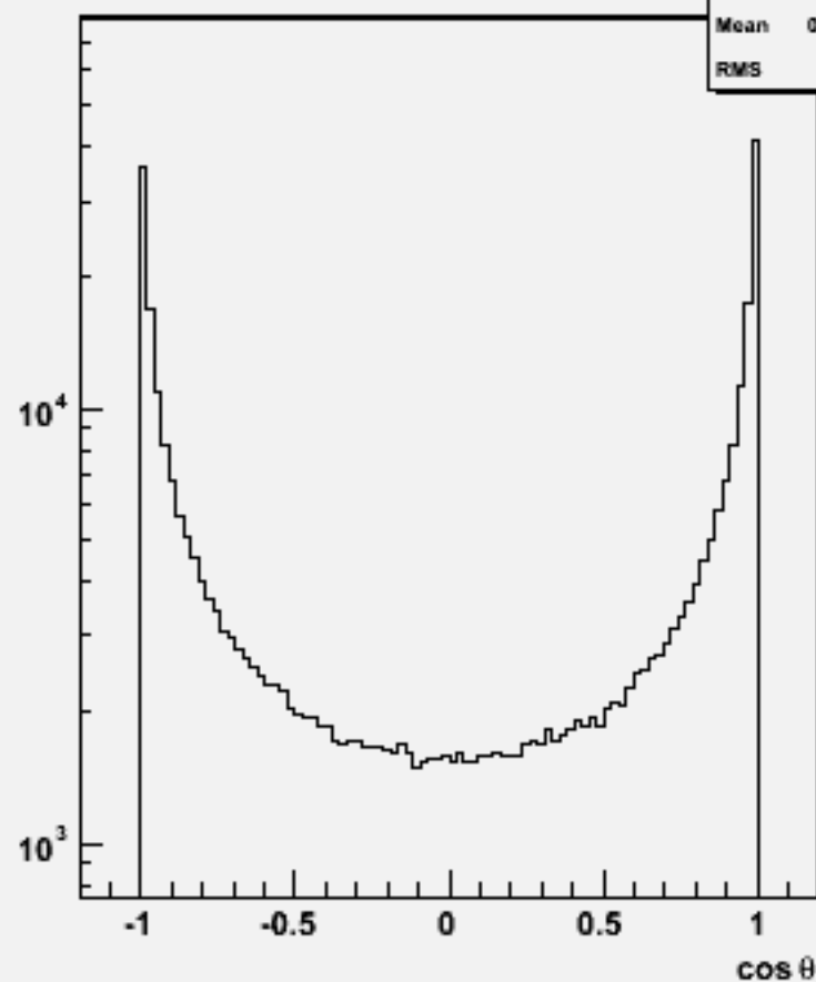
Particle cosθ : w102398 cce1e1e1e1_o
