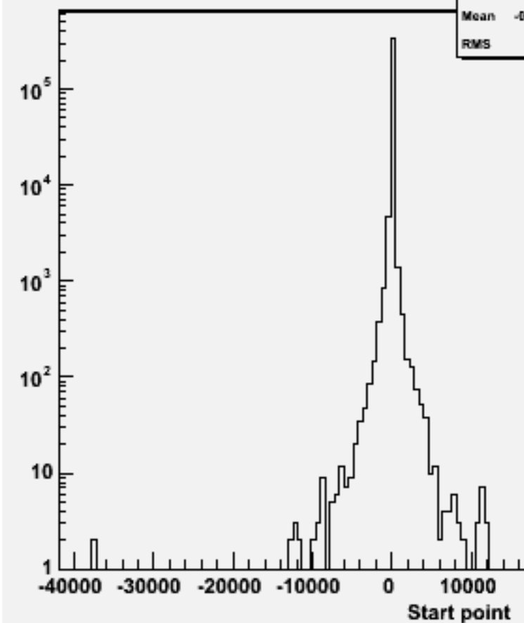
Start point Z : w102398 cce1e1e1e1_o
