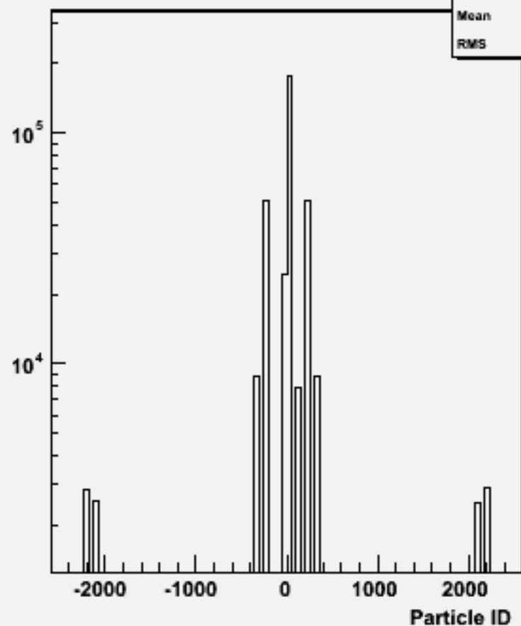
Particle ID : w102398 cce1e1e1e1_o
