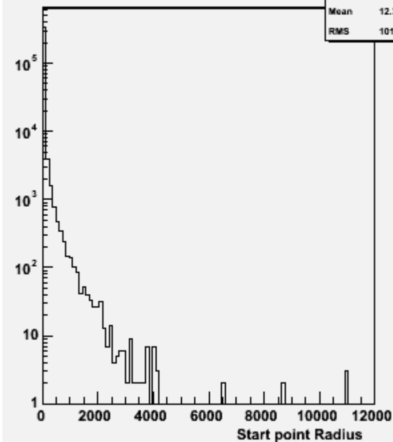
Start point R : w102398 cce1e1e1e1_o
