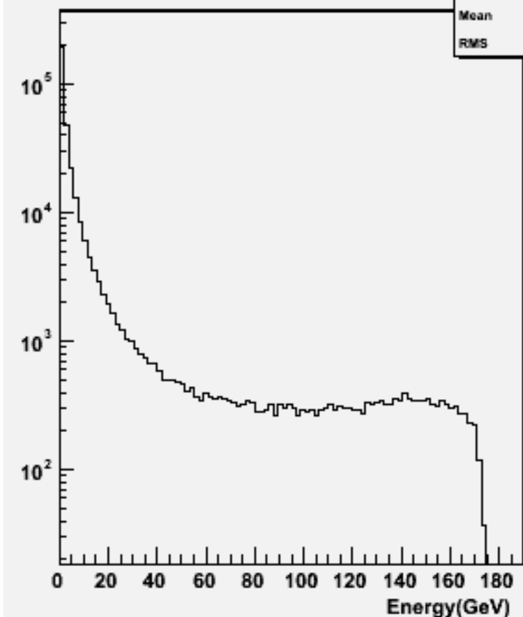
Particle Energy : w102398 cce1e1e1e1_o
