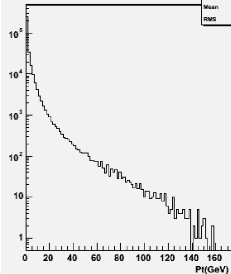
Particle Pt : w102398 cce1e1e1e1_o
