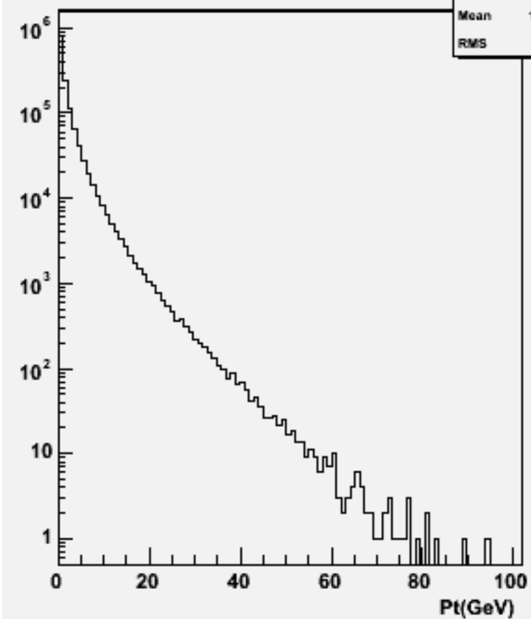
Particle Pt : w102393 uubbbb_o
