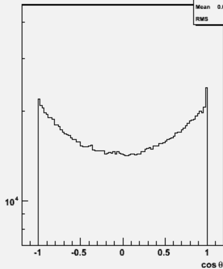
Particle cos \theta : w102393 uubbbb_o
