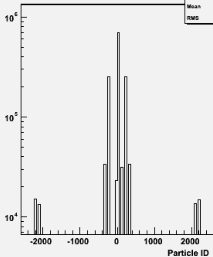
Particle ID : w102393 uubbbb_o
