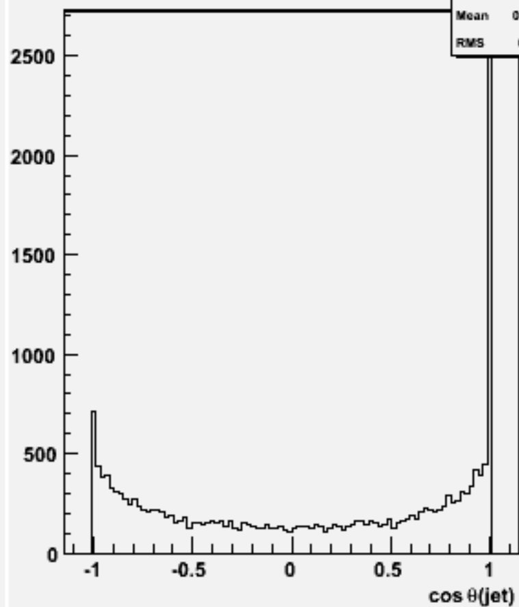
cos \theta for 2-jets :w102389 uussbb_o
