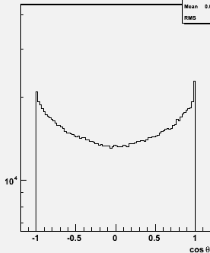
Particle \cos\theta : w102389 uussbb_o
