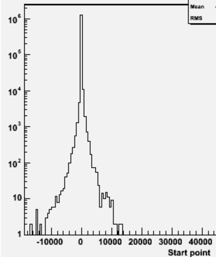
Start point Z : w102389 uussbb_o
