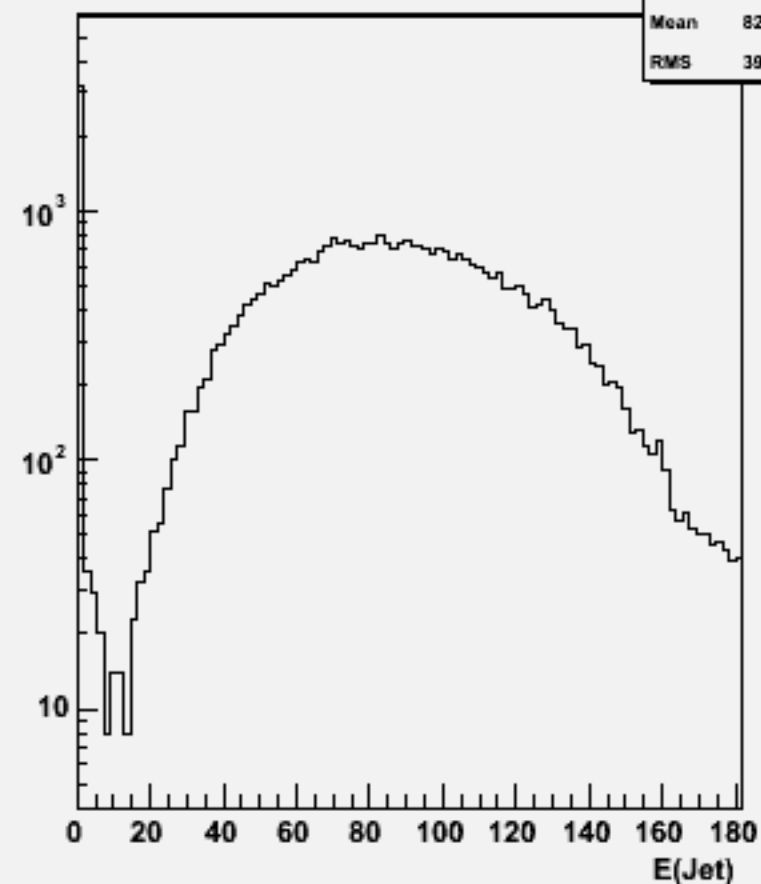
Jet energies(All jets)w102389 uussbb_o
