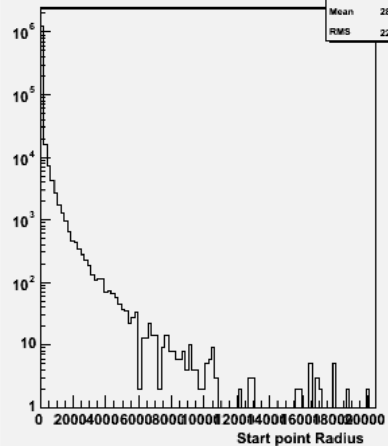
Start point R : w102389 uussbb_o
