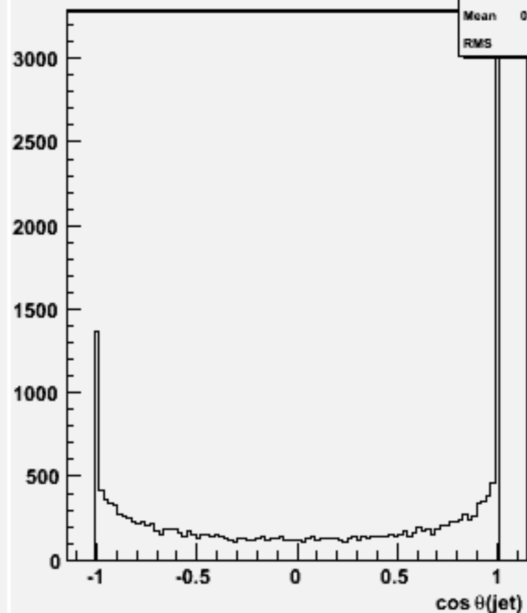
cos \theta for 2-jets :w102385 uussss_o
