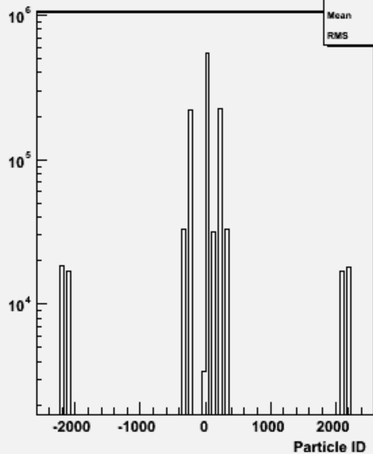
Particle ID : w102385 uussss_o
