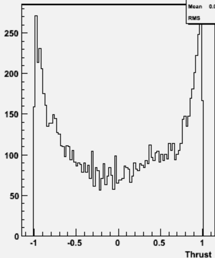
cos \Theta (thrust) w102385 uussss_o
