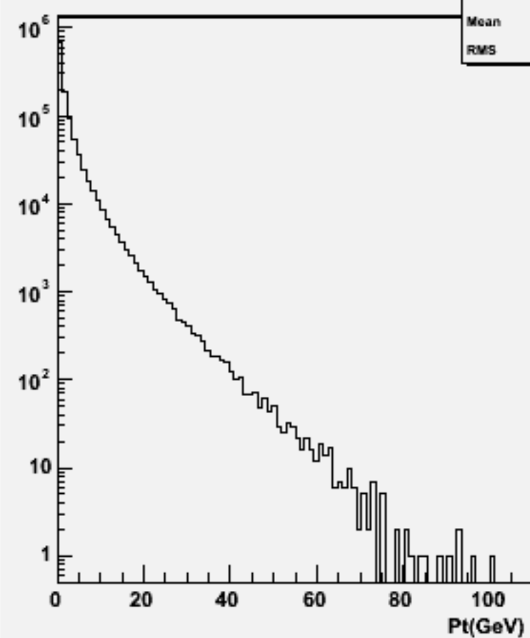
Particle Pt : w102385 uussss_o
