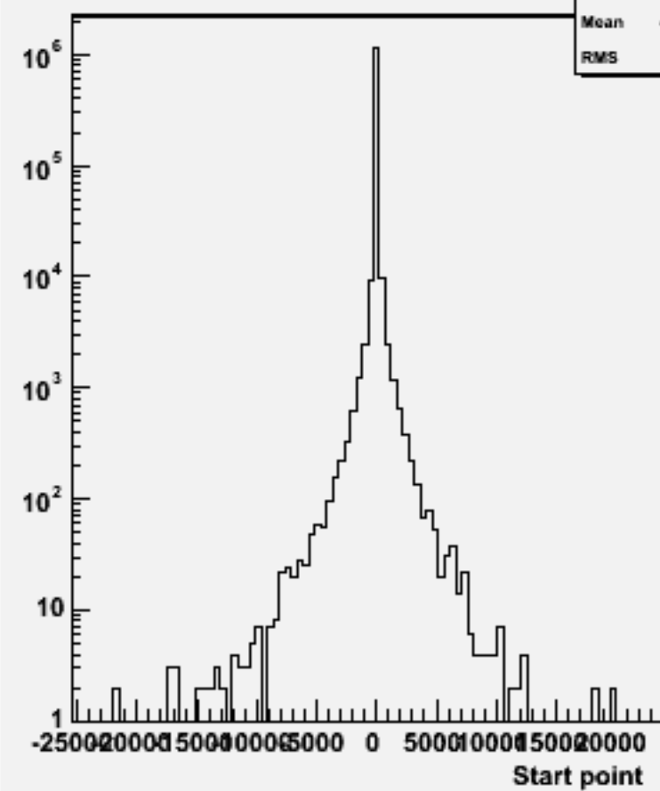
Start point Z : w102385 uussss_o
