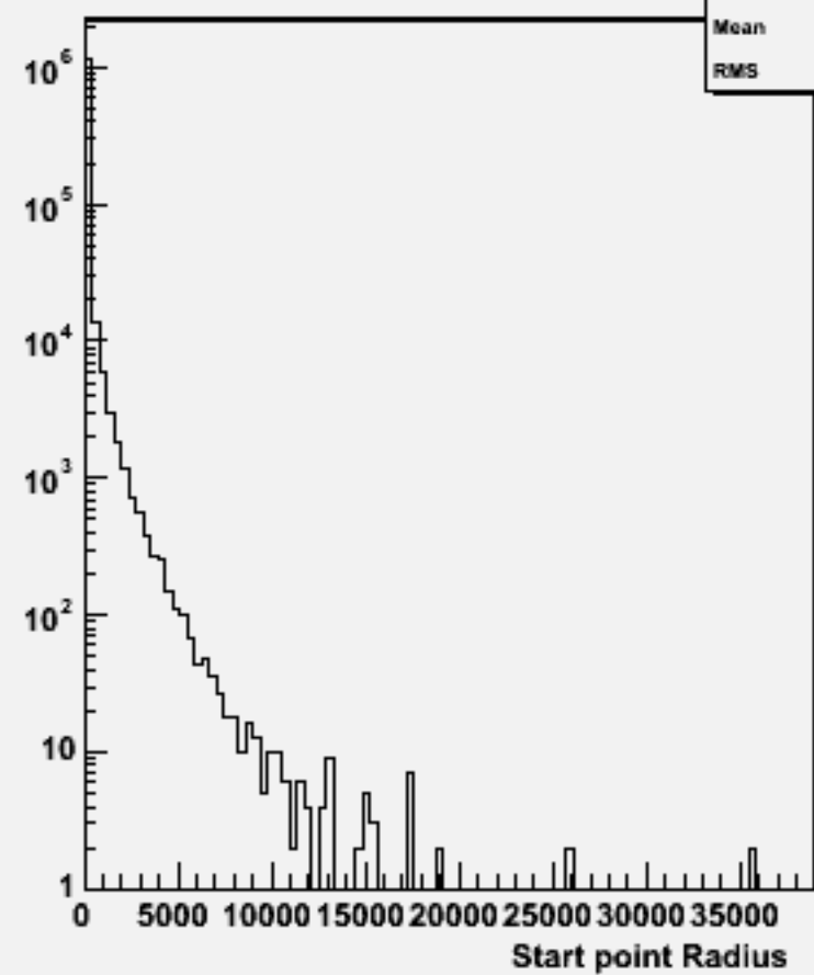
Start point R : w102385 uussss_o
