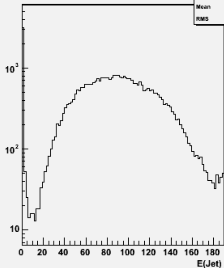
Jet energies(All jets)w102385 uussss_o
