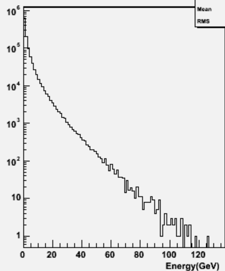
Particle Energy : w102385 uussss_o
