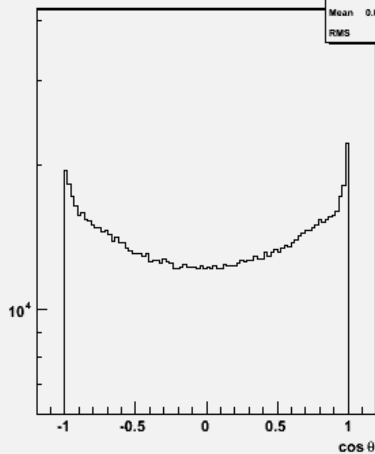
Particle cos \theta : w102385 uussss_o
