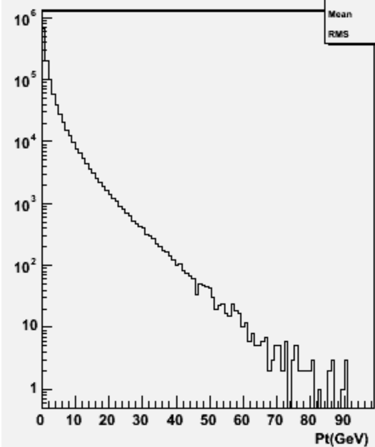
Particle Pt : w102384 uussss_o
