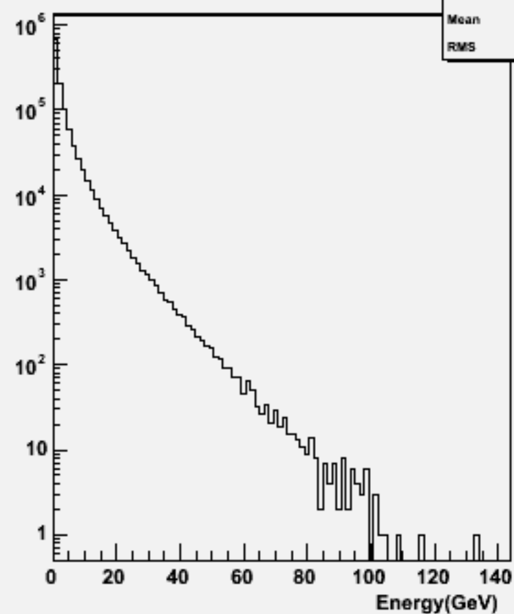
Particle Energy : w102384 uussss_o
