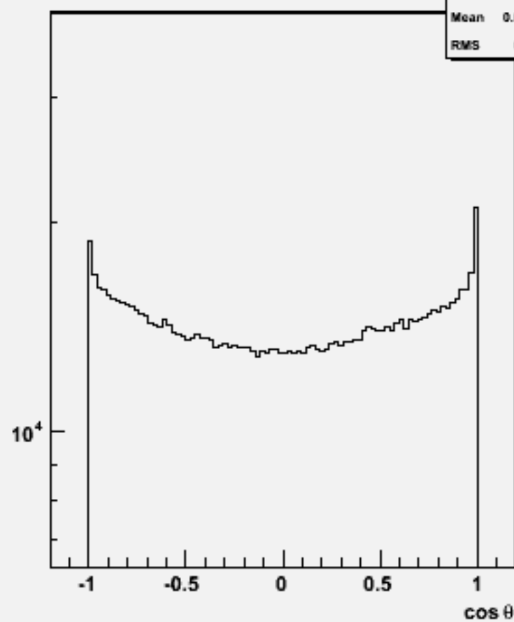
Particle cosθ : w102384 uussss_o
