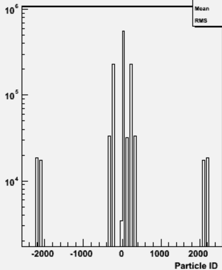
Particle ID : w102384 uussss_o
