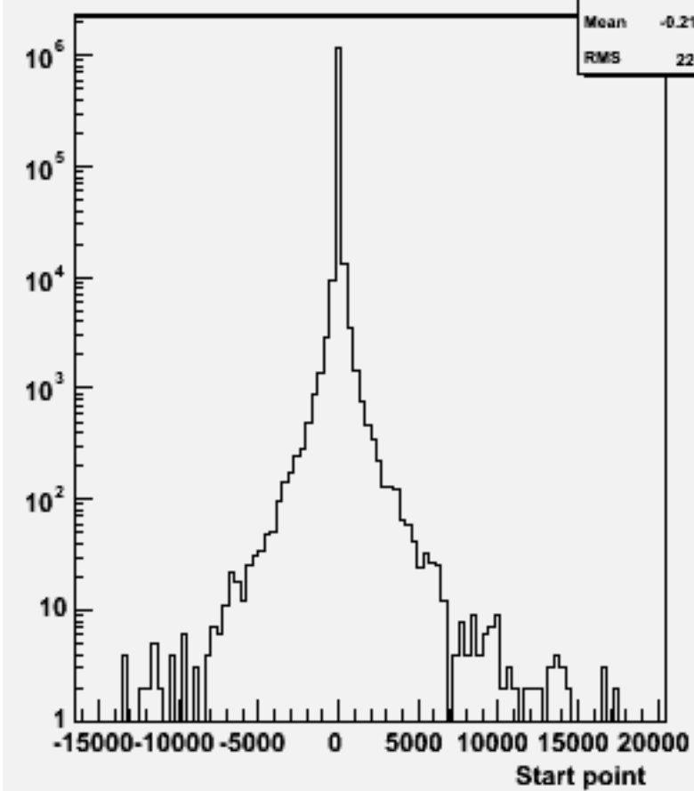
Start point Z : w102384 uussss_o
