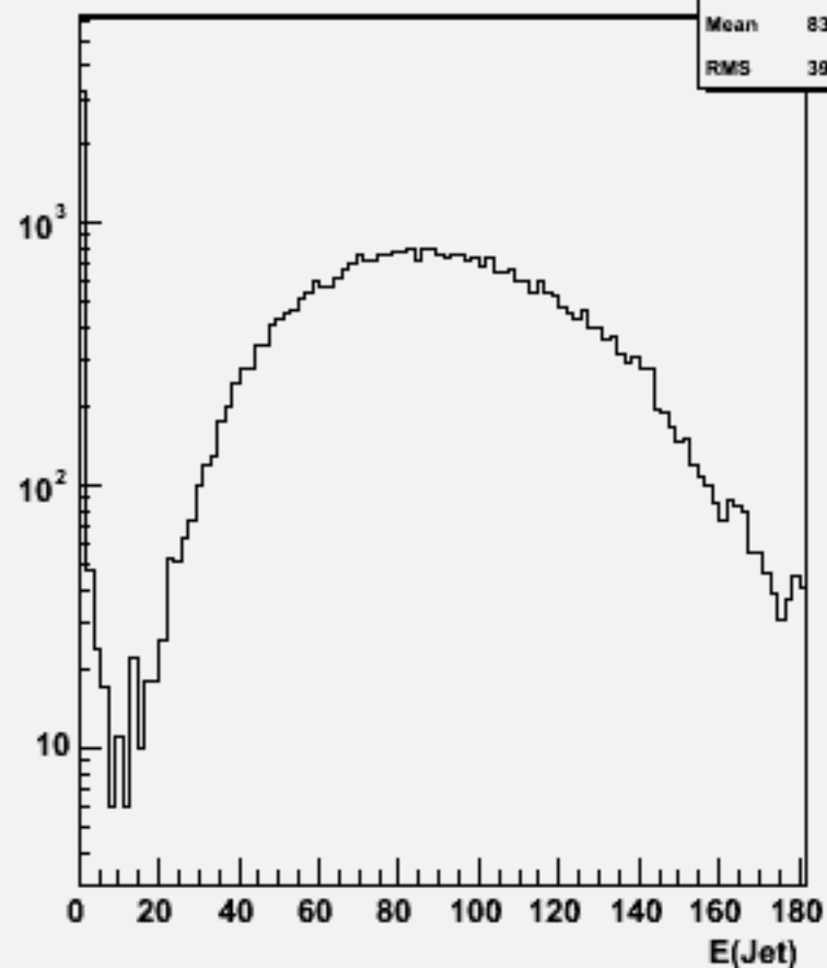
Jet energies(All jets)w102384 uussss_o
