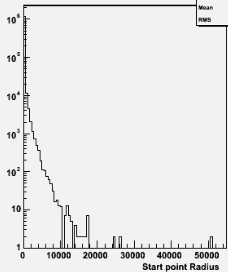
Start point R : w102384 uussss_o
