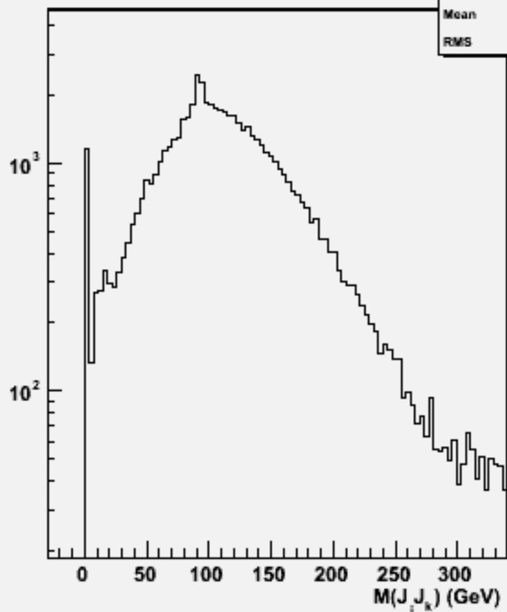
2jets mass(All comb)w102380 uue3e3bb_o
