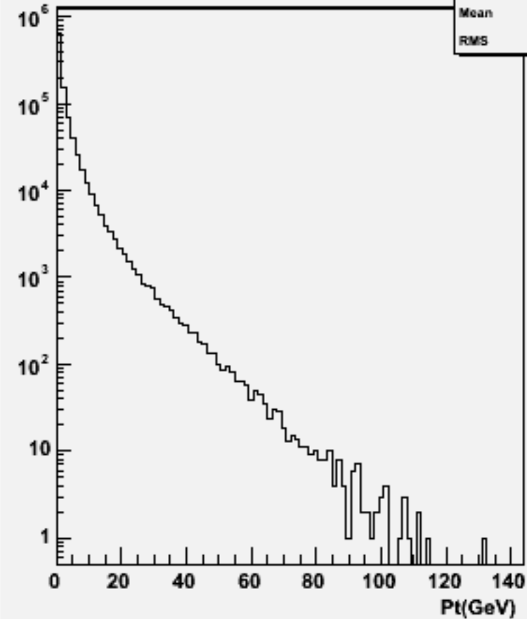
Particle Pt : w102380 uue3e3bb_o
