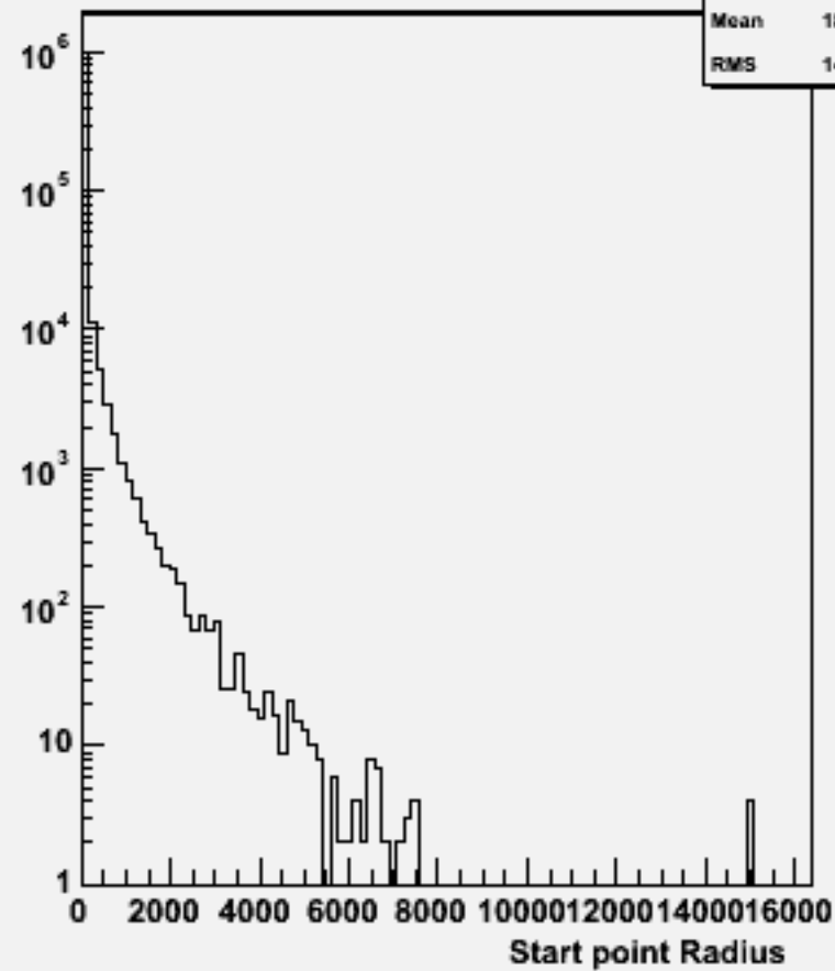
Start point R : w102380 uue3e3bb_o
