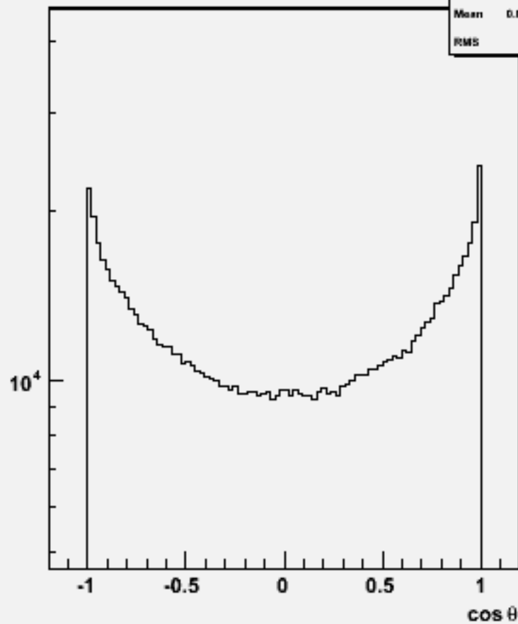
Particle cos \theta : w102380 uue3e3bb_o
