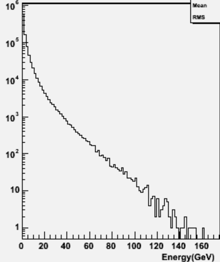
Particle Energy : w102380 uue3e3bb_o
