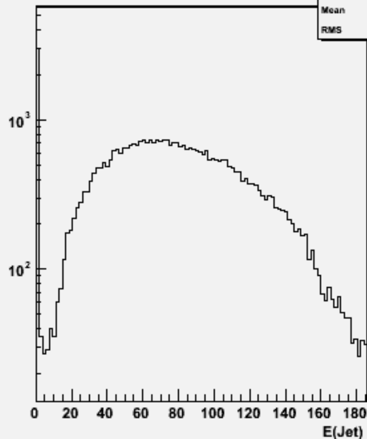
Jet energies(All jets)w102380 uue3e3bb_o
