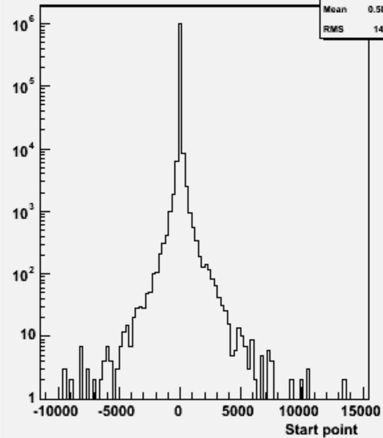
Start point Z : w102380 uue3e3bb_o
