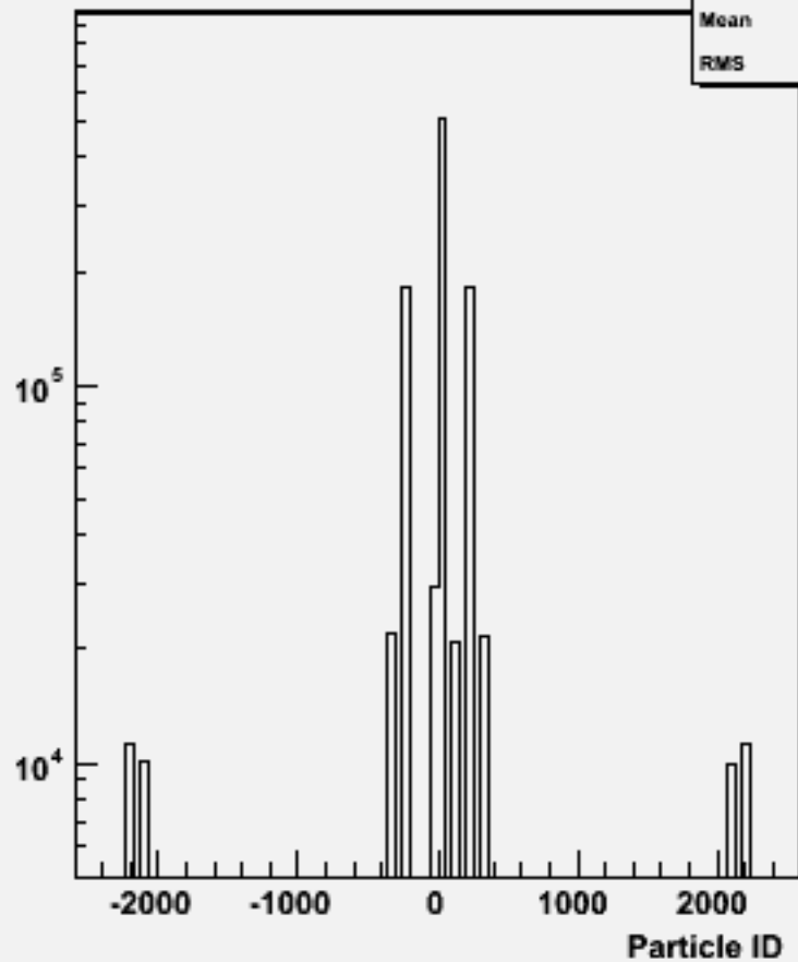
Particle ID : w102380 uue3e3bb_o
