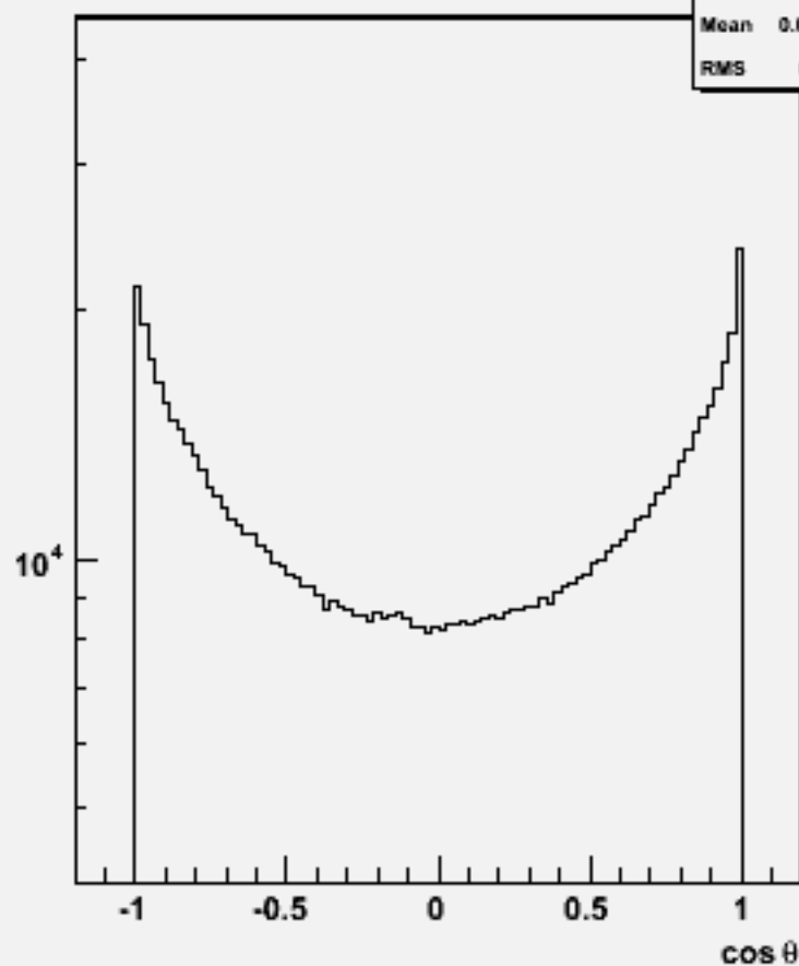
Particle cos \theta : w102369 uue2e2bb_o
