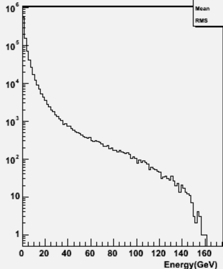
Particle Energy : w102369 uue2e2bb_o
