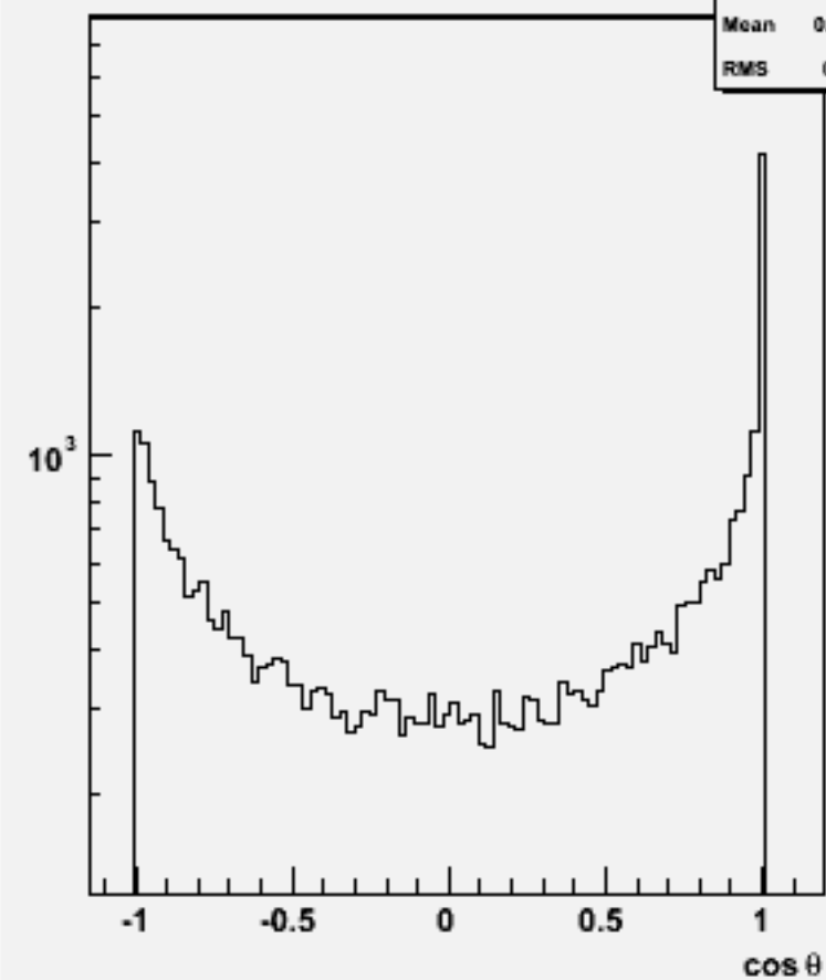
Jet cosθ (All jets)w102369 uue2e2bb_o
