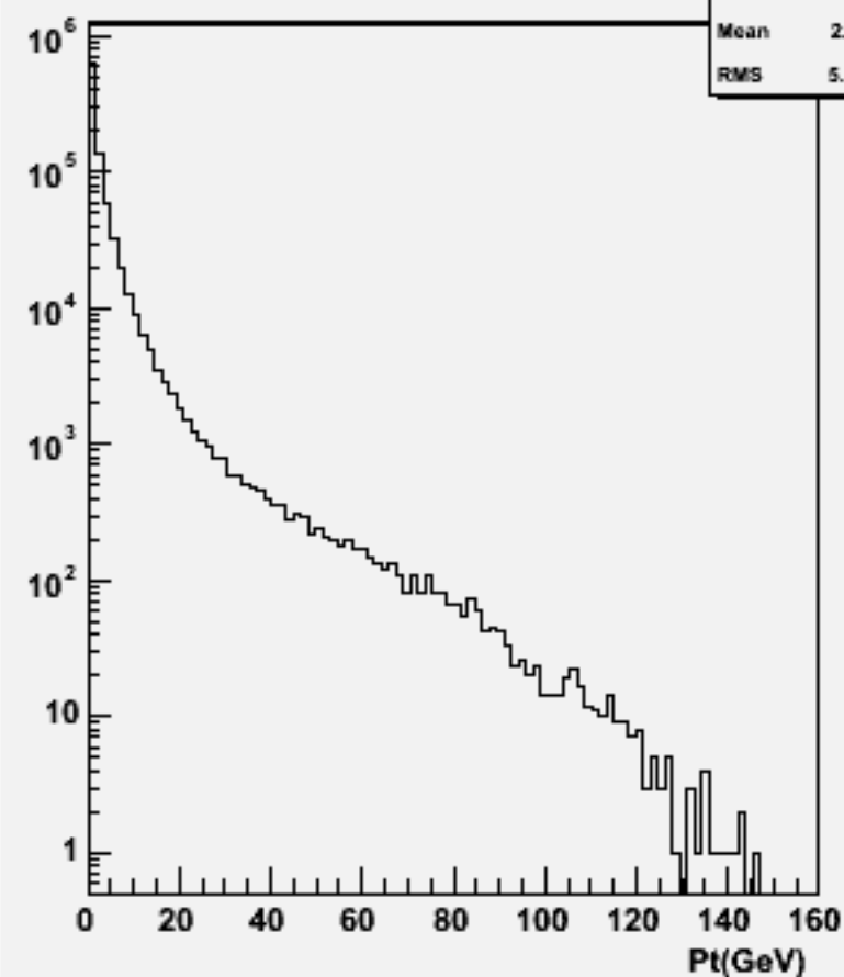
Particle Pt : w102369 uue2e2bb_o
