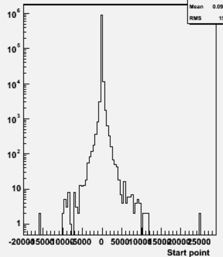
Start point Z : w102369 uue2e2bb_o
