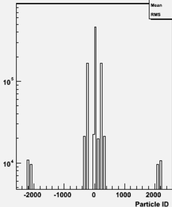
Particle ID : w102369 uue2e2bb_o
