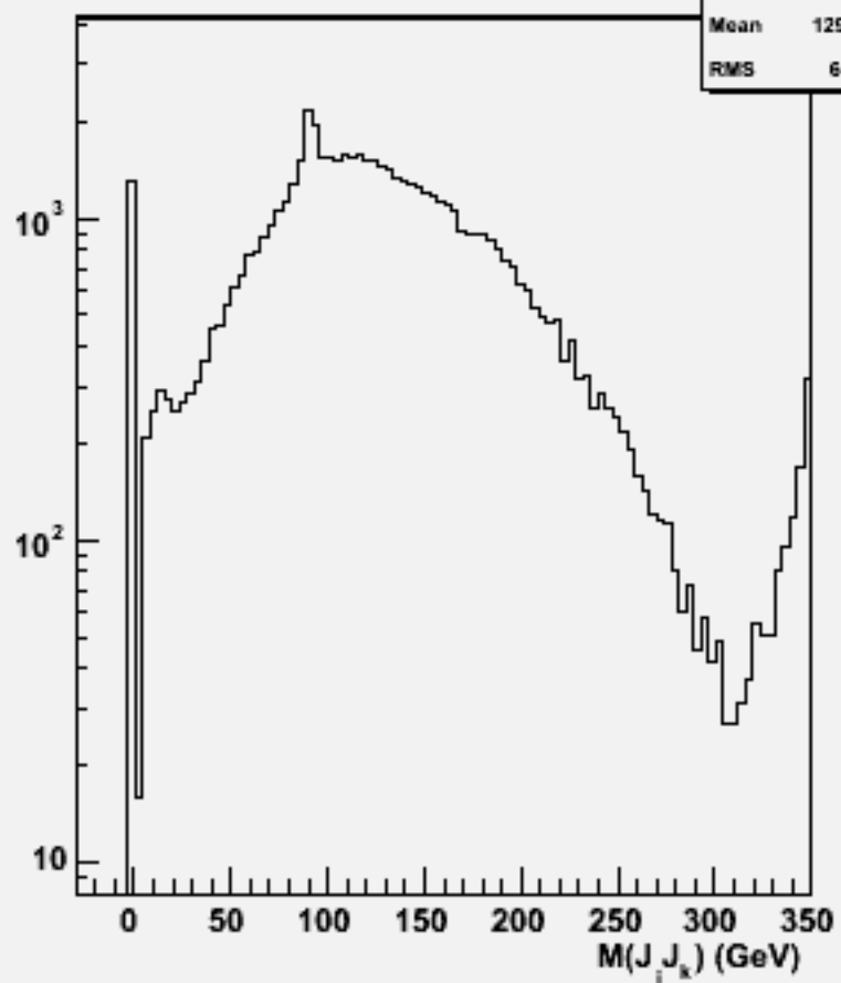
2jets mass(All comb)w102369 uue2e2bb_o
