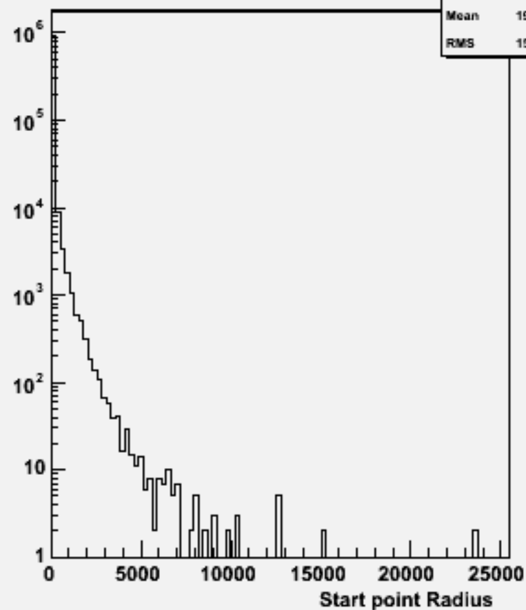
Start point R : w102369 uue2e2bb_o
