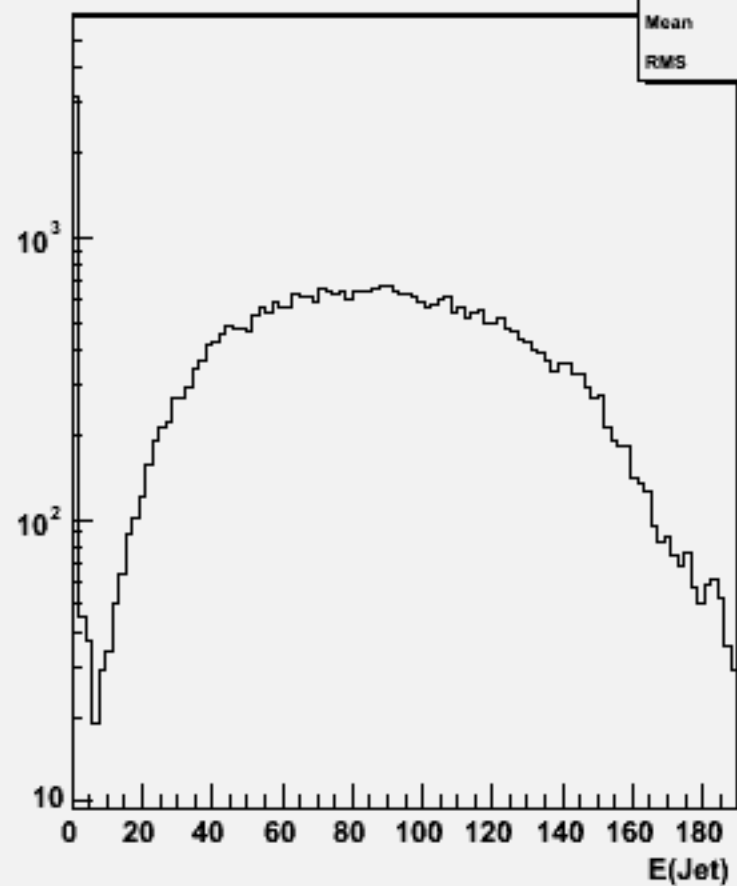
Jet energies(All jets)w102369 uue2e2bb_o
