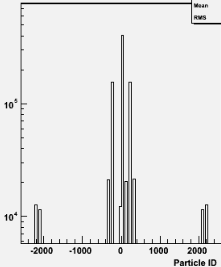
Particle ID : w102364 uue2e2ss_o
