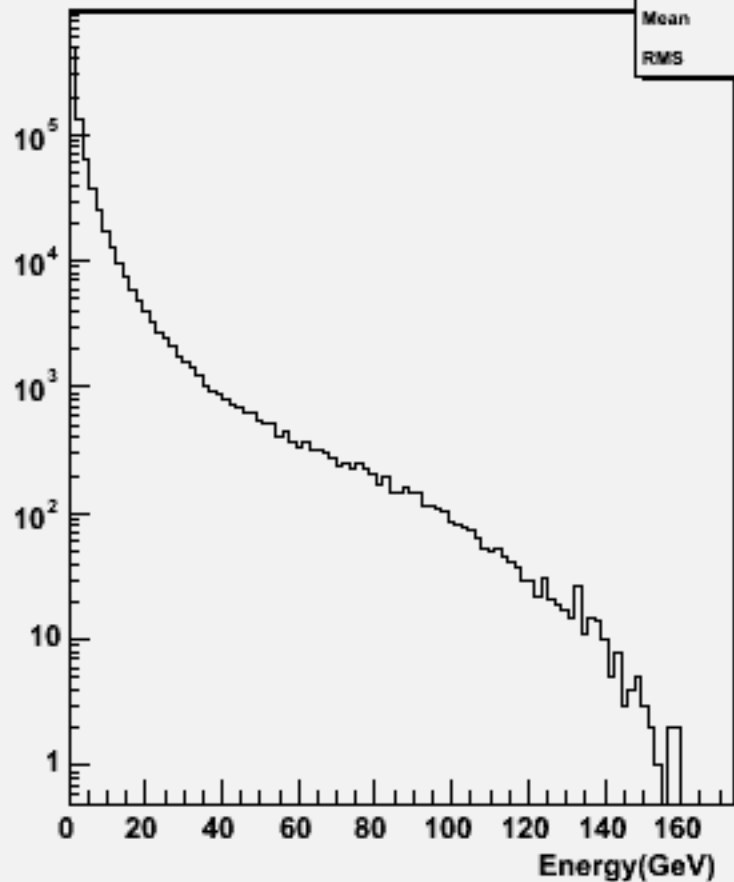
Particle Energy : w102364 uue2e2ss_o
