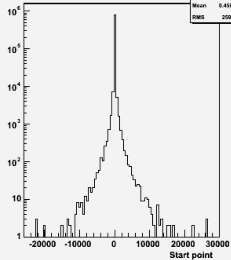
Start point Z : w102364 uue2e2ss_o
