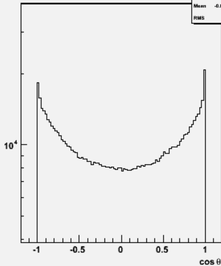
Particle cos \theta : w102364 uue2e2ss_o
