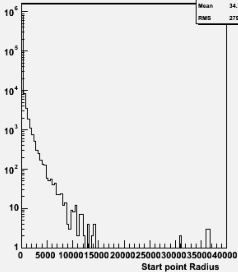
Start point R : w102364 uue2e2ss_o
