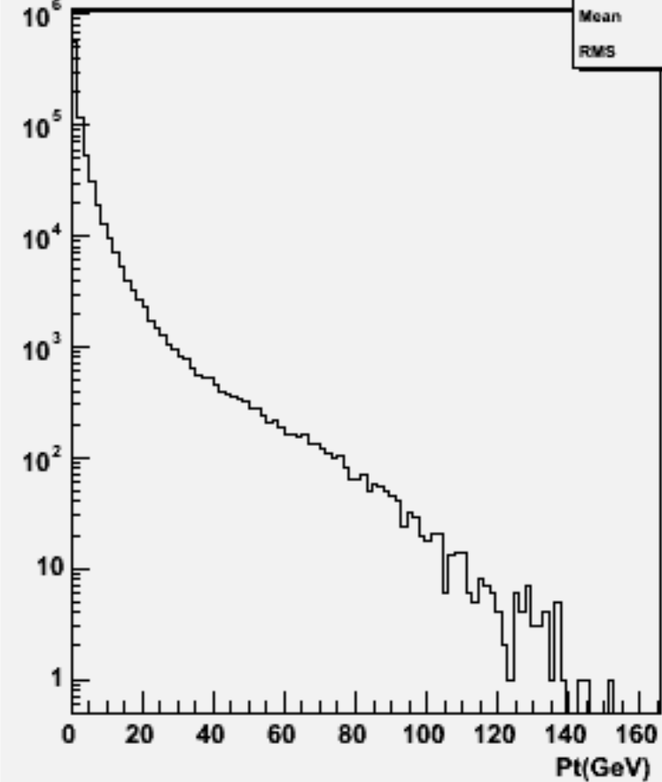
Particle Pt : w102364 uue2e2ss_o
