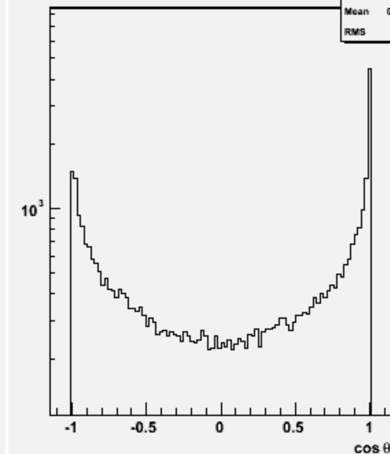
Jet cos \theta (All jets)w102361 uue2e2e3e3_o
