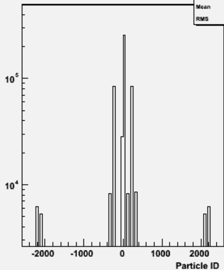
Particle ID : w102361 uue2e2e3e3_o
