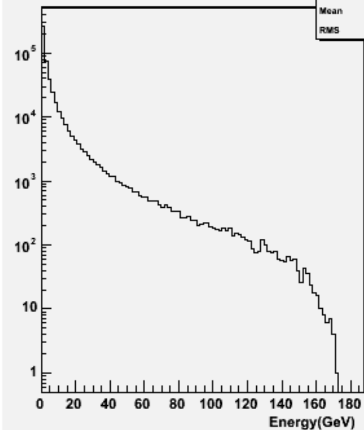
Particle Energy : w102361 uue2e2e3e3_o
