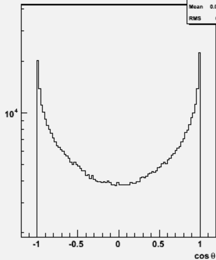
Particle cosθ : w102361 uue2e2e3e3_o
