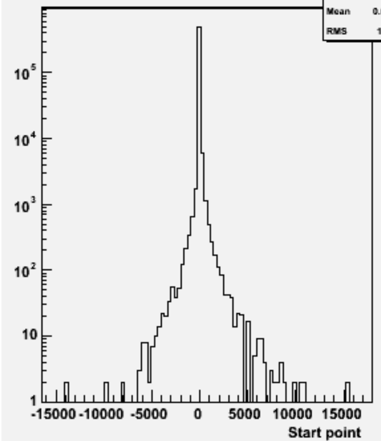
Start point Z : w102361 uue2e2e3e3_o
