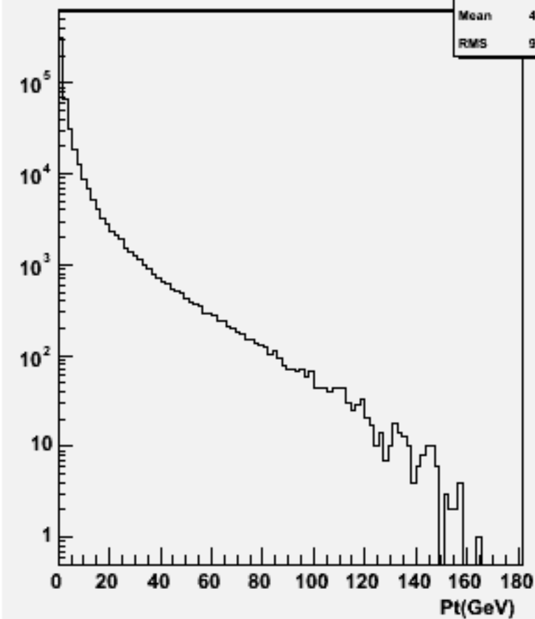
Particle Pt : w102361 uue2e2e3e3_o
