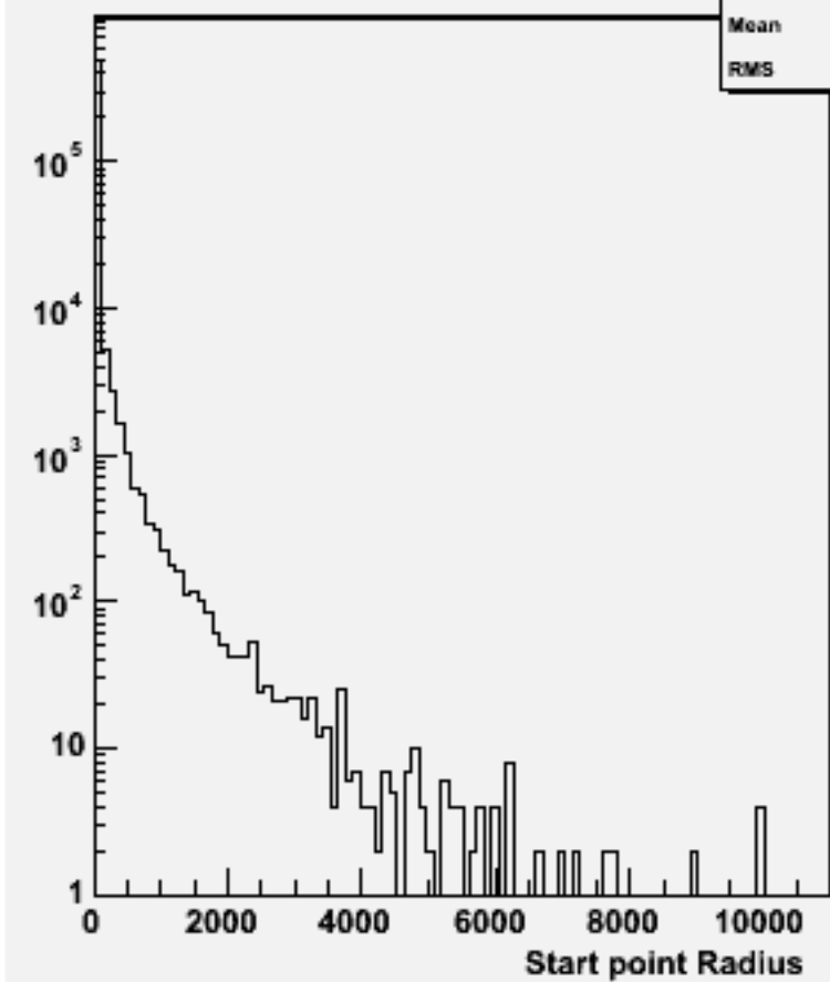
Start point R : w102361 uue2e2e3e3_o
