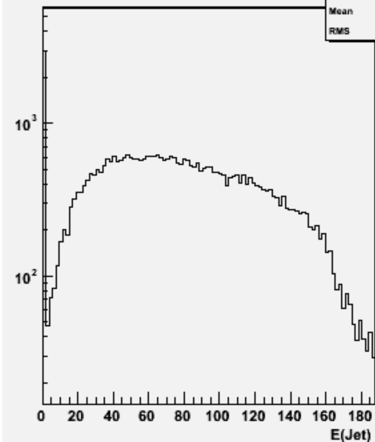
Jet energies(All jets)w102361 uue2e2e3e3_o
