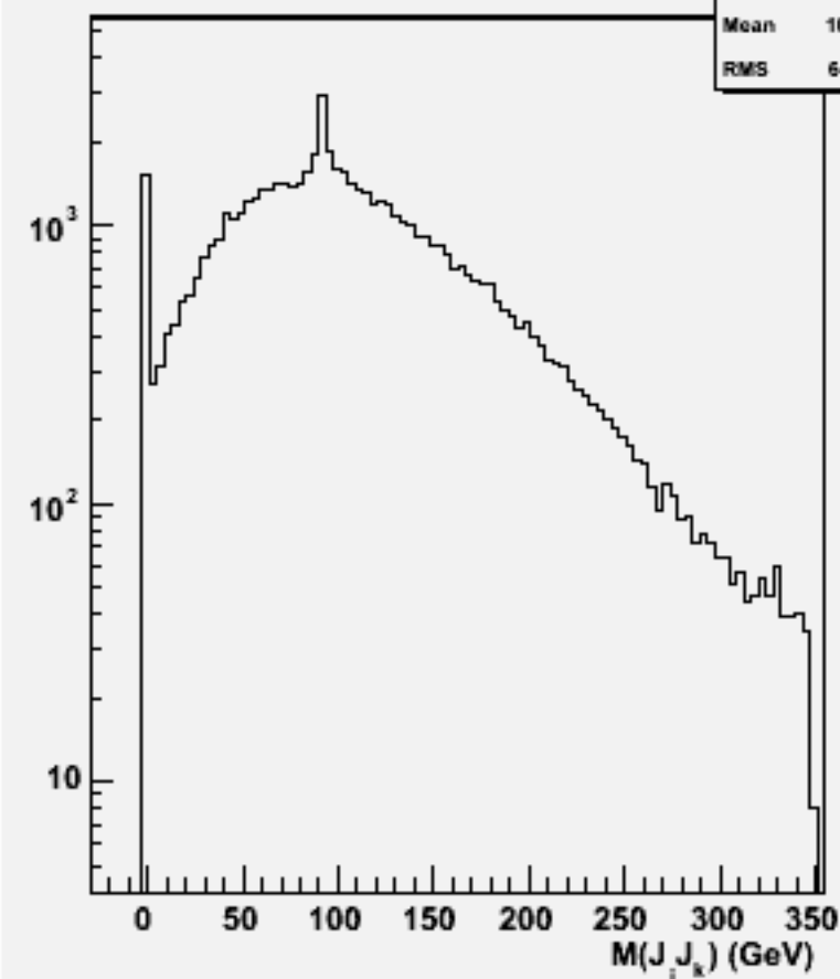
2jets mass(All comb)w102361 uue2e2e3e3_o
