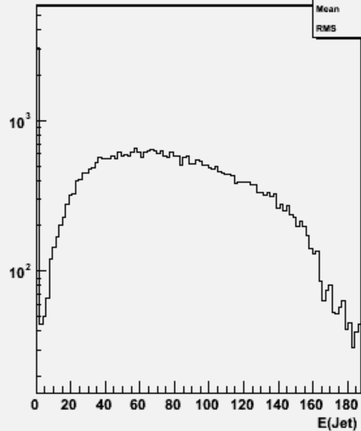
Jet energies(All jets)w102360 uue2e2e3e3_o
