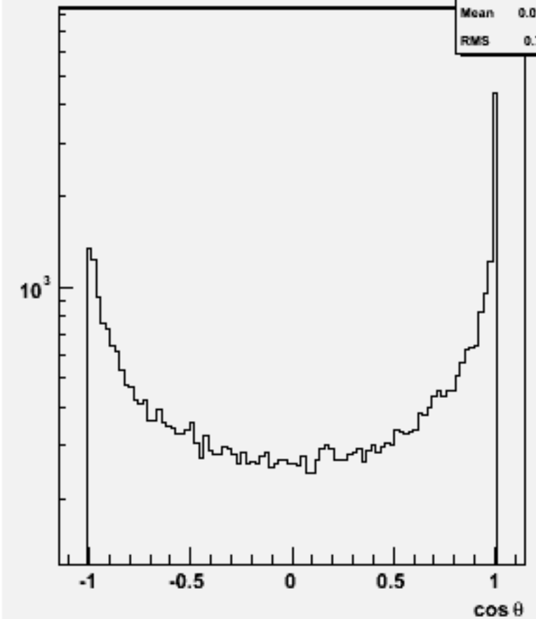
Jet cos \theta (All jets)w102360 uue2e2e3e3_o
