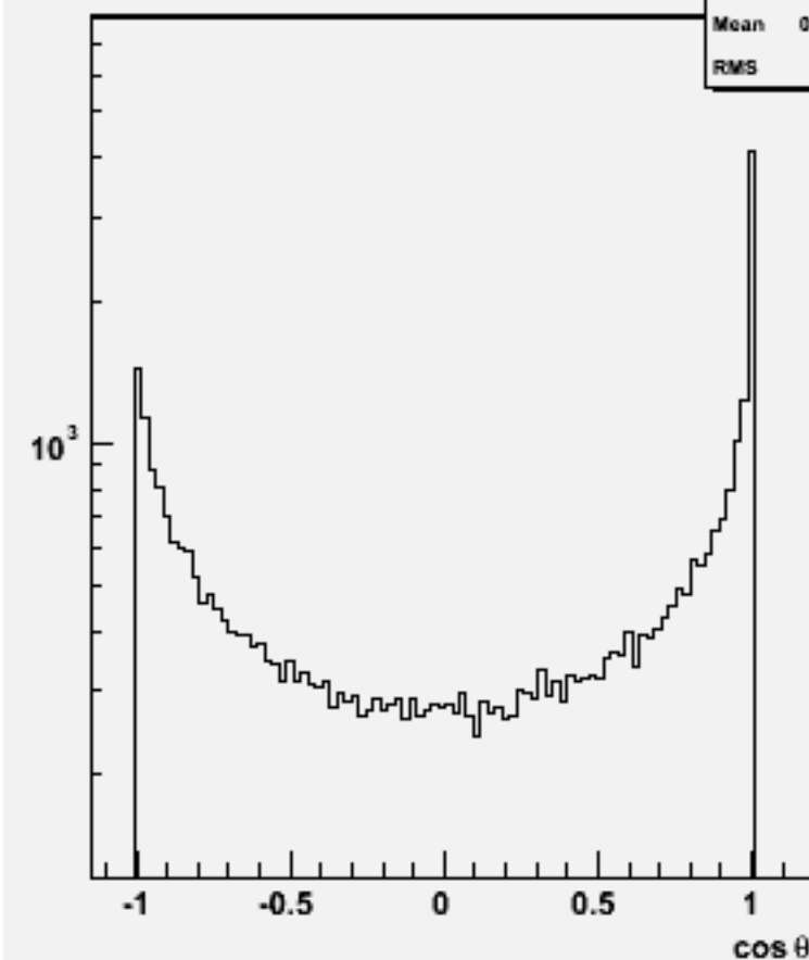
Jet cos \theta (All jets)w102356 uue2e2e2e2_o
