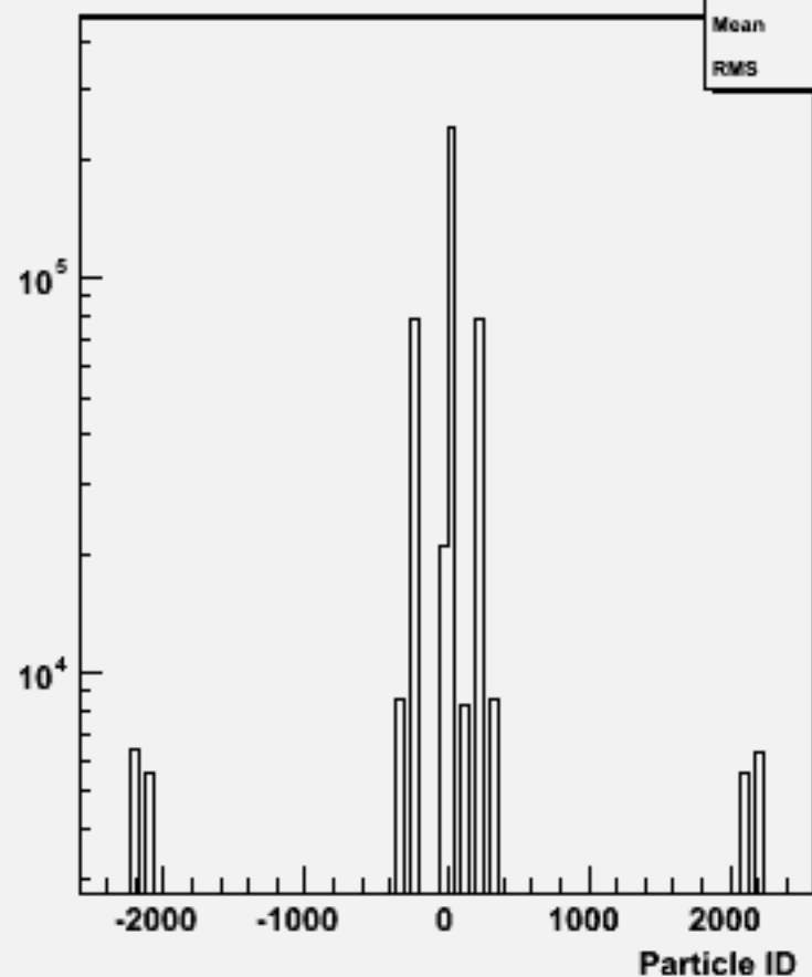
Particle ID : w102356 uue2e2e2e2_o
