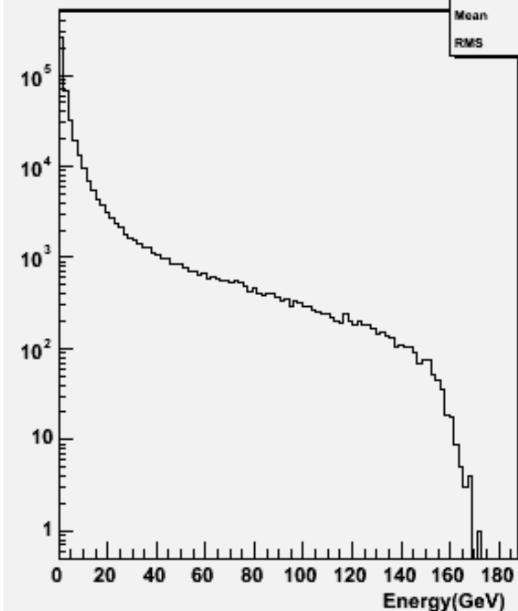
Particle Energy : w102356 uue2e2e2e2_o
