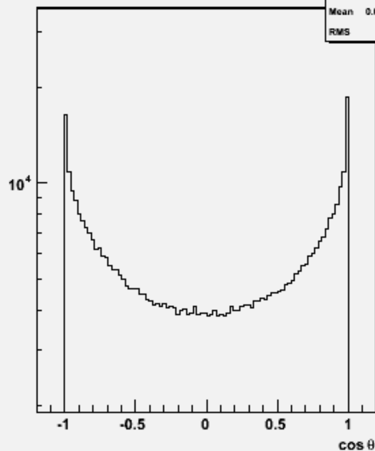
Particle cosθ : w102356 uue2e2e2e2_o
