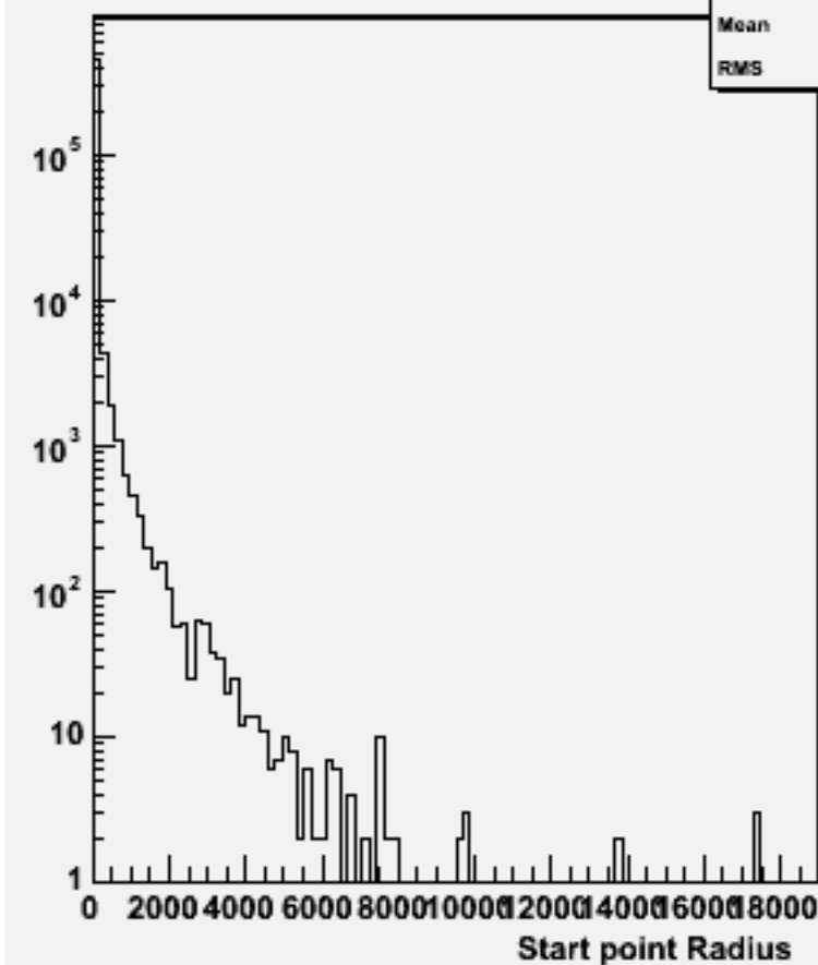
Start point R : w102356 uue2e2e2e2_o
