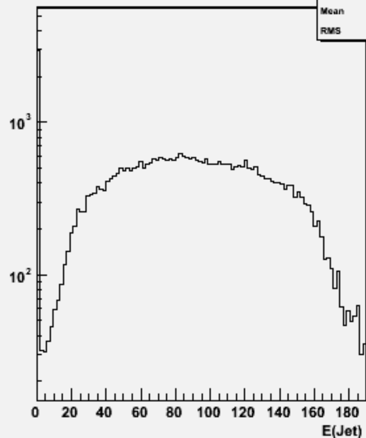
Jet energies(All jets)w102356 uue2e2e2e2_o
