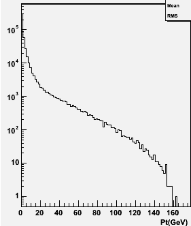
Particle Pt : w102356 uue2e2e2e2_o
