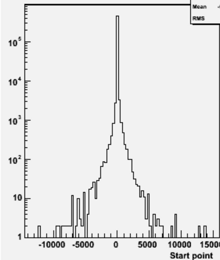
Start point Z : w102356 uue2e2e2e2_o
