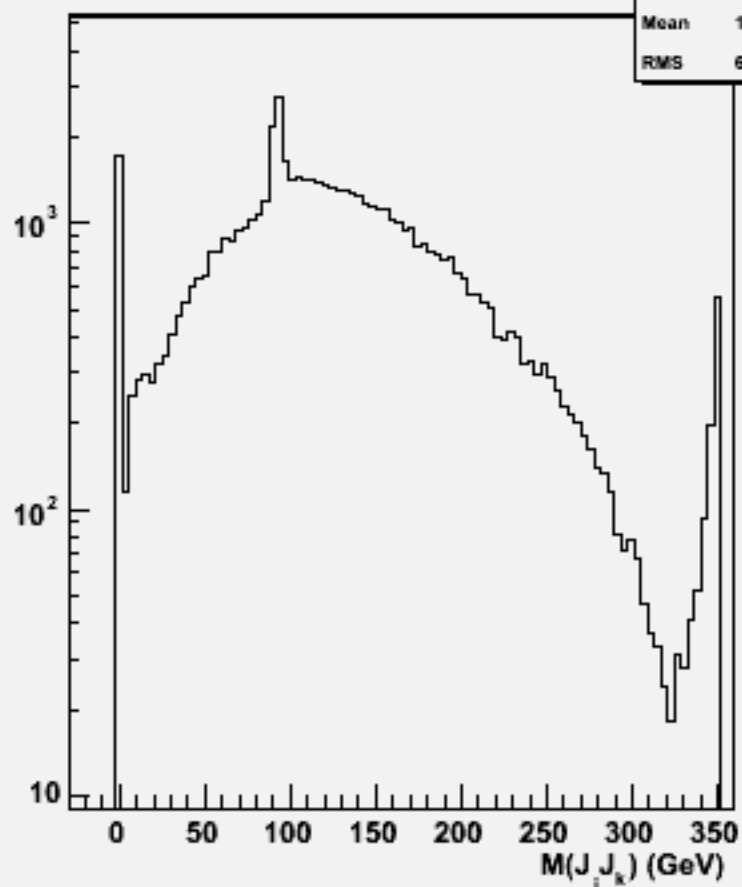
2jets mass(All comb)w102356 uue2e2e2e2_o
