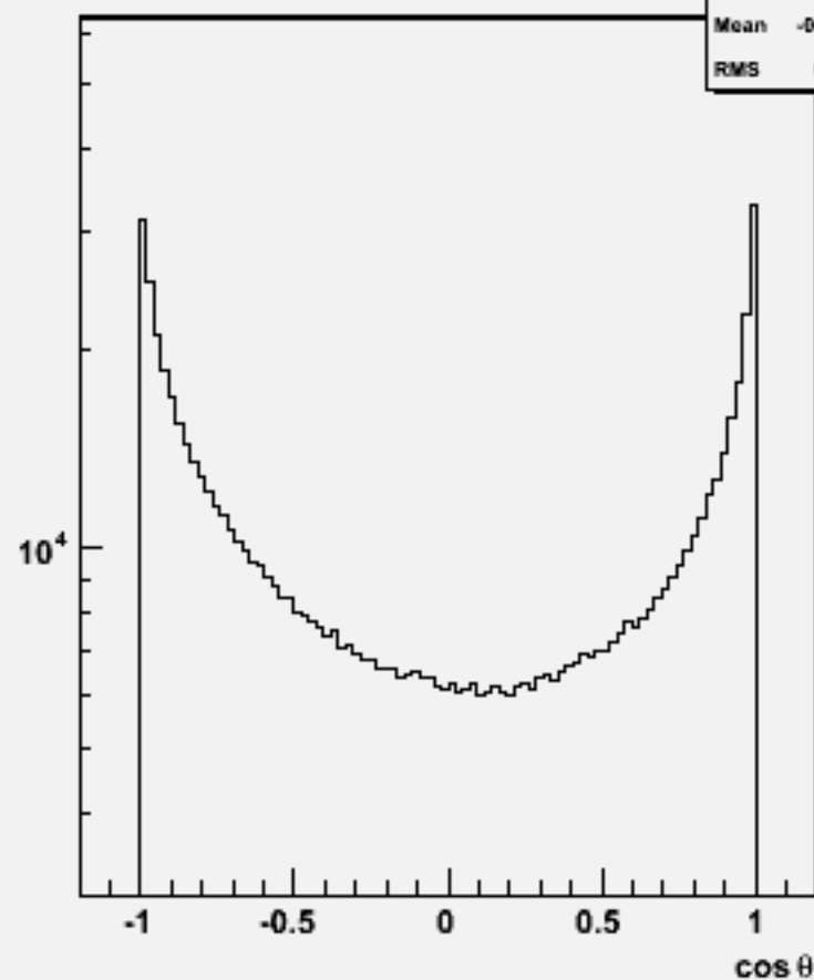
Particle cos \theta : w102354 uue1e1bb_o
