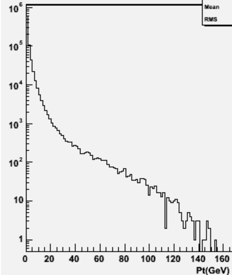
Particle Pt : w102354 uue1e1bb_o
