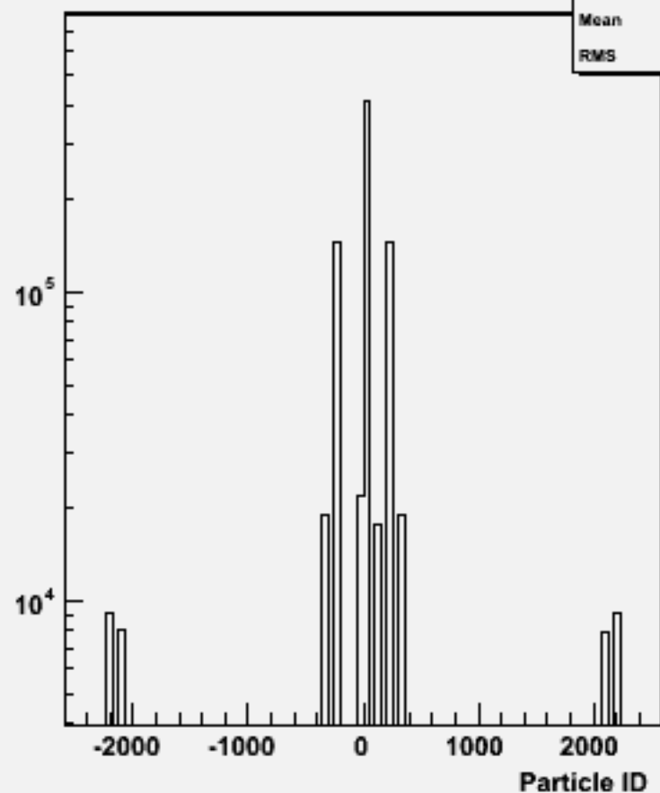
Particle ID : w102354 uue1e1bb_o
