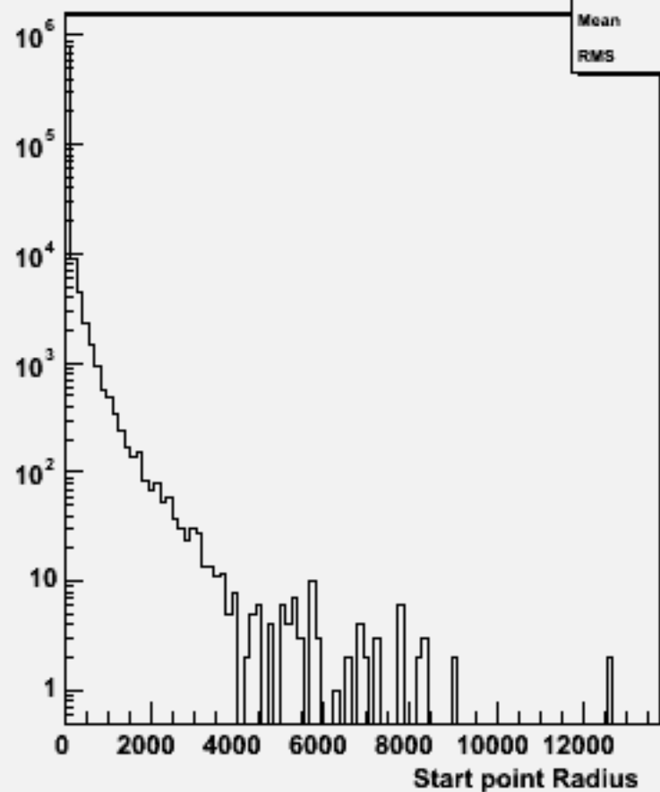
Start point R : w102354 uue1e1bb_o
