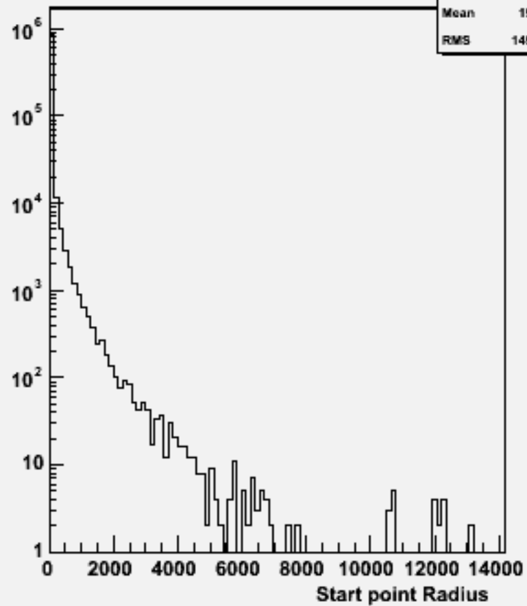
Start point R : w102353 uue1e1bb_o
