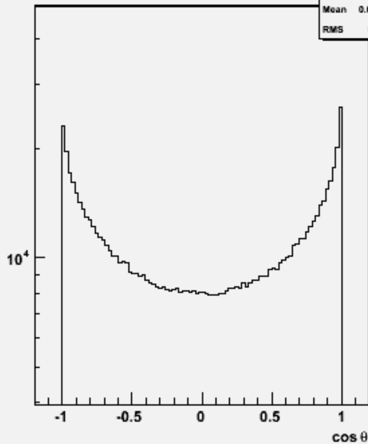
Particle cos \theta : w102353 uue1e1bb_o
