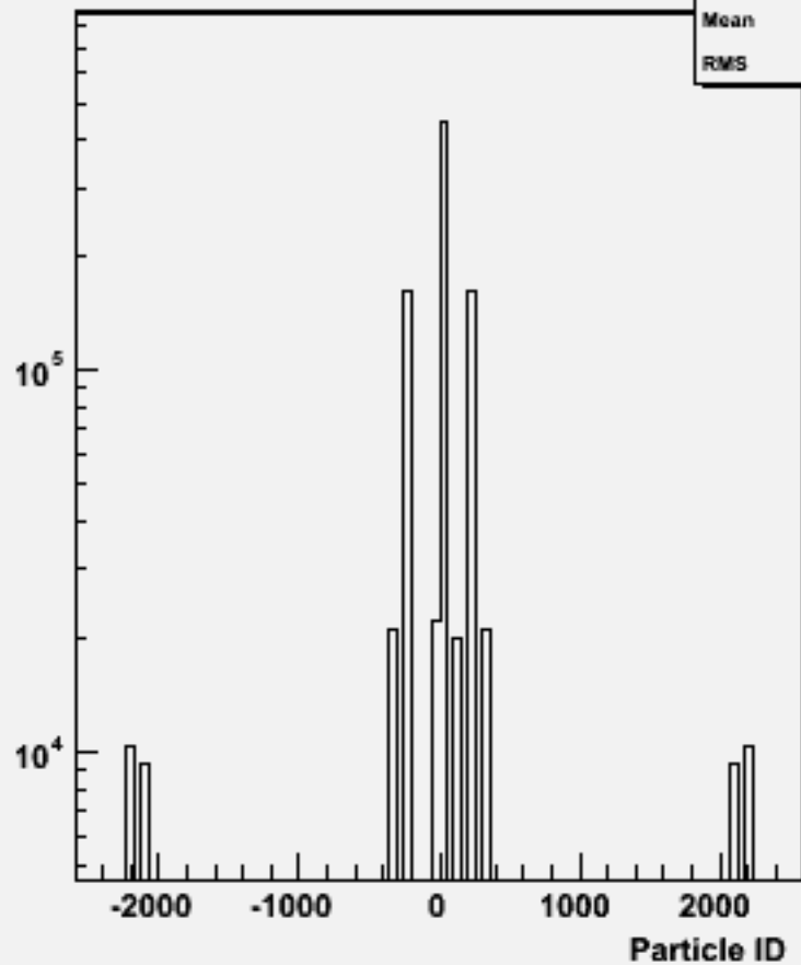
Particle ID : w102353 uue1e1bb_o
