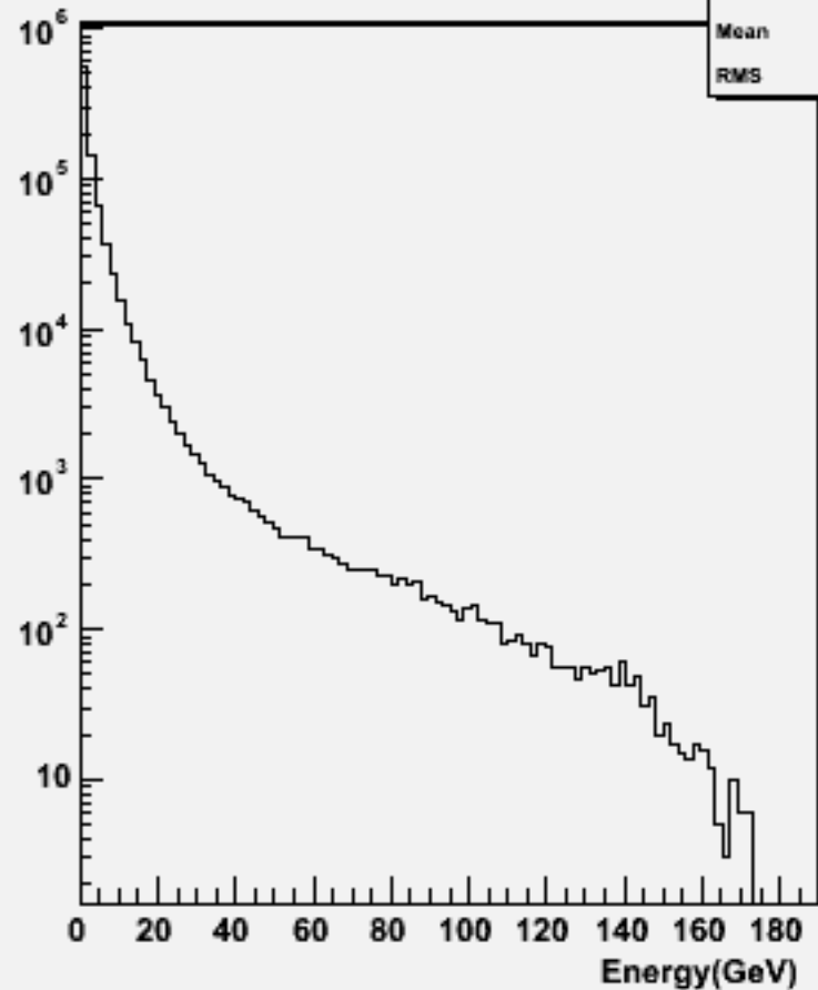
Particle Energy : w102353 uue1e1bb_o
