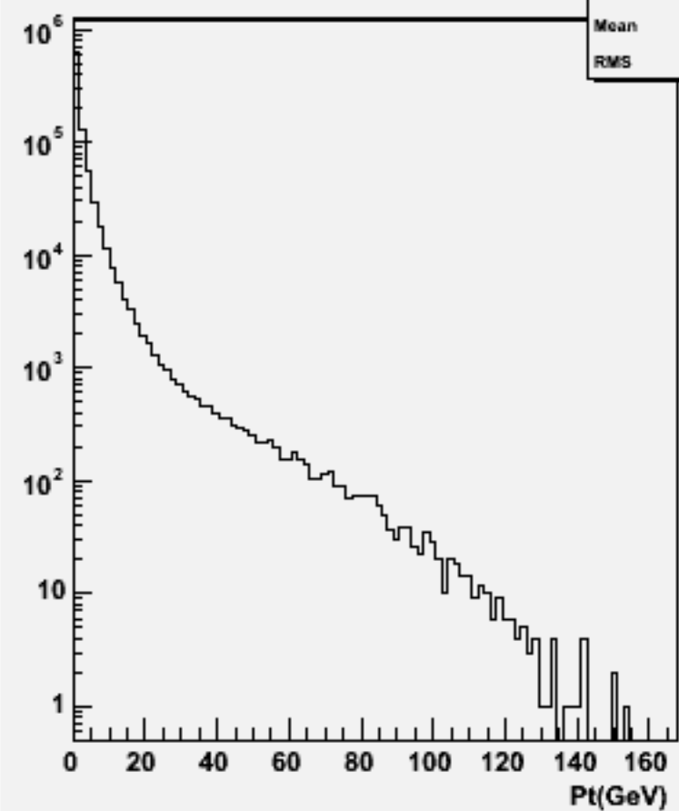
Particle Pt : w102353 uue1e1bb_o
