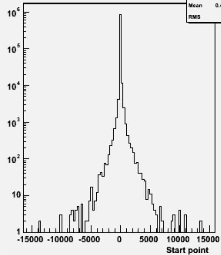
Start point Z : w102353 uue1e1bb_o
