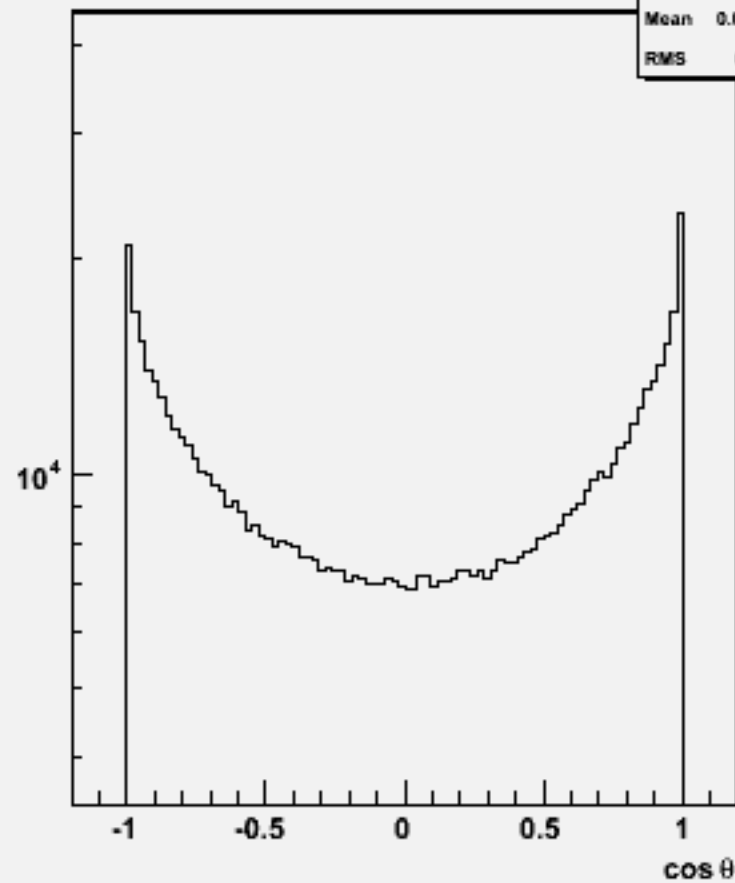
Particle cos \theta : w102349 uue1e1ss_o
