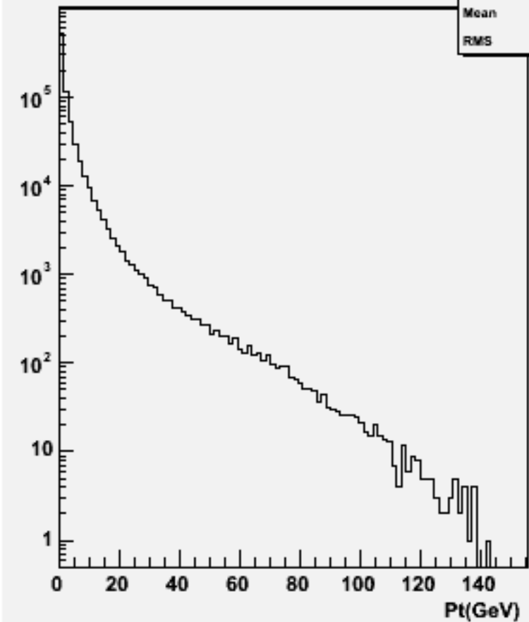
Particle Pt : w102349 uue1e1ss_o
