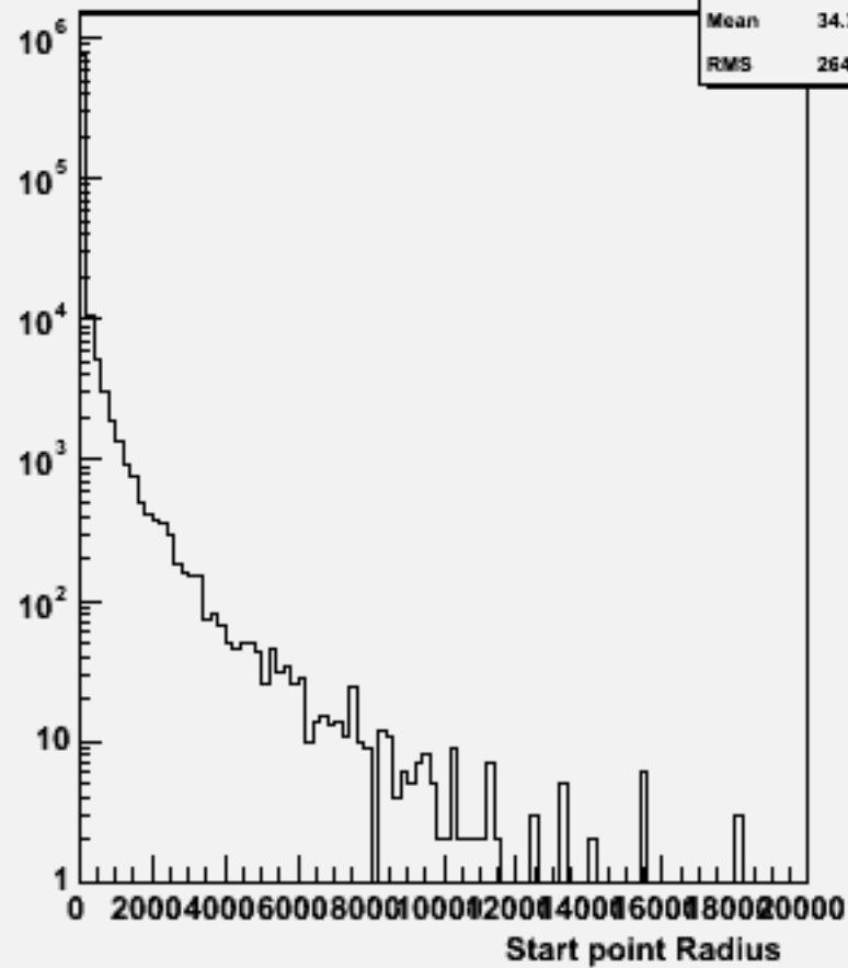
Start point R : w102349 uue1e1ss_o
