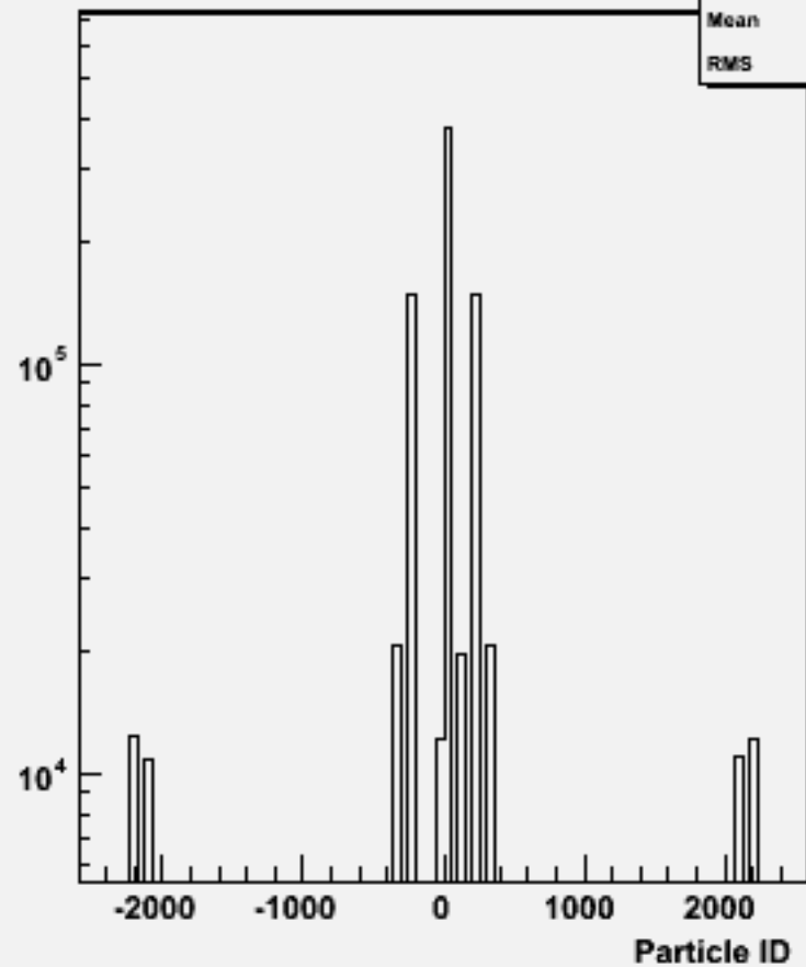
Particle ID : w102349 uue1e1ss_o
