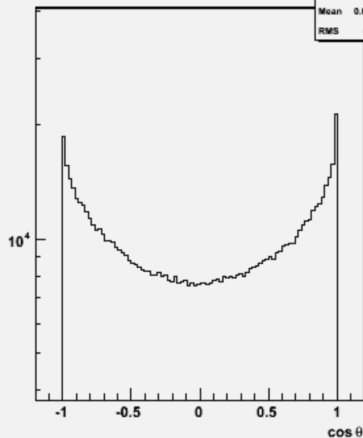
Particle cos \theta : w102348 uue1e1ss_o
