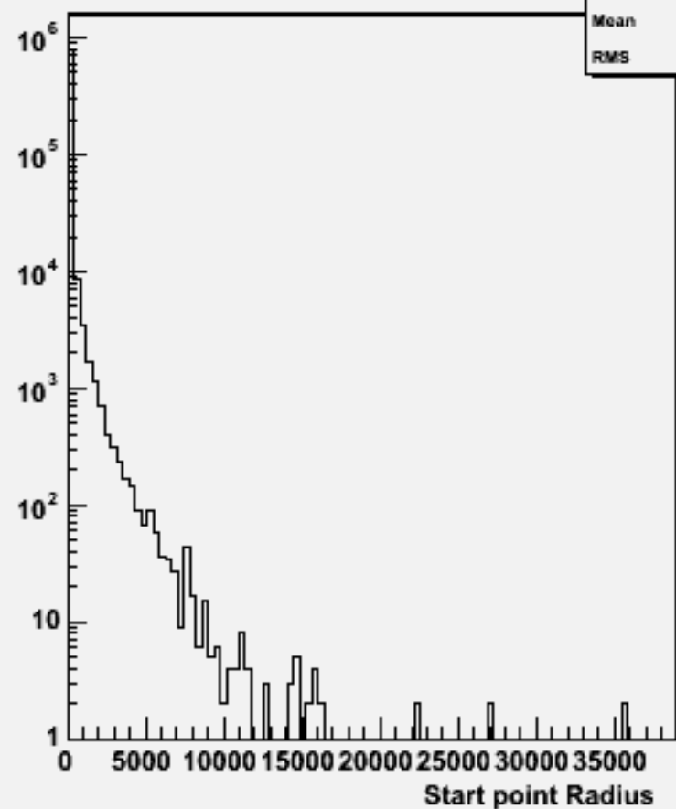
Start point R : w102348 uue1e1ss_o
