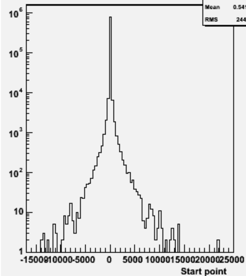
Start point Z : w102348 uue1e1ss_o
