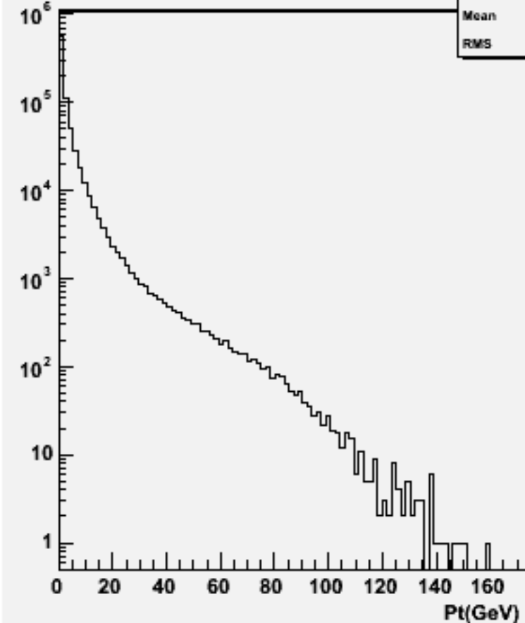
Particle Pt : w102348 uue1e1ss_o
