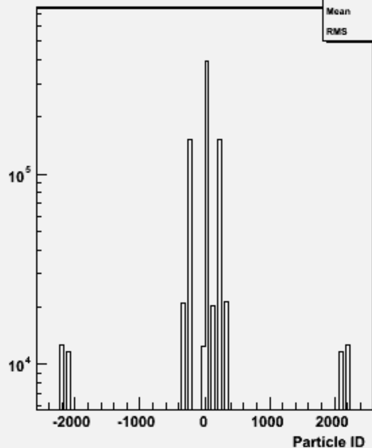
Particle ID : w102348 uue1e1ss_o
