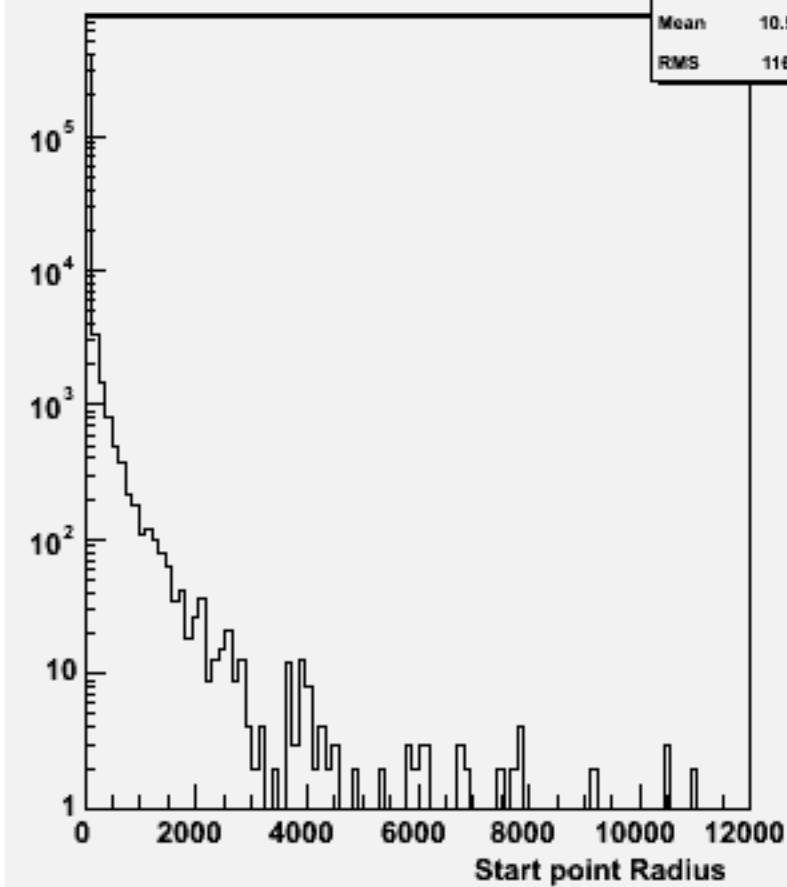
Start point R : w102345 uue1e1e3e3_o
