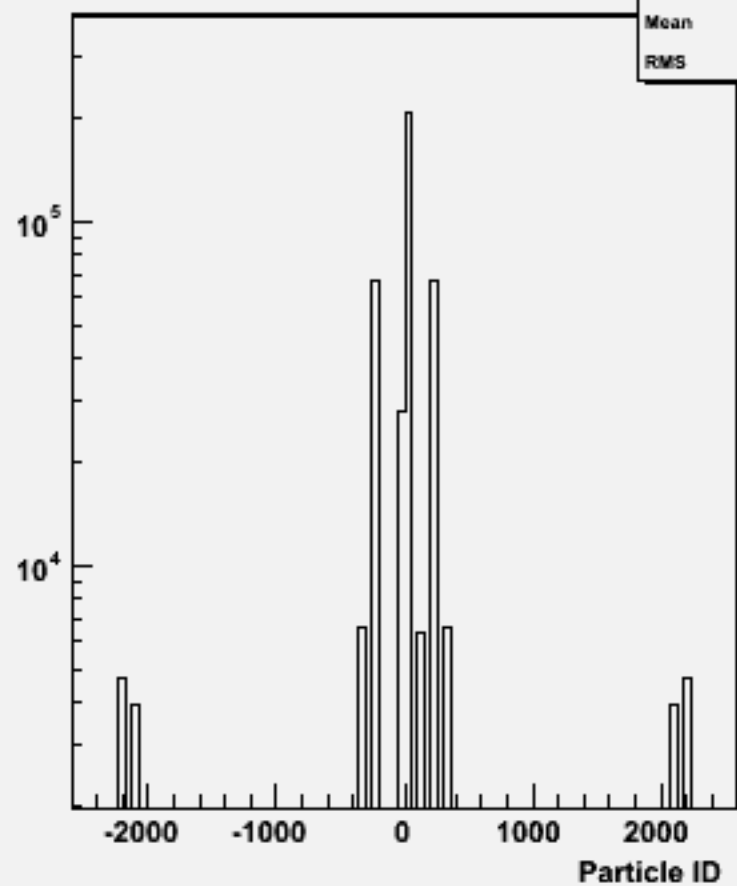
Particle ID : w102345 uue1e1e3e3_o
