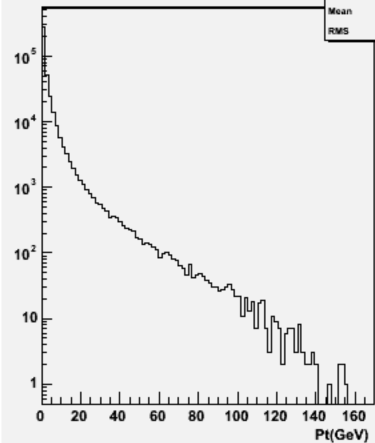
Particle Pt : w102345 uue1e1e3e3_o
