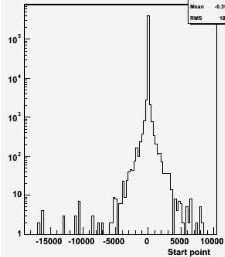
Start point Z : w102345 uue1e1e3e3_o
