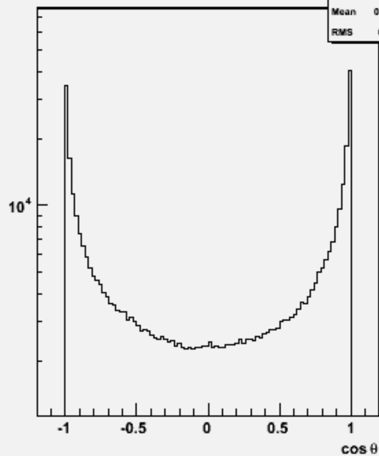
Particle \cos\theta : w102345 uue1e1e3e3_o
