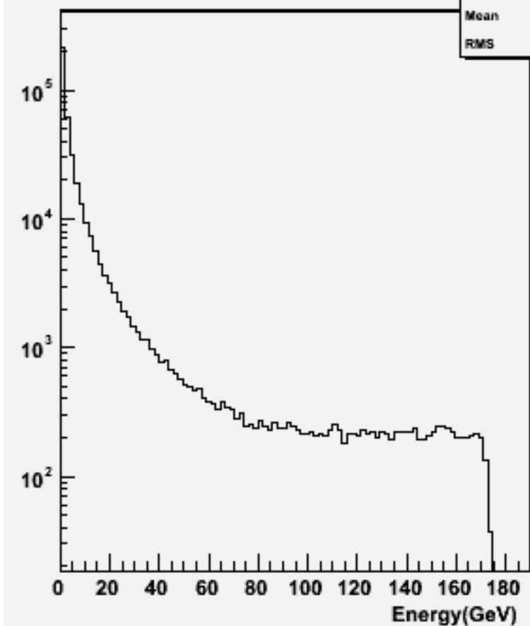
Particle Energy : w102345 uue1e1e3e3_o
