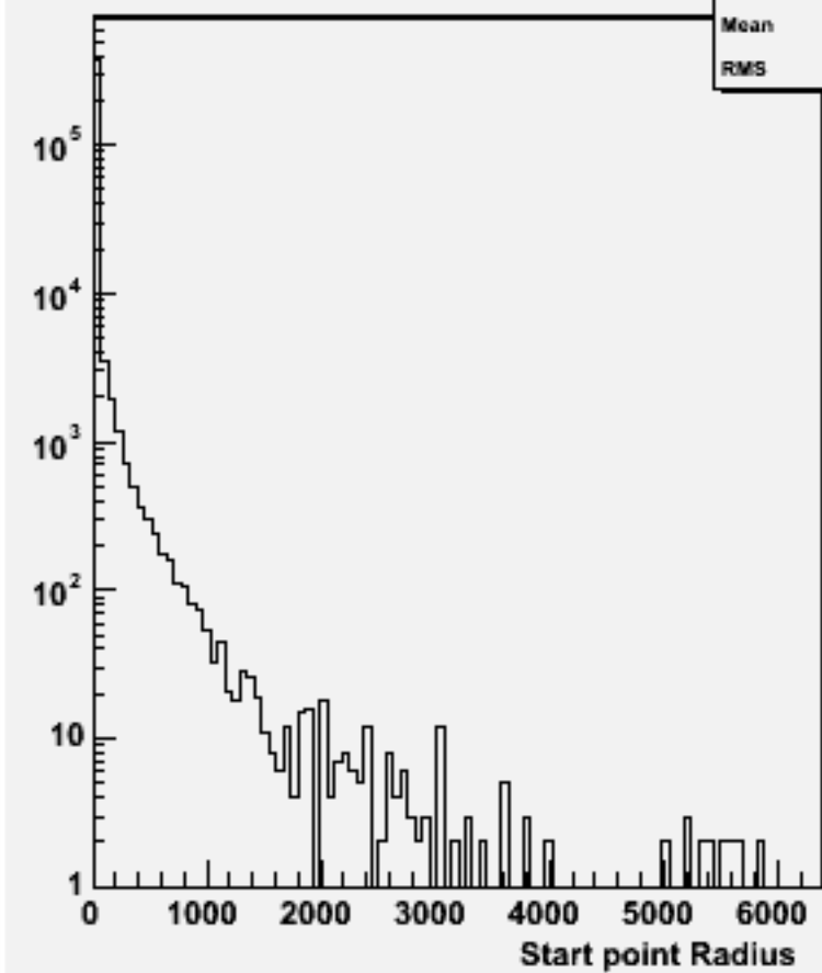
Start point R : w102343 uue1e1e3e3_o
