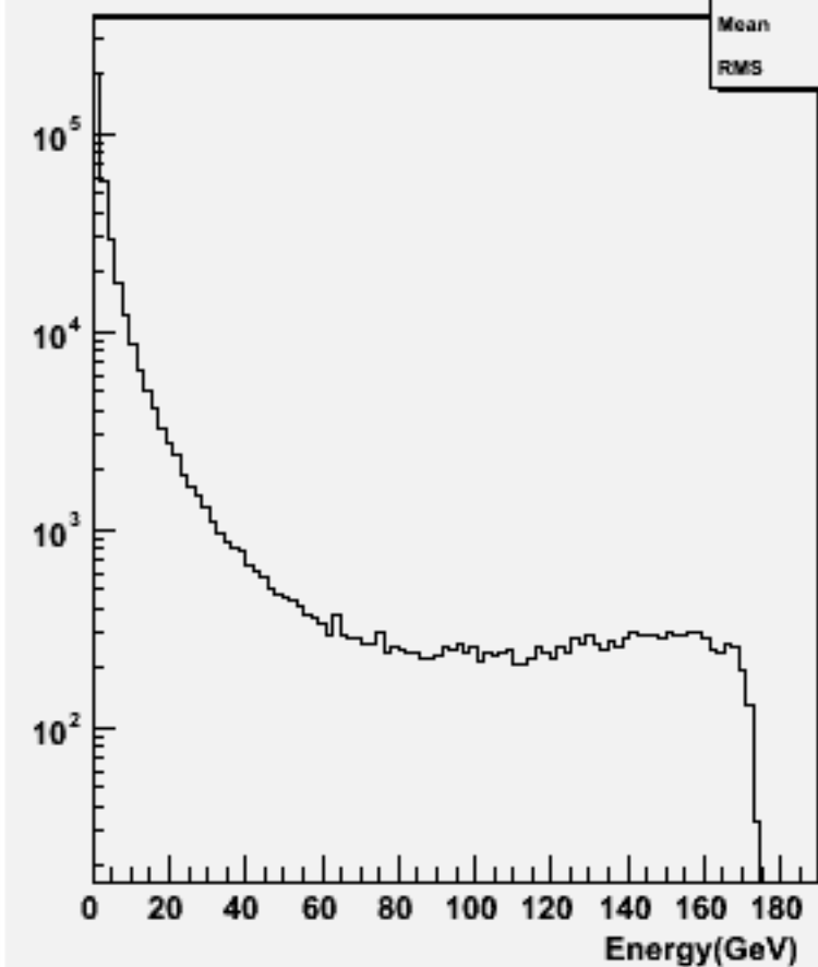
Particle Energy : w102343 uue1e1e3e3_o
