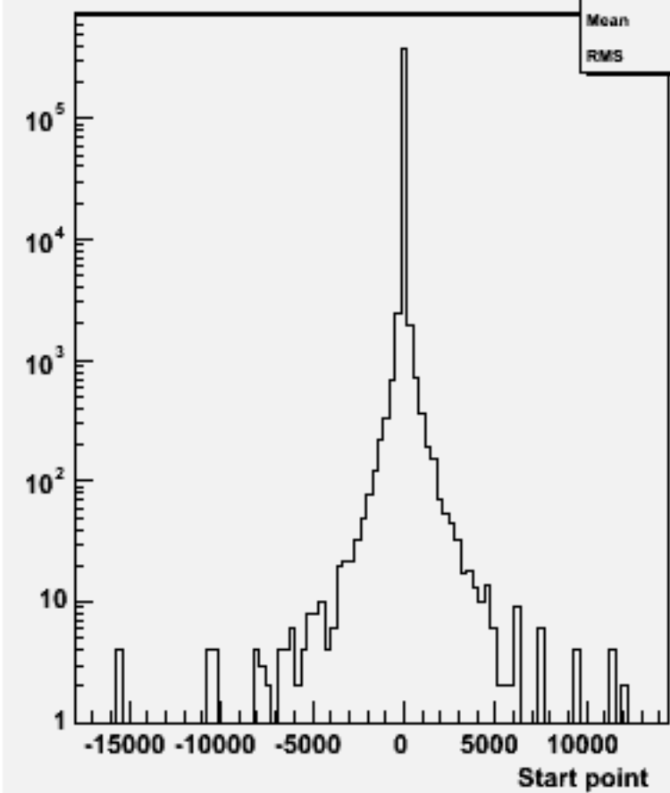
Start point Z : w102343 uue1e1e3e3_o
