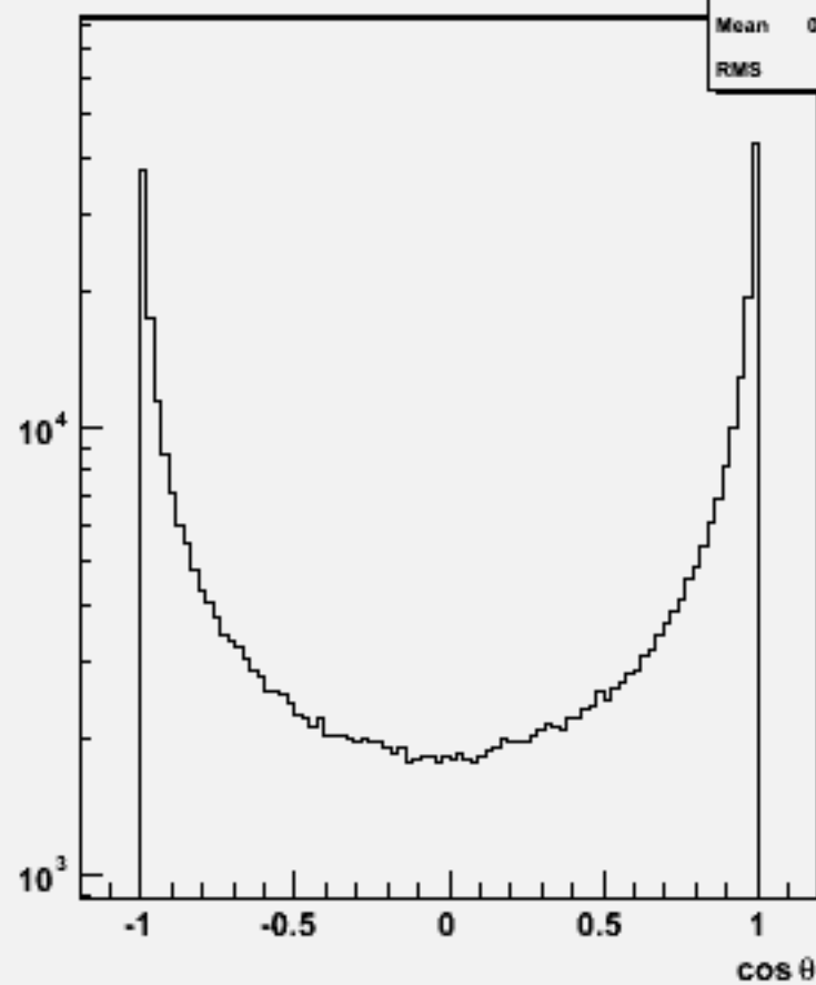
Particle \cos\theta : w102343 uue1e1e3e3_o
