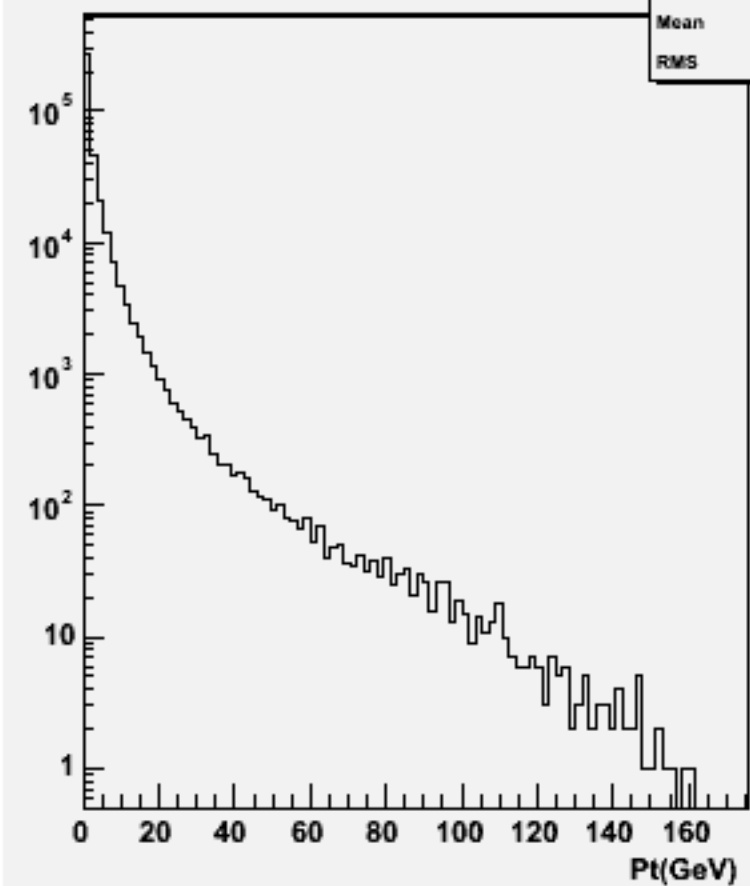
Particle Pt : w102343 uue1e1e3e3_o
