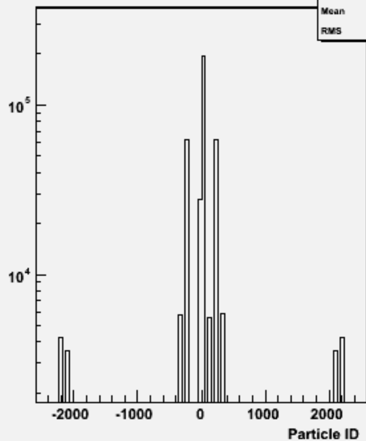
Particle ID : w102343 uue1e1e3e3_o
