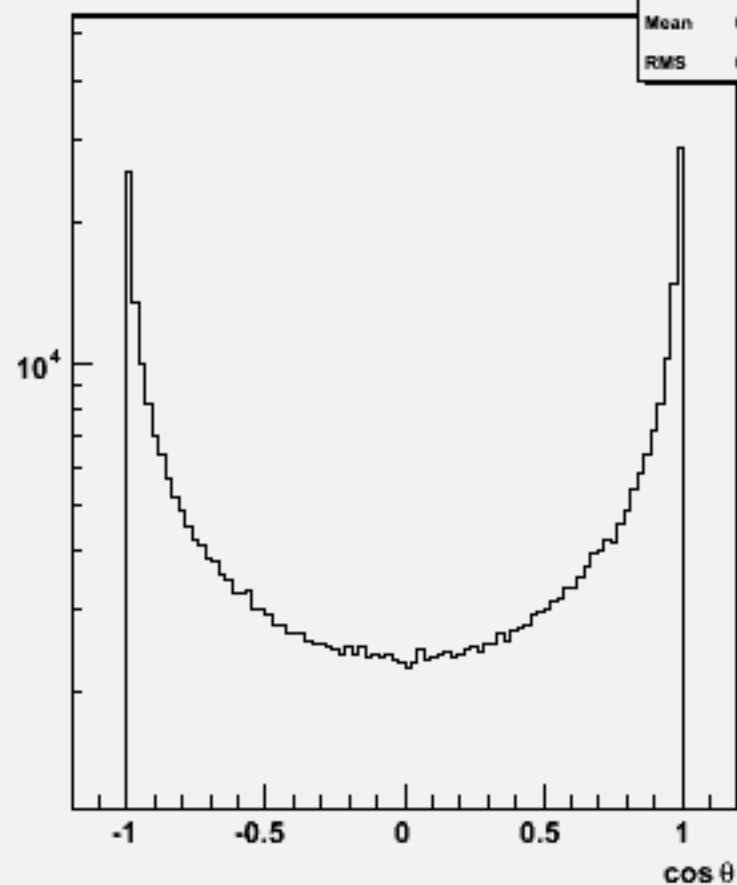
Particle cosθ : w102341 uue1e1e2e2_o
