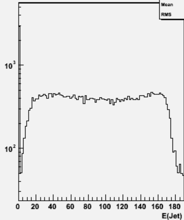
Jet energies(All jets)w102341 uue1e1e2e2_o
