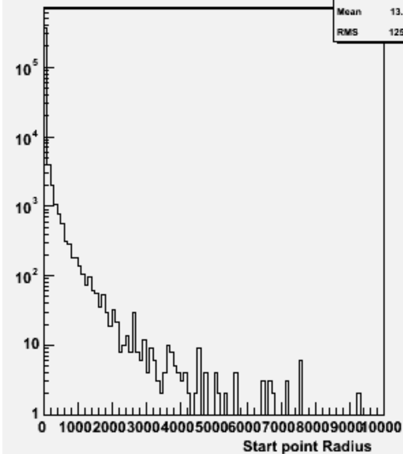
Start point R : w102341 uue1e1e2e2_o
