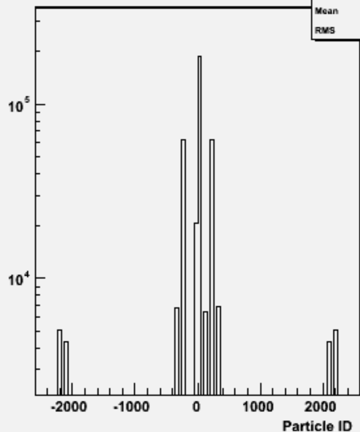
Particle ID : w102341 uue1e1e2e2_o
