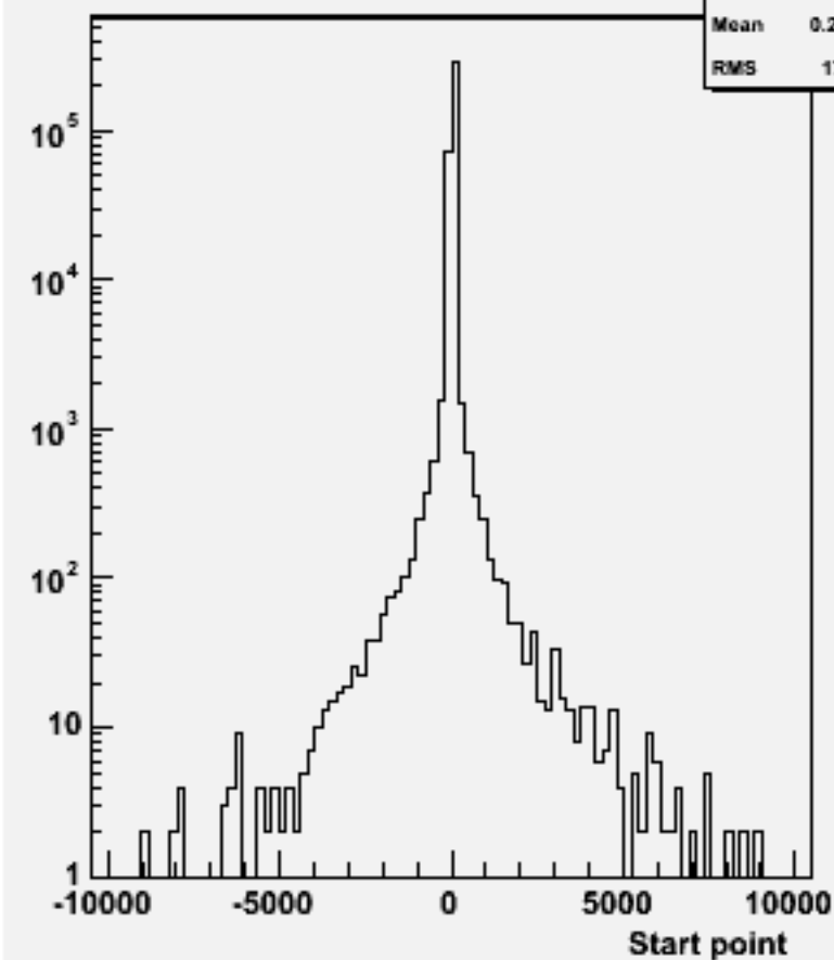
Start point Z : w102341 uue1e1e2e2_o
