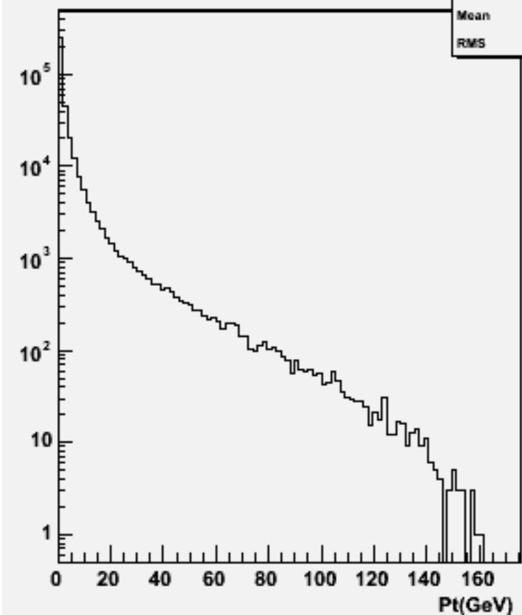
Particle Pt : w102341 uue1e1e2e2_o
