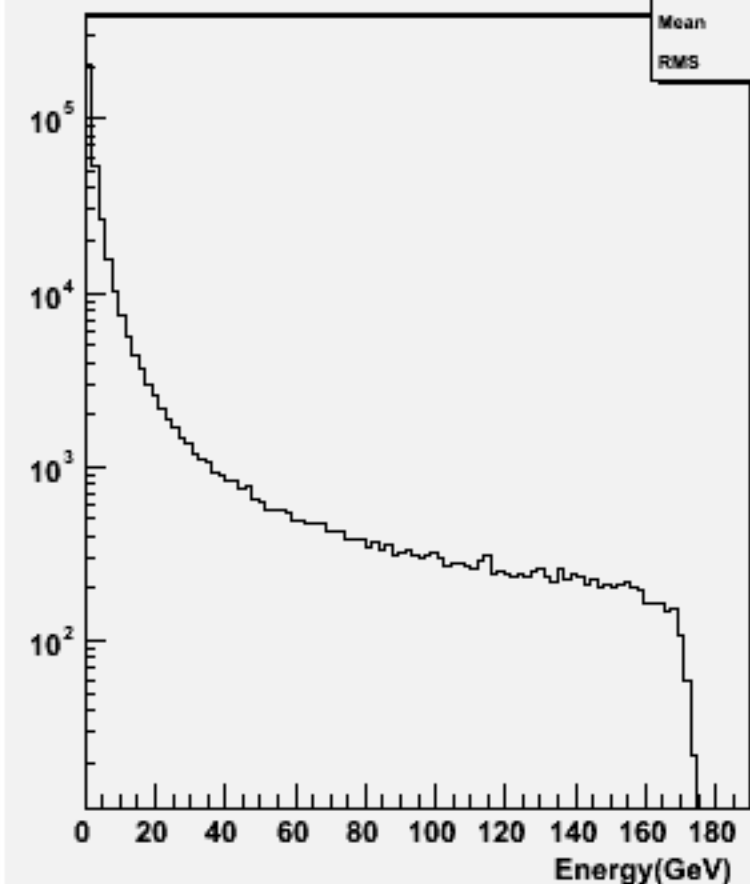
Particle Energy : w102341 uue1e1e2e2_o
