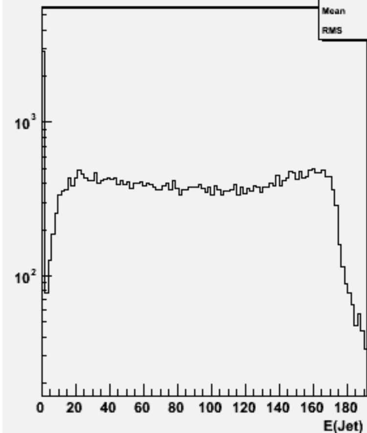
Jet energies(All jets)w102340 uue1e1e2e2_o
