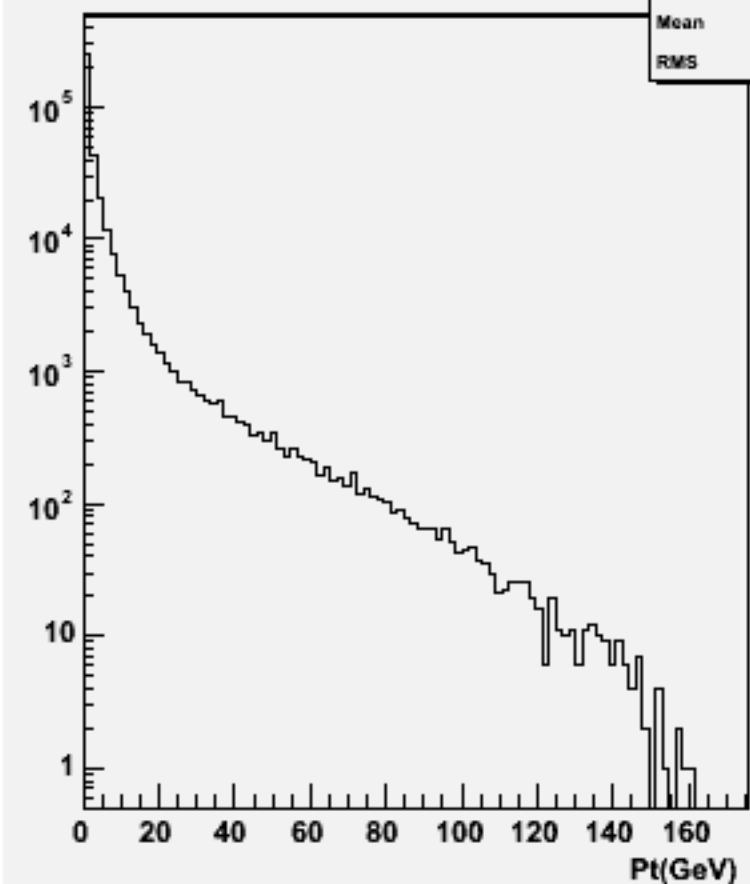
Particle Pt : w102340 uue1e1e2e2_o
