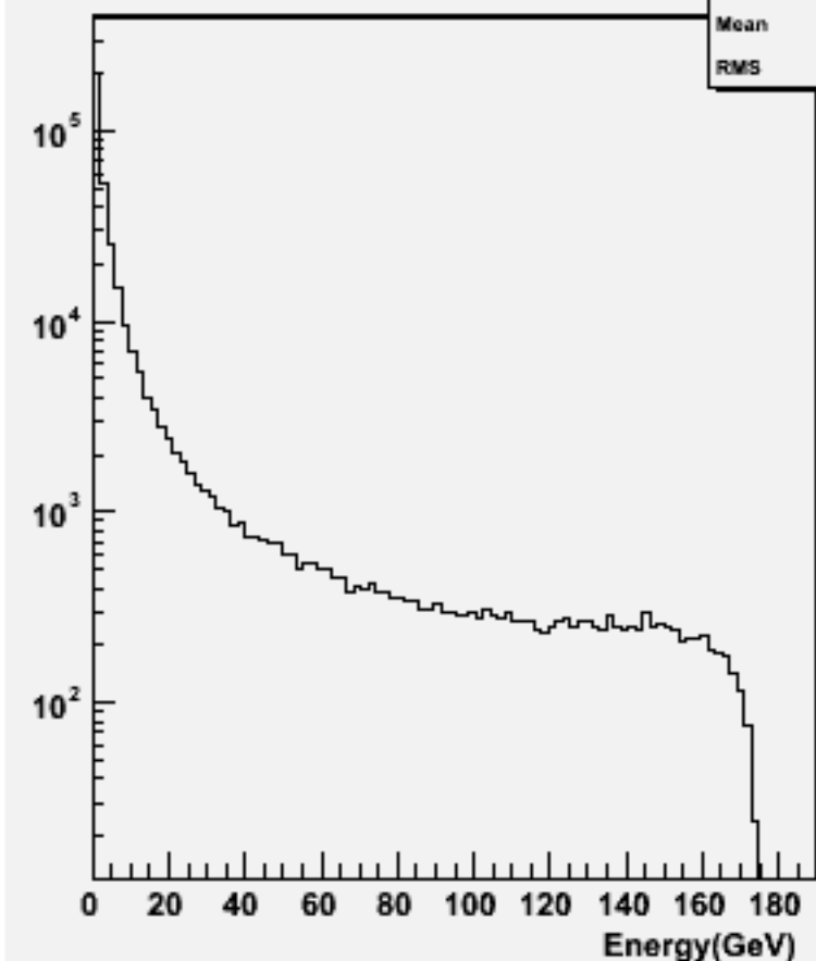
Particle Energy : w102340 uue1e1e2e2_o
