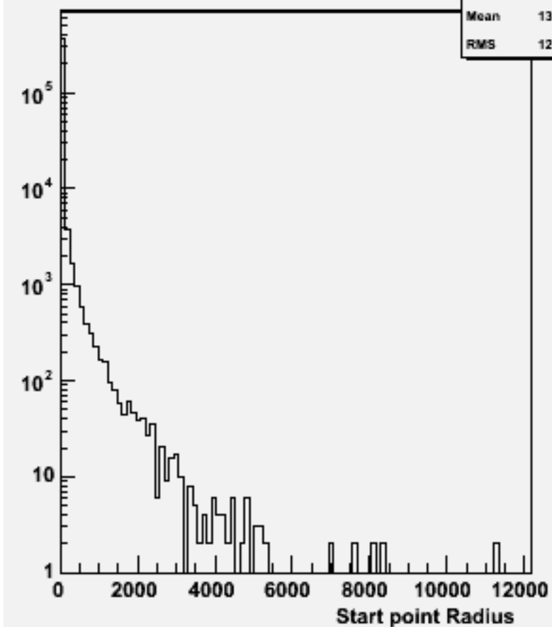
Start point R : w102340 uue1e1e2e2_o
