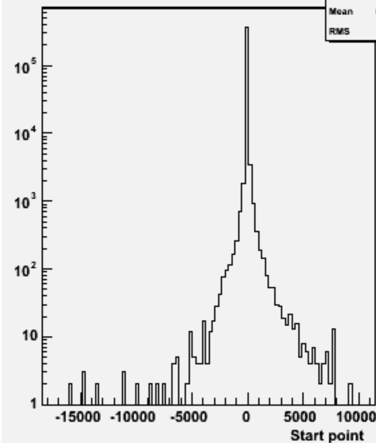
Start point Z : w102340 uue1e1e2e2_o
