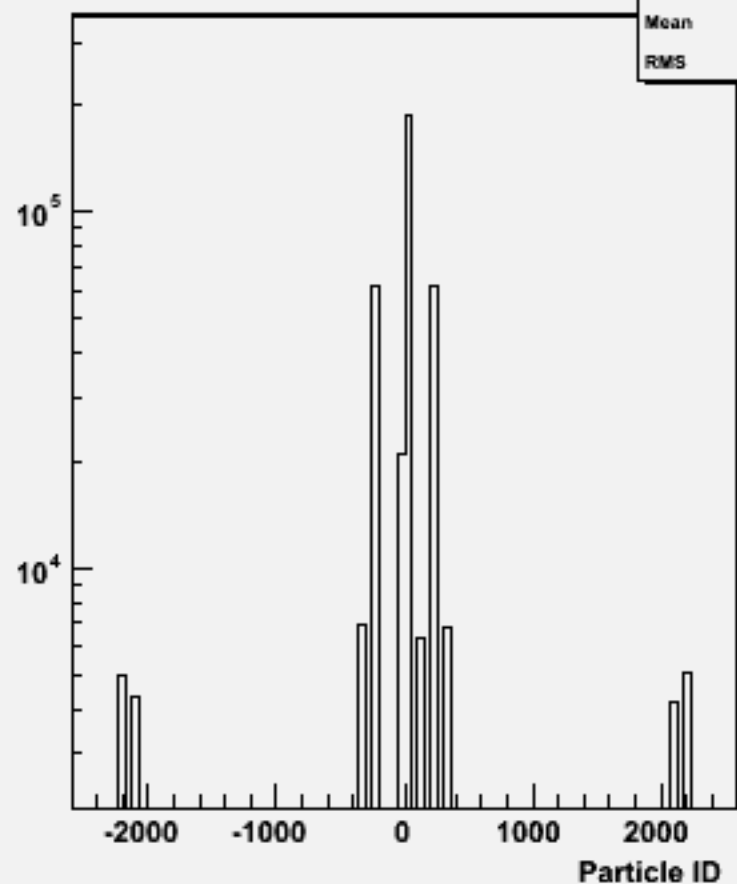
Particle ID : w102340 uue1e1e2e2_o
