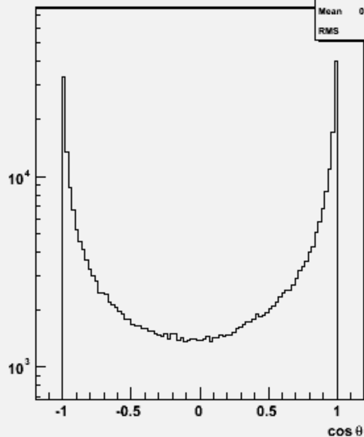
Particle cosθ : w102339 uue1e1e2e2_o
