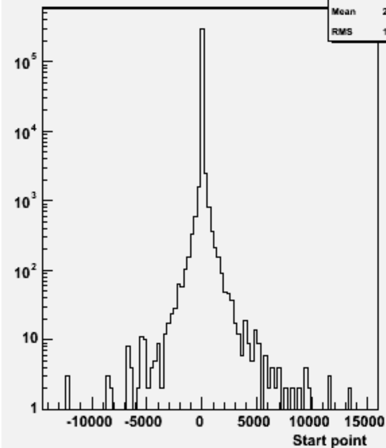
Start point Z : w102339 uue1e1e2e2_o
