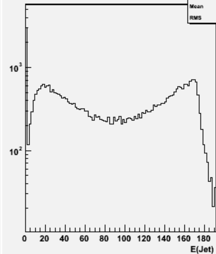
Jet energies(All jets)w102339 uue1e1e2e2_o
