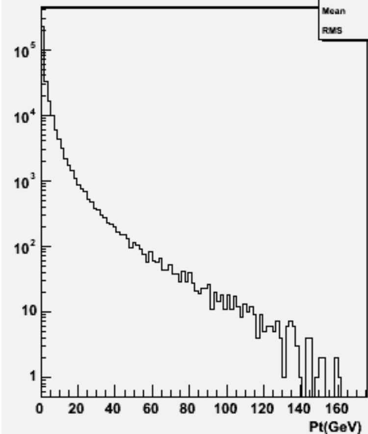
Particle Pt : w102339 uue1e1e2e2_o
