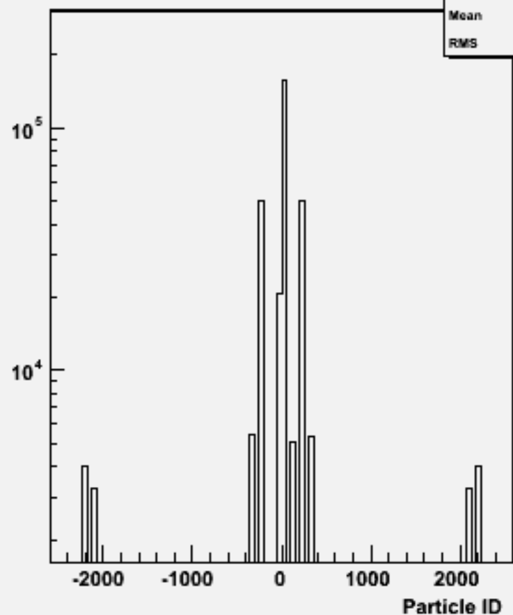
Particle ID : w102339 uue1e1e2e2_o
