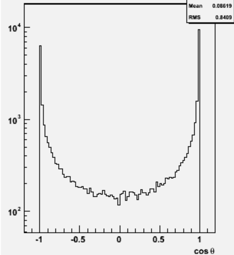
Jet cos \theta (All jets)w102336 uue1e1e1e1_o
