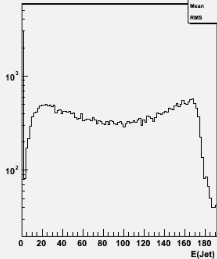
Jet energies(All jets)w102336 uue1e1e1e1_o
