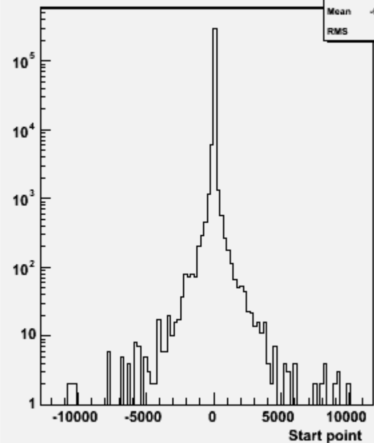
Start point Z : w102335 uue1e1e1e1_o
