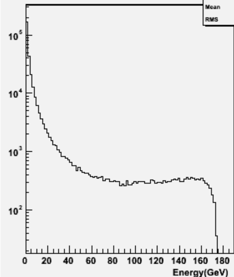
Particle Energy : w102335 uue1e1e1e1_o
