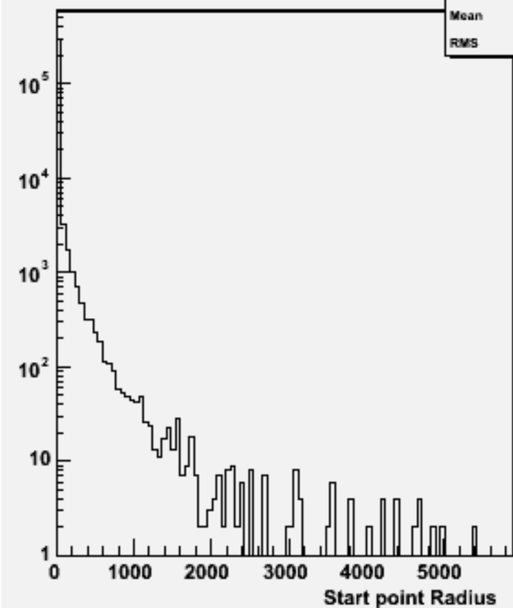
Start point R : w102335 uue1e1e1e1_o
