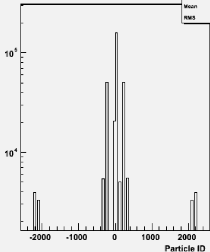
Particle ID : w102335 uue1e1e1e1_o
