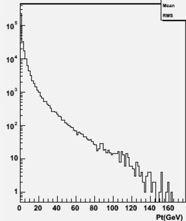
Particle Pt : w102335 uue1e1e1e1_o
