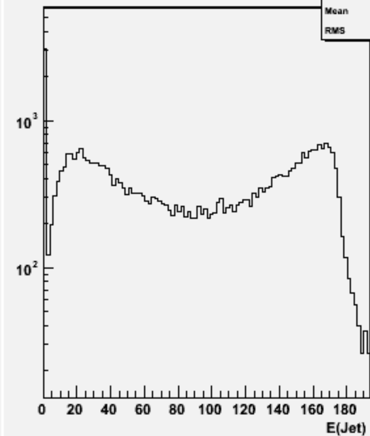
Jet energies(All jets)w102335 uue1e1e1e1_o
