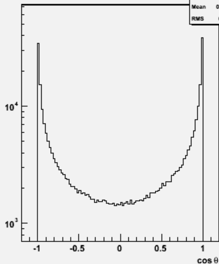
Particle \cos\theta : w102335 uue1e1e1e1_o
