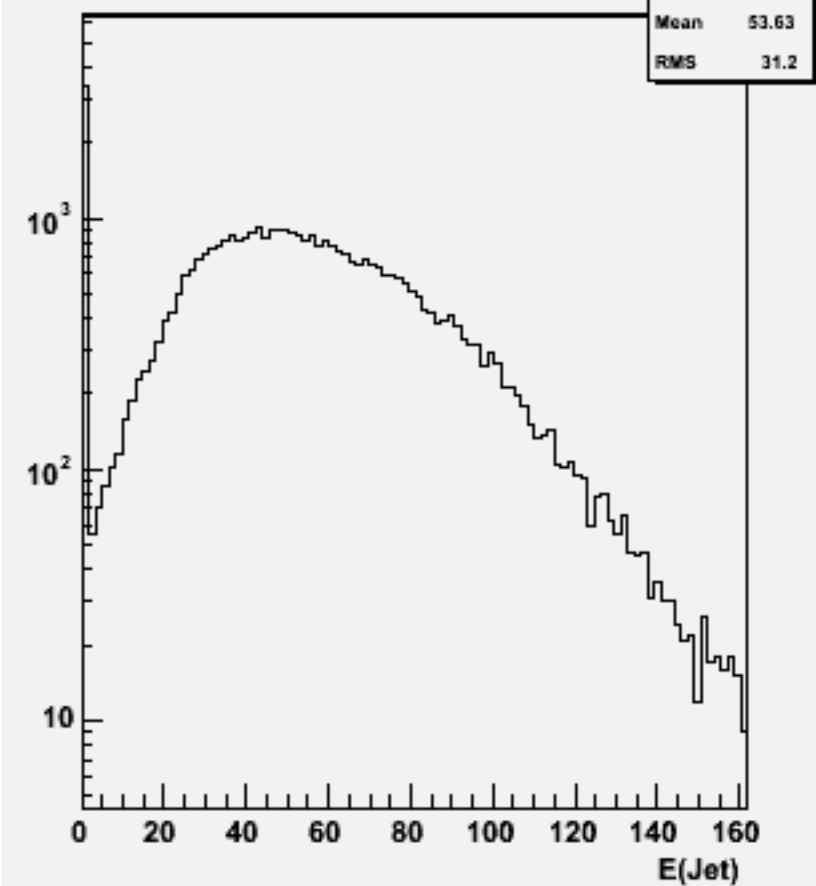
Jet energies(All jets)w102333 n3n3bbbb_o
