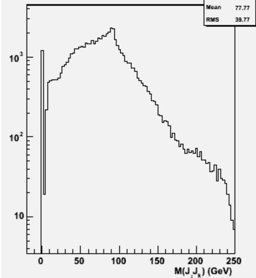
2jets mass(All comb)w102333 n3n3bbbb_o
