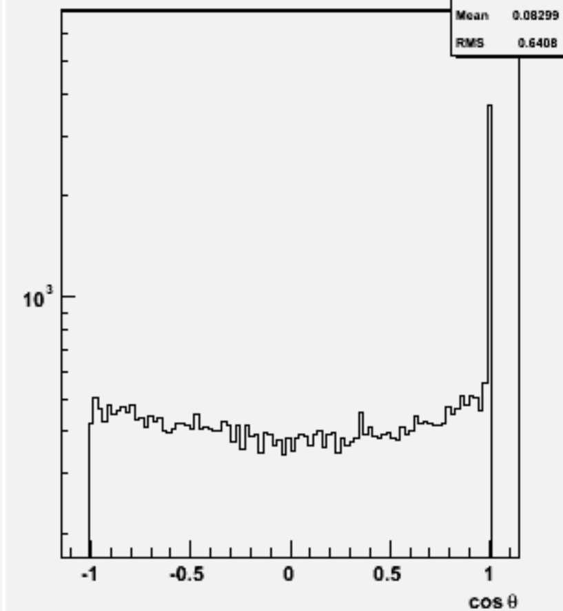
Jet cos \theta (All jets)w102333 n3n3bbbb_o
