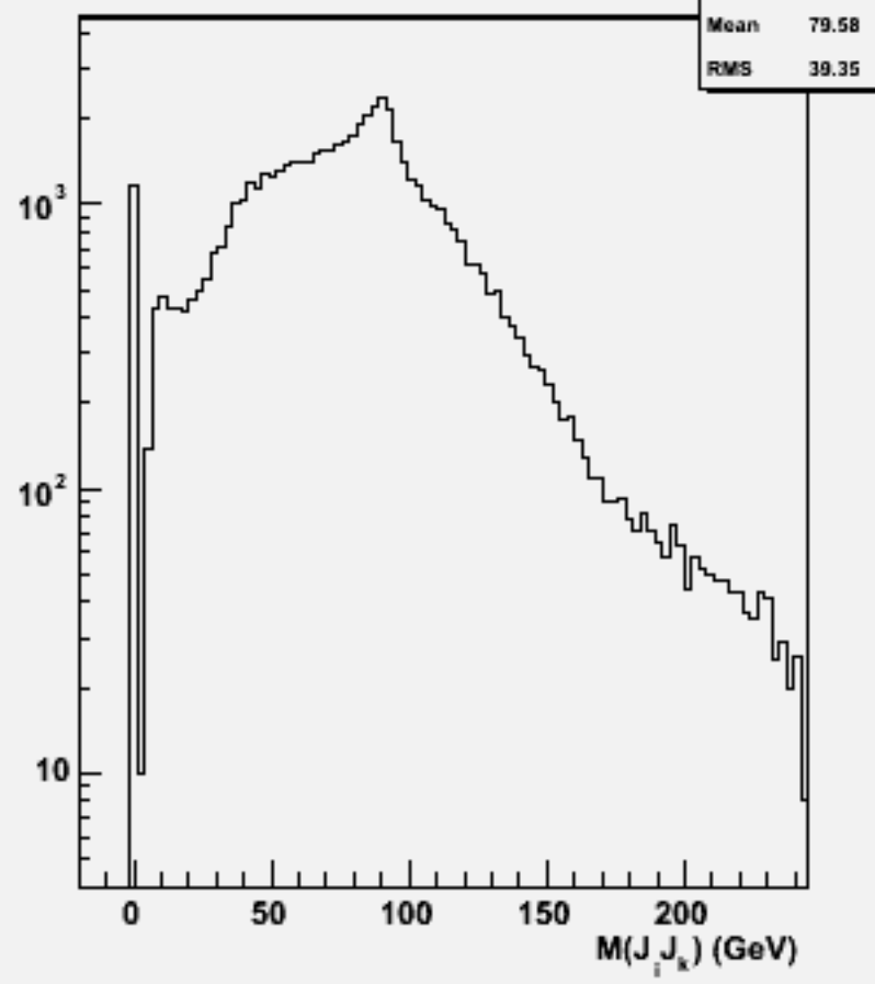
2jets mass(All comb)w102332 n3n3bbbb_o
