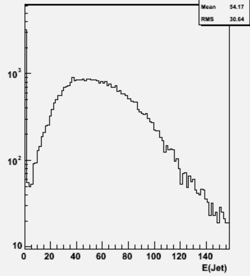
Jet energies(All jets)w102332 n3n3bbbb_o
