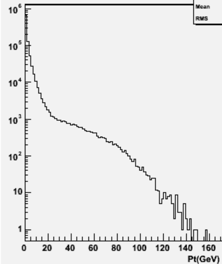
Particle Pt : w102329 n3n3ssbb_o
