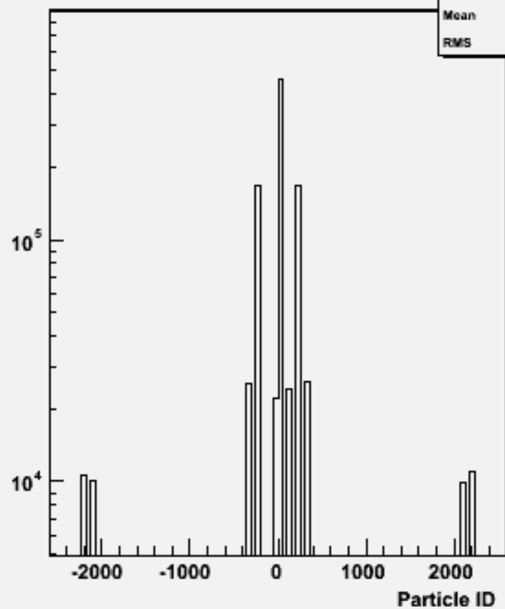
Particle ID : w102329 n3n3ssbb_o
