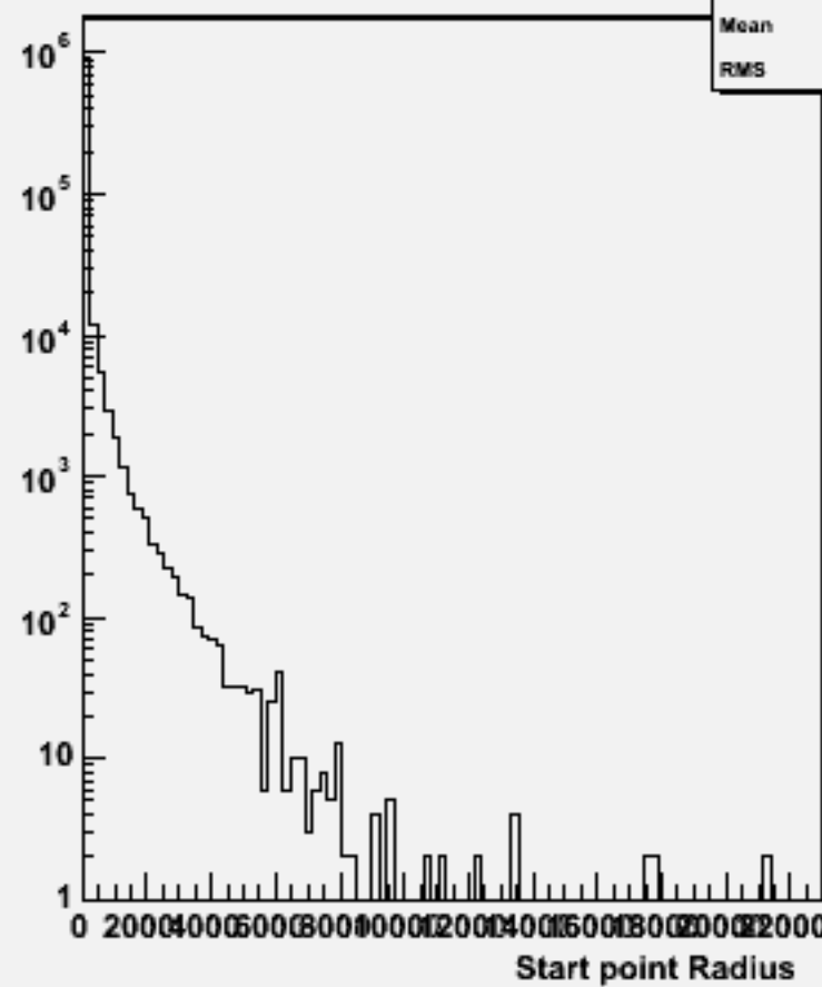
Start point R : w102329 n3n3ssbb_o
