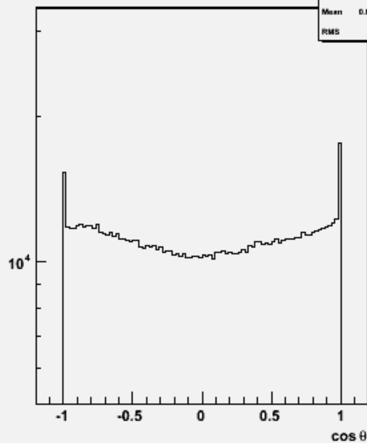
Particle cos \theta : w102329 n3n3ssbb_o
