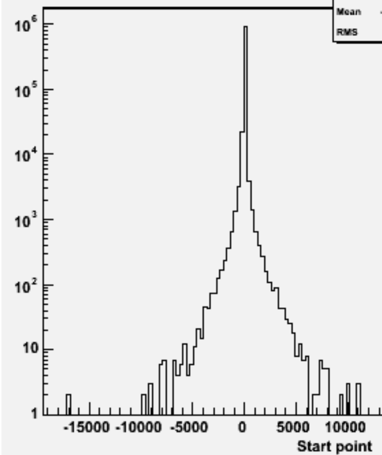
Start point Z : w102329 n3n3ssbb_o
