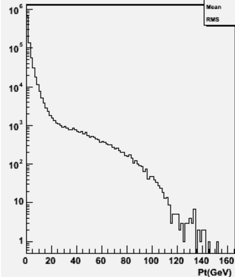
Particle Pt : w102320 n3n3ddb_o
