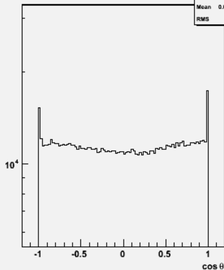
Particle cos \theta : w102320 n3n3ddb_o
