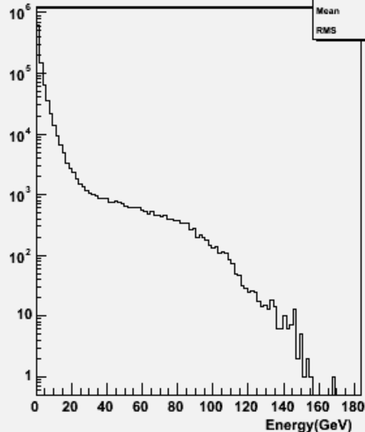
Particle Energy : w102320 n3n3ddb_o
