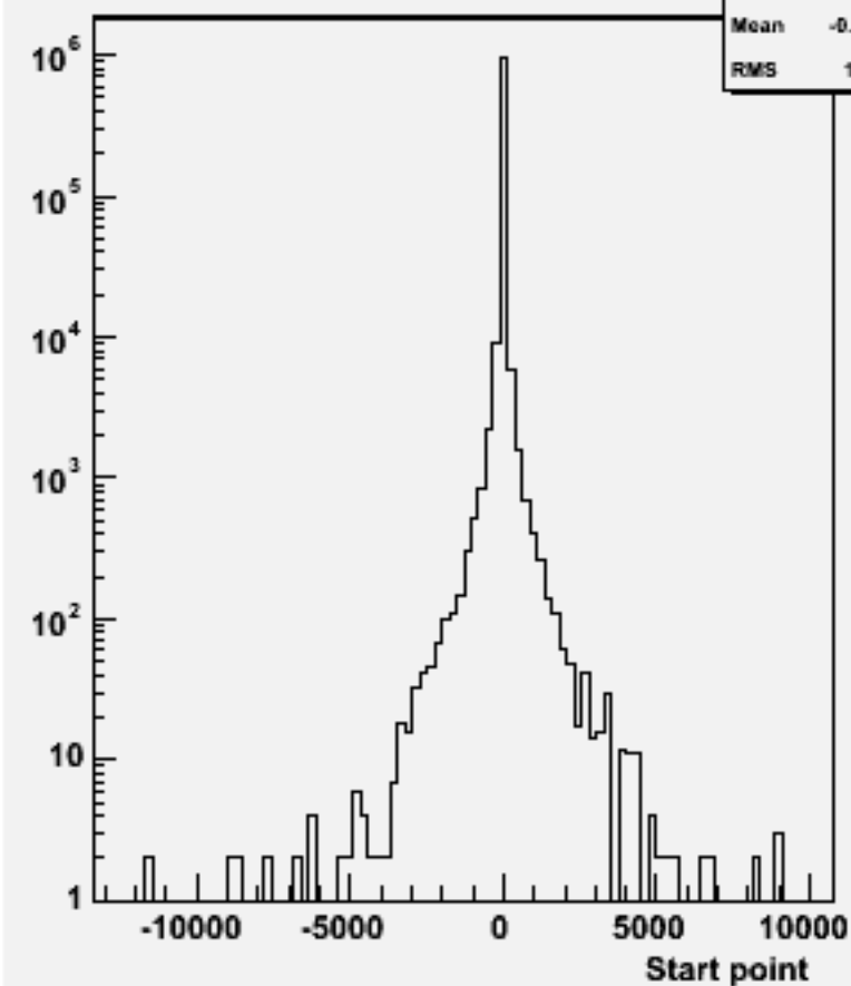
Start point Z : w102320 n3n3ddb_o
