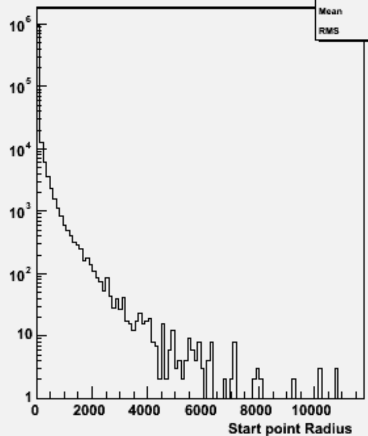
Start point R : w102320 n3n3ddb_o
