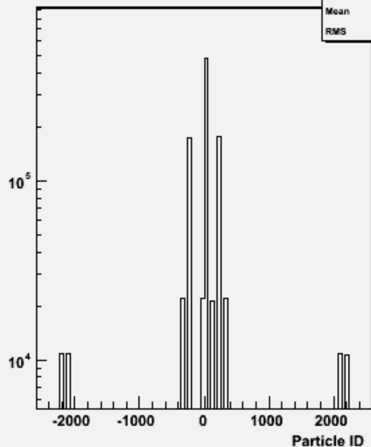
Particle ID : w102320 n3n3ddb_o
