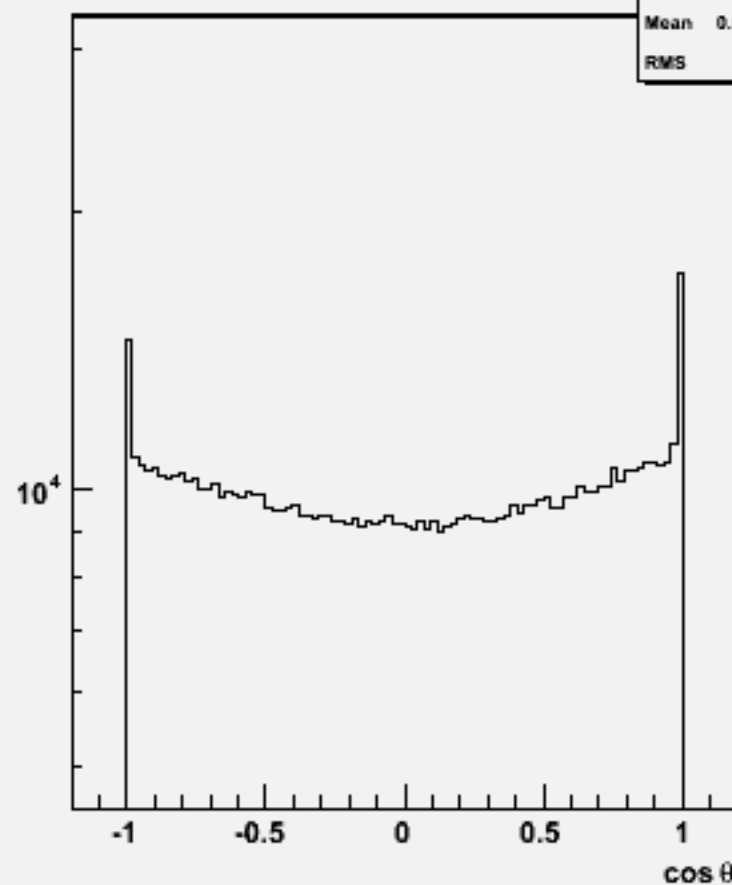
Particle cos \theta : w102313 n3n3dddd_o
