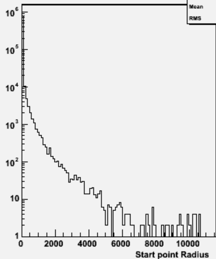
Start point R : w102313 n3n3dddd_o
