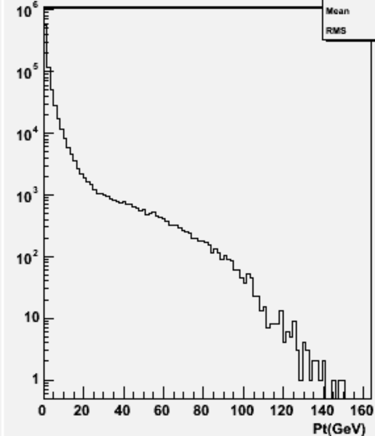
Particle Pt : w102313 n3n3dddd_o
