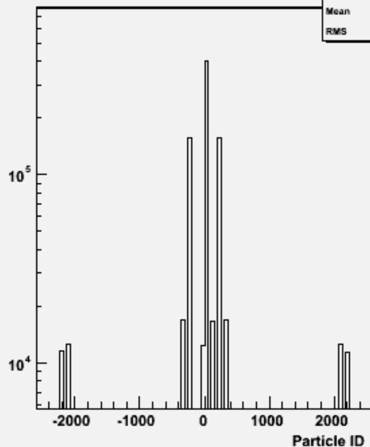
Particle ID : w102313 n3n3dddd_o
