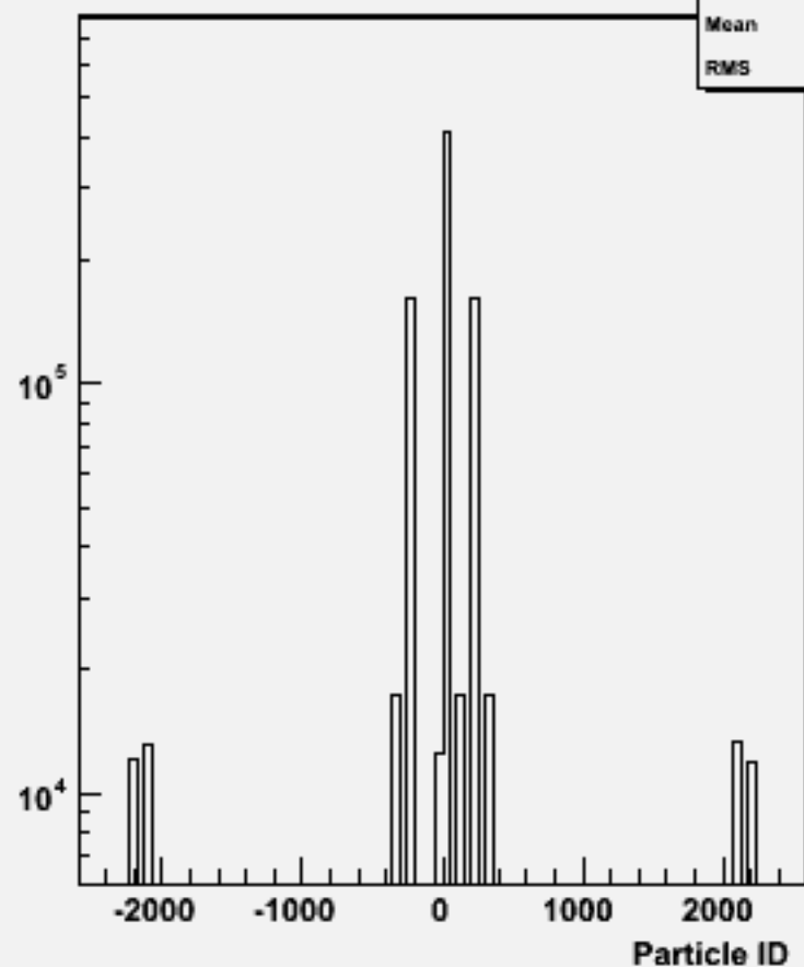
Particle ID : w102312 n3n3dddd_o
