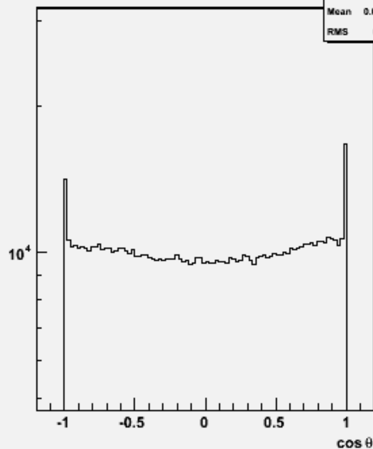
Particle cos \theta : w102312 n3n3dddd_o
