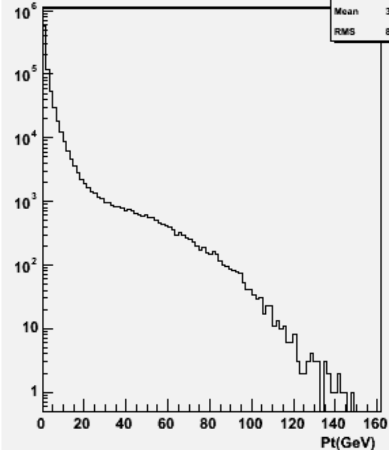
Particle Pt : w102312 n3n3dddd_o
