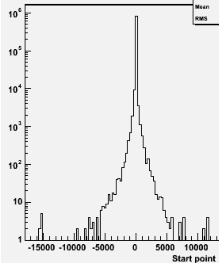
Start point Z : w102312 n3n3dddd_o
