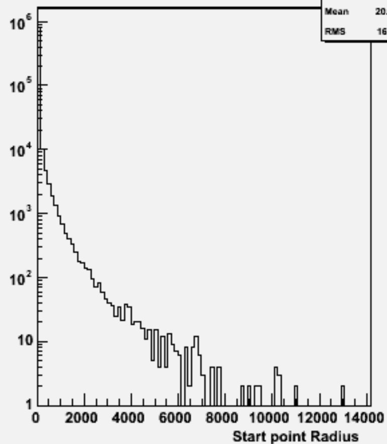
Start point R : w102312 n3n3dddd_o
