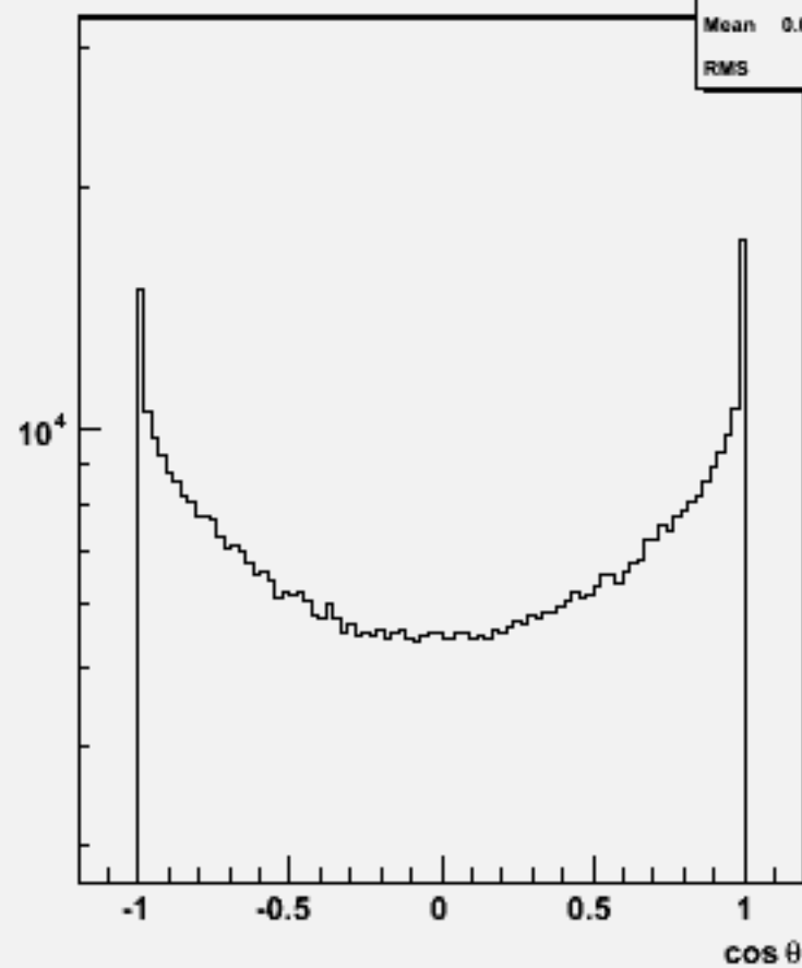
Particle cos \theta : w102309 n3n3e2e2bb_o
