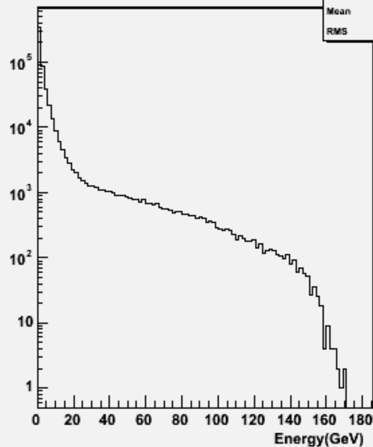
Start point R : w102309 n3n3e2e2bb_o
