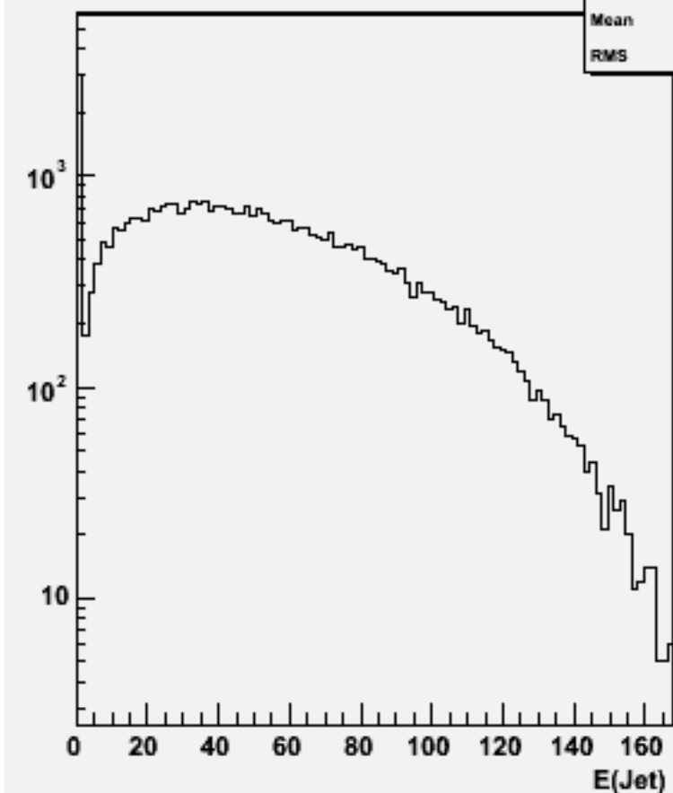
Jet energies(All jets)w102309 n3n3e2e2bb_o
