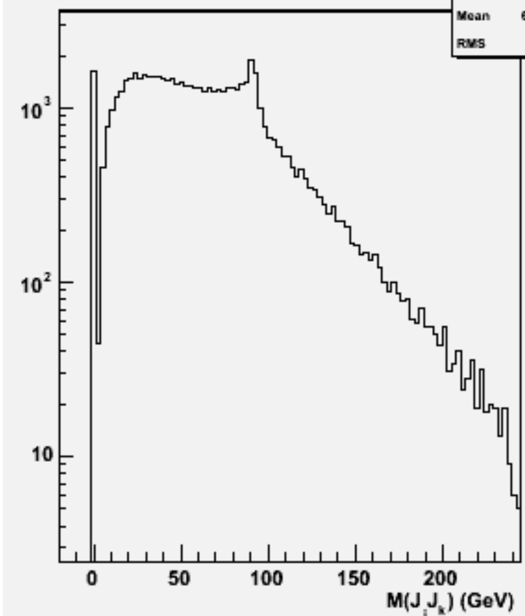
2jets mass(All comb)w102309 n3n3e2e2bb_o
