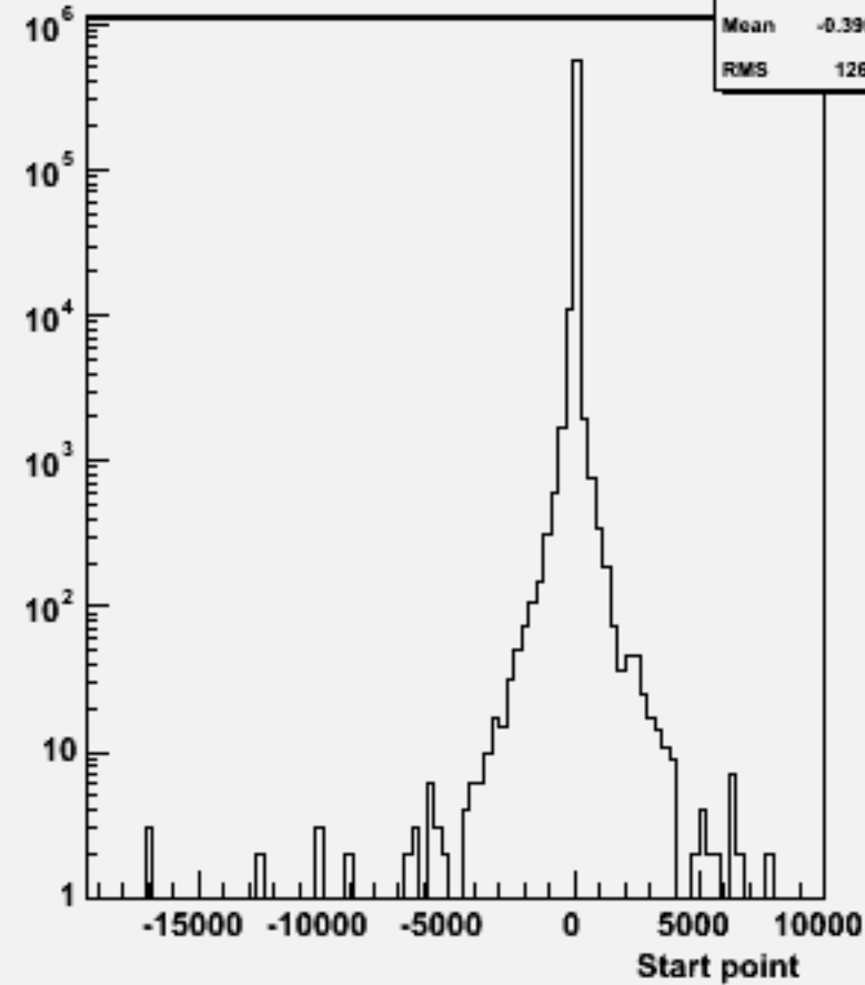
Start point Z : w102309 n3n3e2e2bb_o
