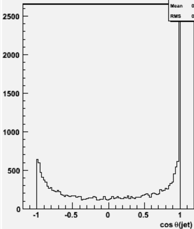
cos \theta for 2-jets :w102309 n3n3e2e2bb_o
