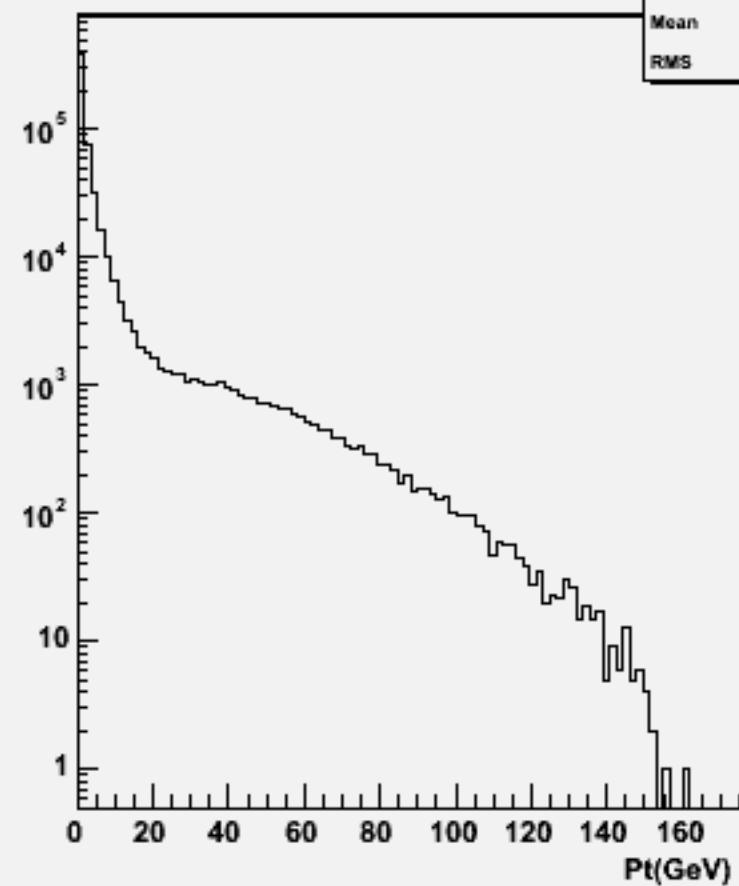
Start point Z : w102309 n3n3e2e2bb_o
