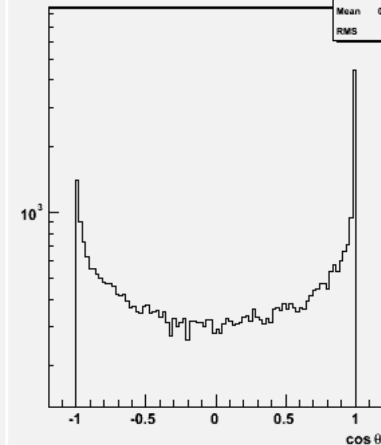
Jet cos \theta (All jets)w102309 n3n3e2e2bb_o
