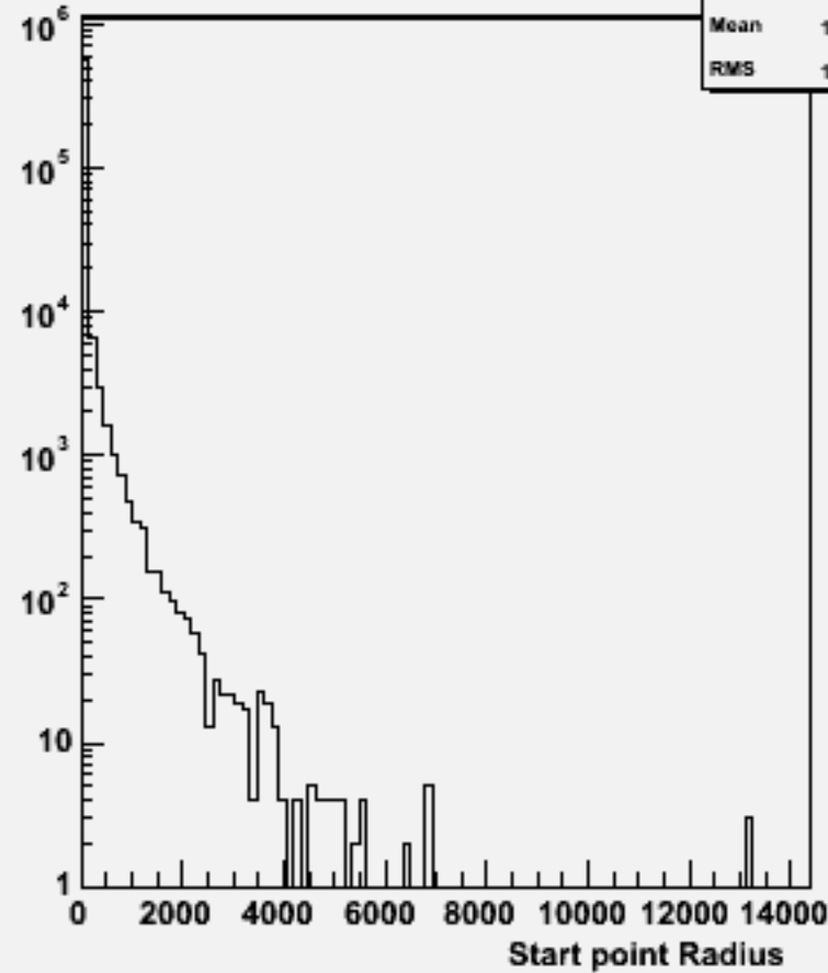
Start point R : w102309 n3n3e2e2bb_o
