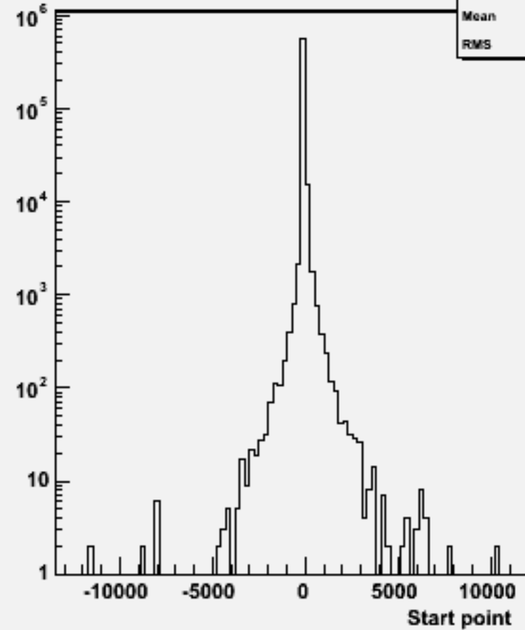
Start point Z : w102308 n3n3e2e2bb_o
