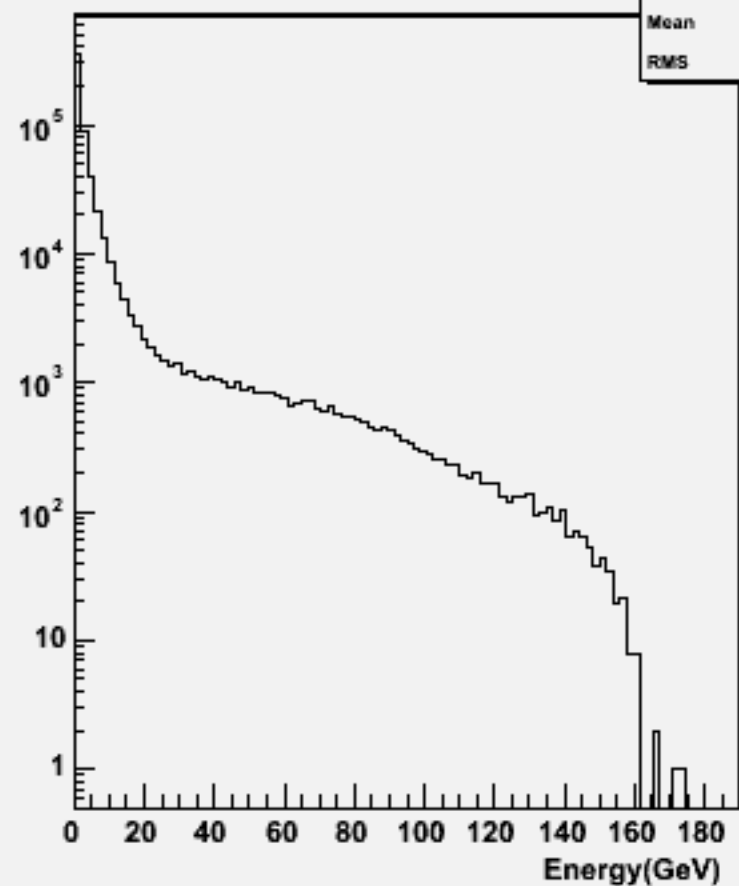
Start point R : w102308 n3n3e2e2bb_o
