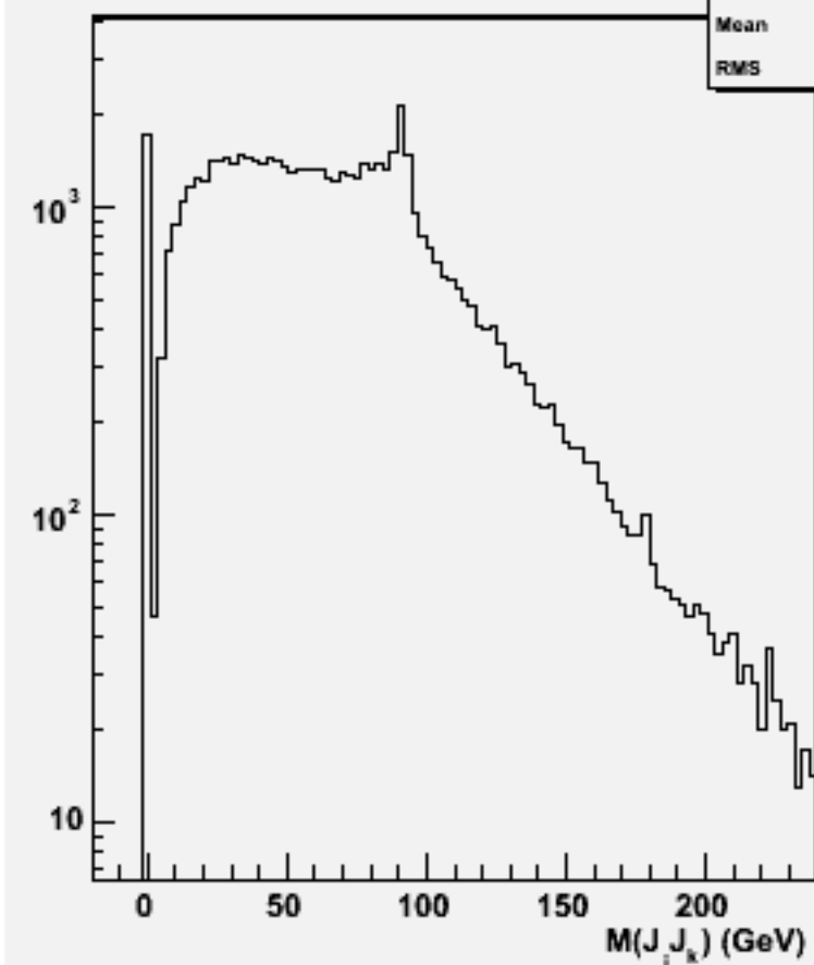
2jets mass(All comb)w102308 n3n3e2e2bb_o
