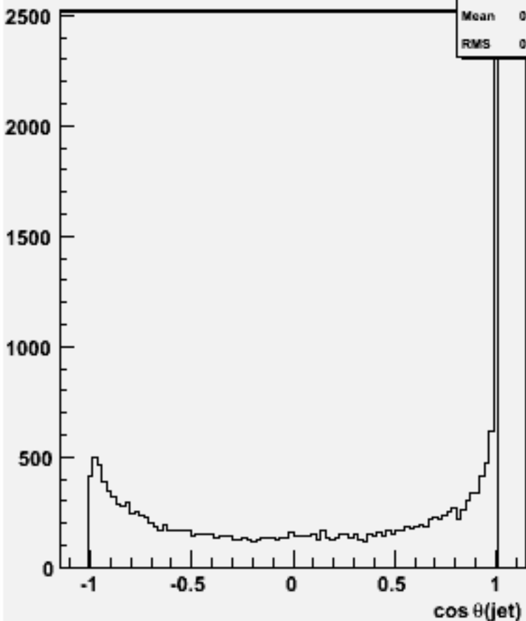
cos \theta for 2-jets :w102308 n3n3e2e2bb_o
