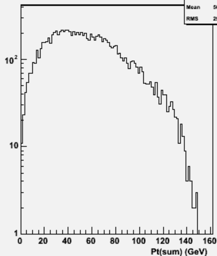
Pt Sum: w102308 n3n3e2e2bb_o
