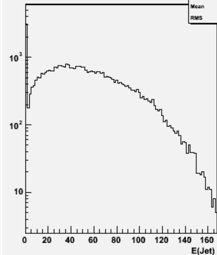
Jet energies(All jets)w102308 n3n3e2e2bb_o
