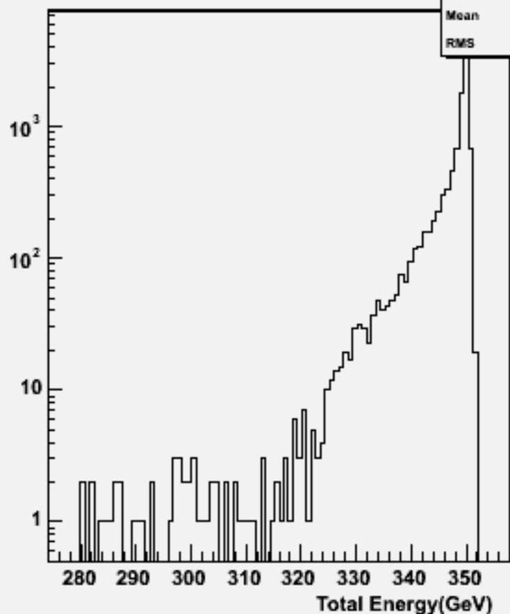
Pt Sum: w102308 n3n3e2e2bb_o
