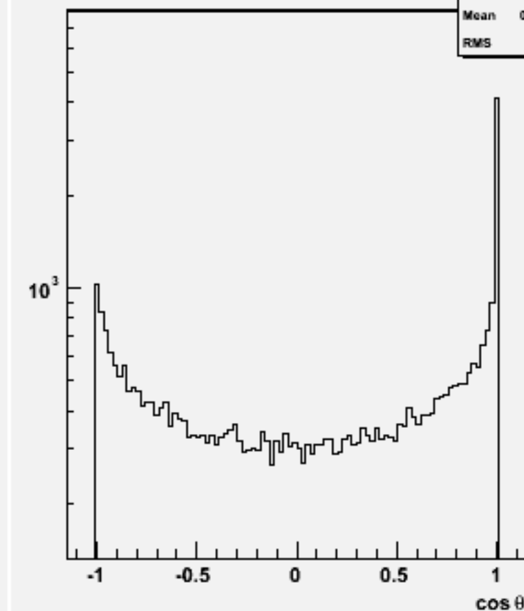
Jet cos \theta (All jets)w102308 n3n3e2e2bb_o
