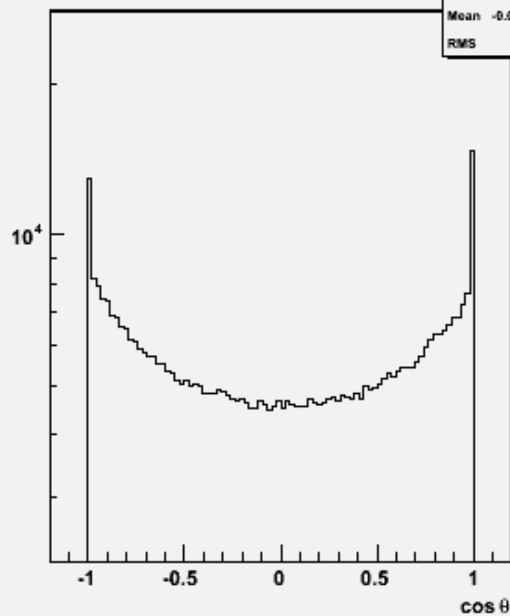
Particle cosθ : w102304 n3n3e2e2ss_o
