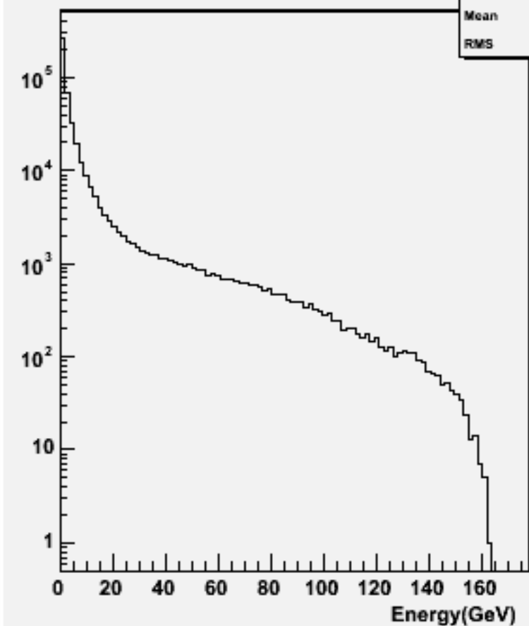
Particle Energy : w102304 n3n3e2e2ss_o
