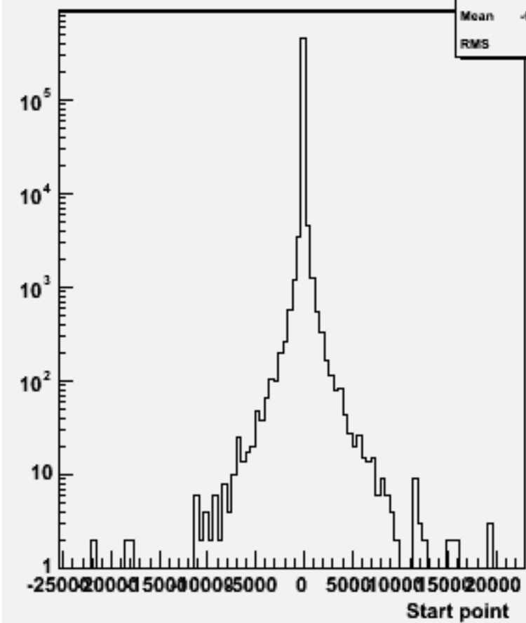
Start point Z : w102304 n3n3e2e2ss_o
