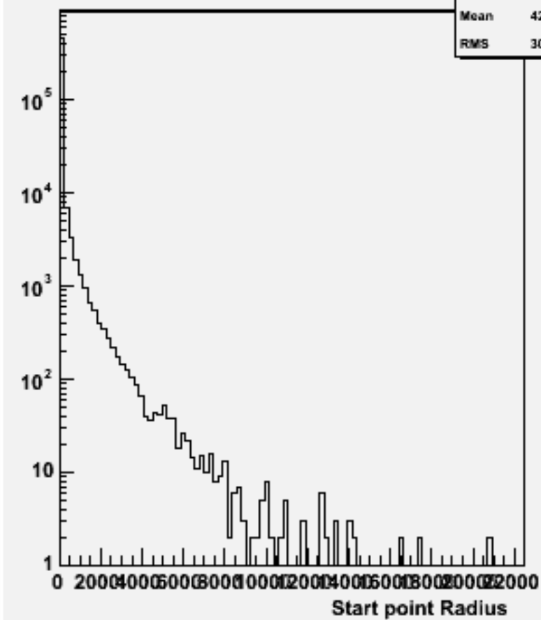
Start point R : w102304 n3n3e2e2ss_o
