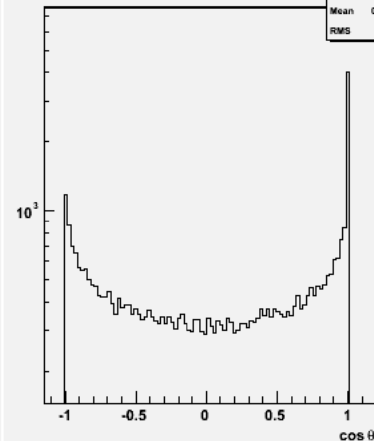
Jet cos \theta (All jets)w102304 n3n3e2e2ss_o
