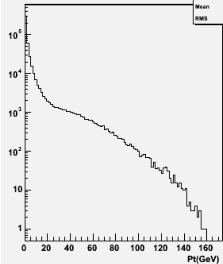
Particle Pt : w102304 n3n3e2e2ss_o
