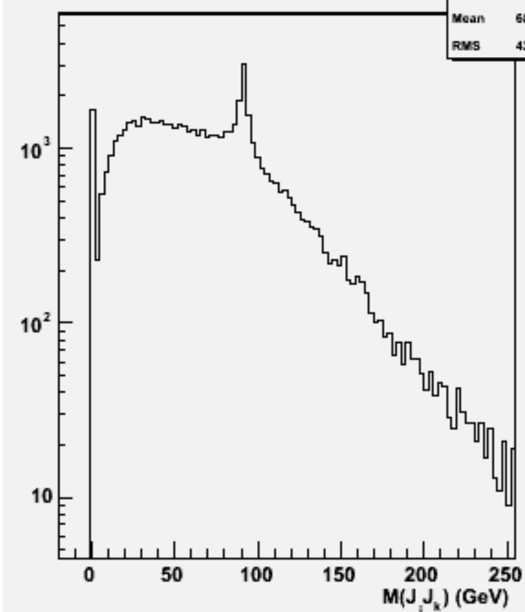
2jets mass(All comb)w102304 n3n3e2e2ss_o
