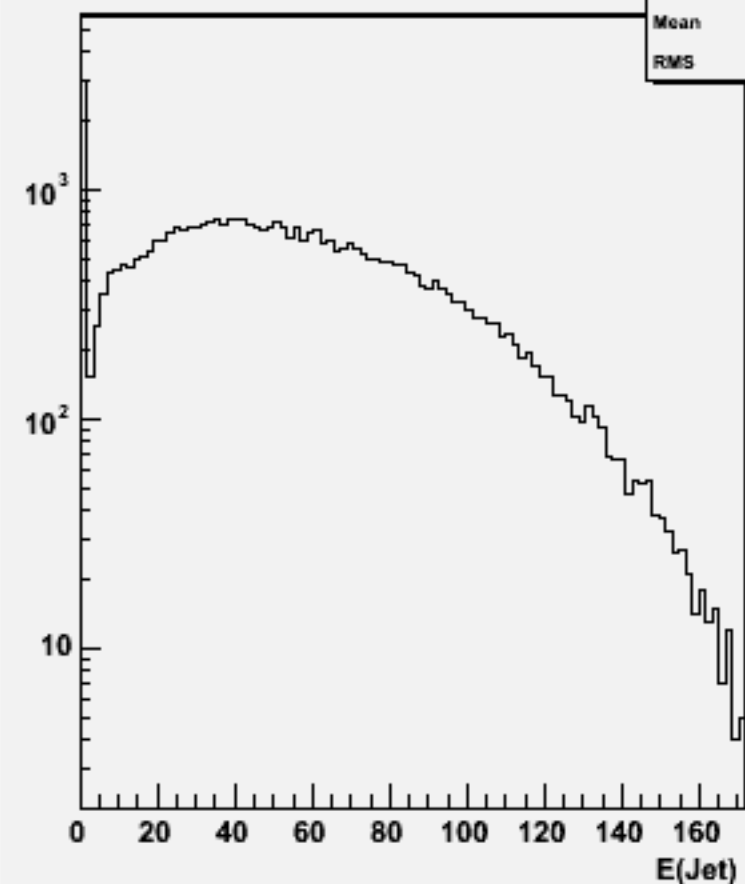
Jet energies(All jets)w102304 n3n3e2e2ss_o
