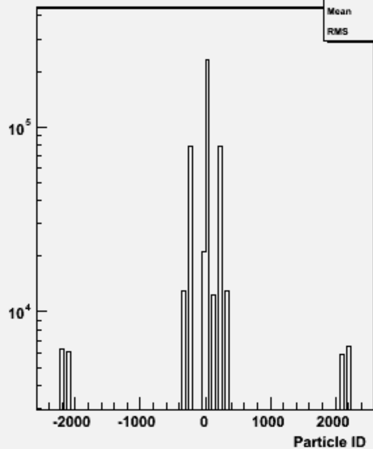
Particle ID : w102304 n3n3e2e2ss_o
