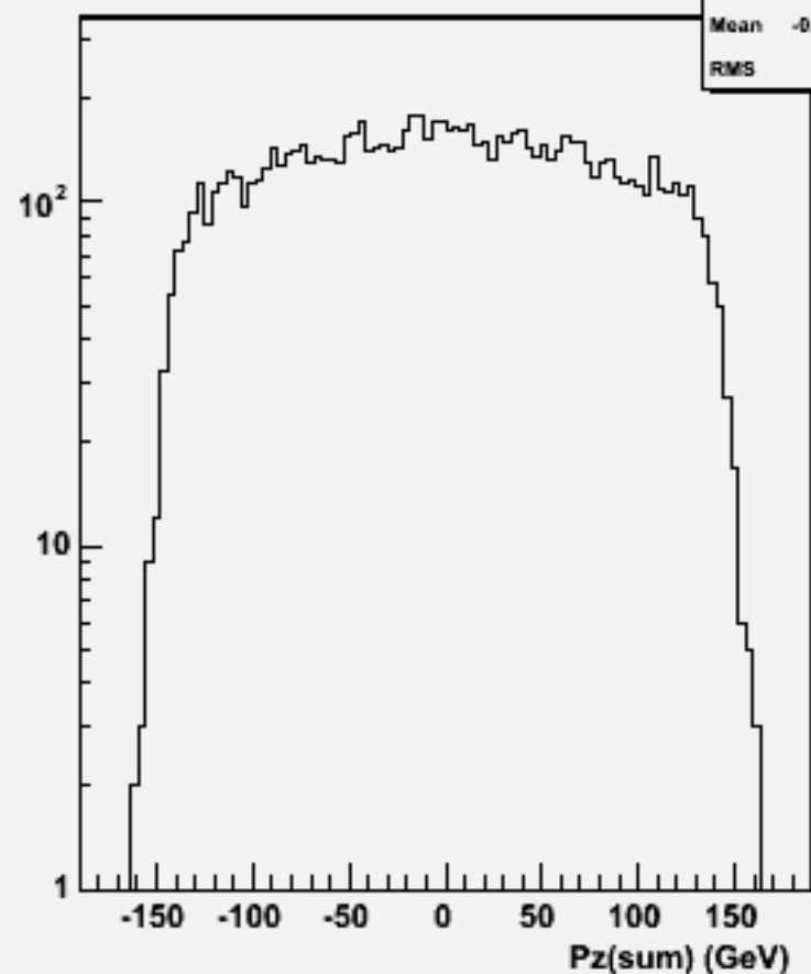
Pz Sum: w102301 n3n3e2e2dd_o
