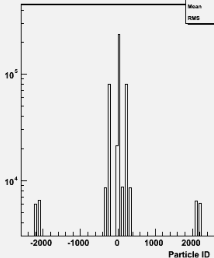
Particle ID : w102301 n3n3e2e2dd_o
