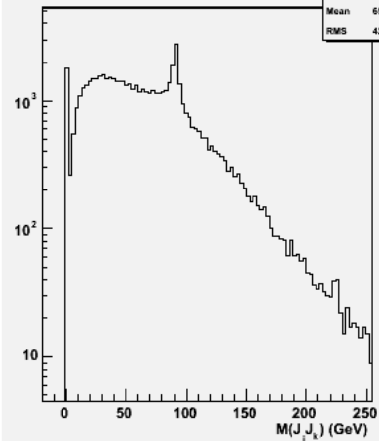
2jets mass(All comb)w102301 n3n3e2e2dd_o
