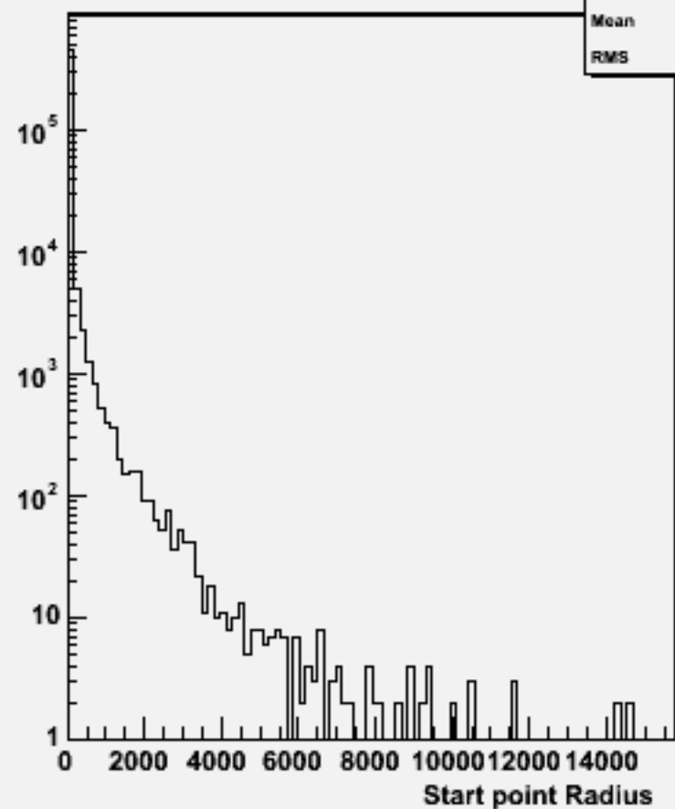
Start point R : w102301 n3n3e2e2dd_o
