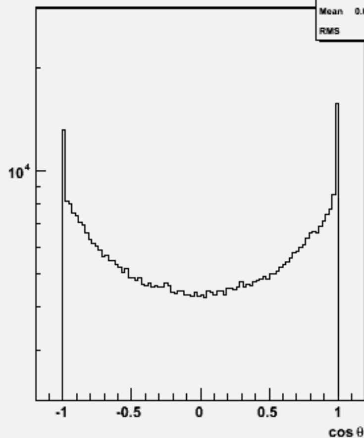
Particle cos \theta : w102301 n3n3e2e2dd_o
