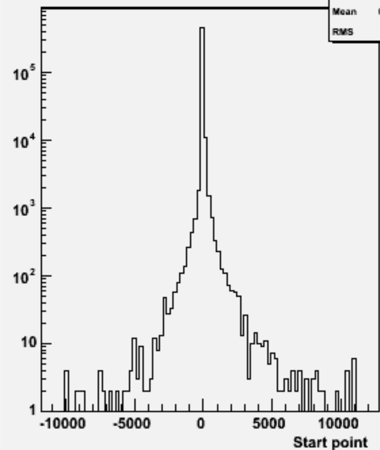
Start point Z : w102301 n3n3e2e2dd_o
