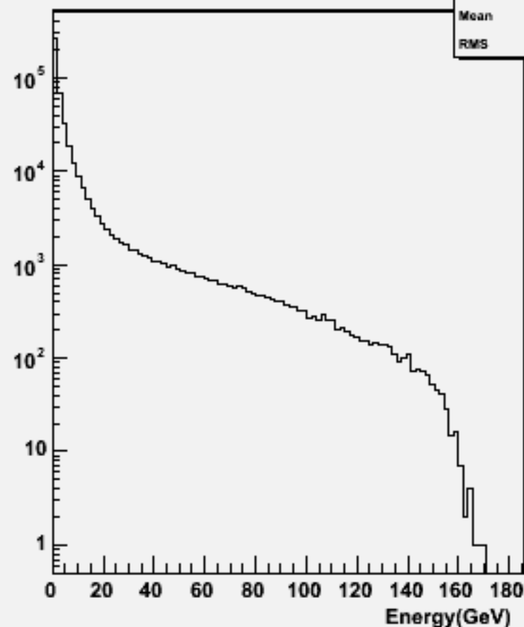
Particle Energy : w102301 n3n3e2e2dd_o
