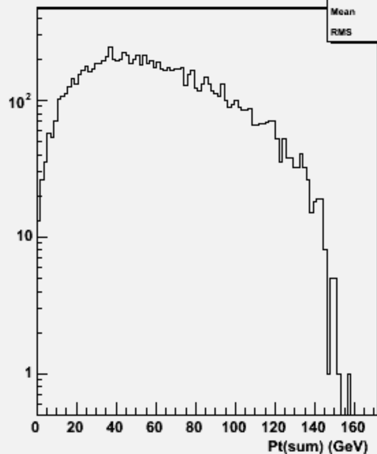
Pt Sum: w102301 n3n3e2e2dd_o
