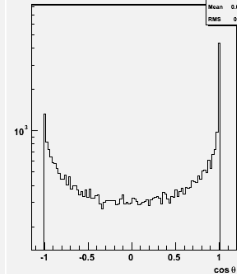
Jet cos \theta (All jets)w102301 n3n3e2e2dd_o
