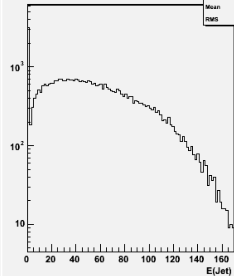
Jet energies(All jets)w102301 n3n3e2e2dd_o
