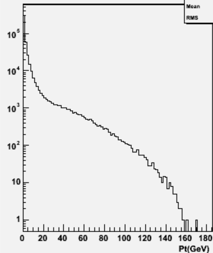
Particle Pt : w102301 n3n3e2e2dd_o
