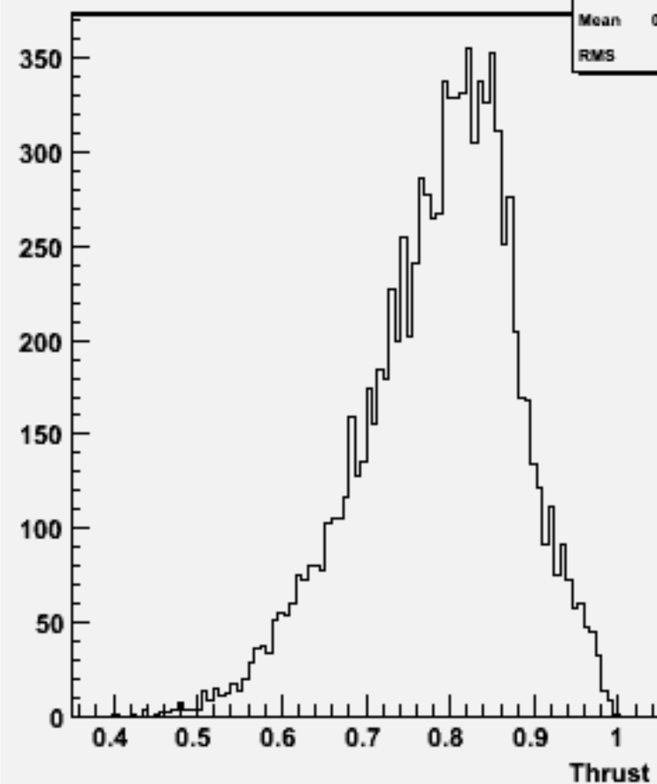
Thrust w102301 n3n3e2e2dd_o
